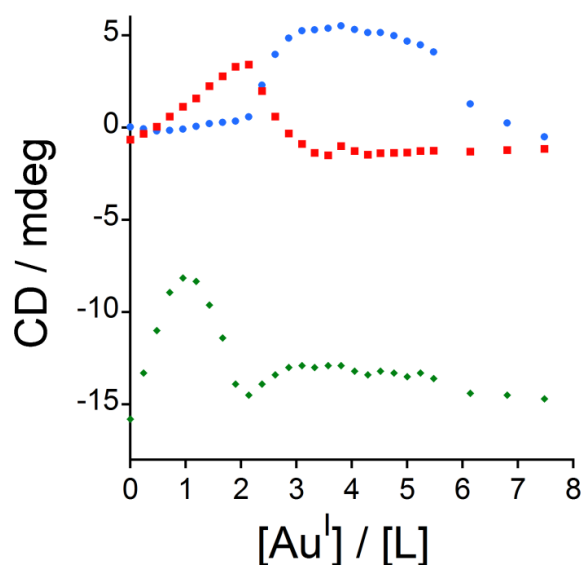
Figure 79 : Suivi du titrage par dichroïsme circulaire de CP1(CCCC) (15 μM) en fonction du nombre d'équivalents d'Au I en tampon phosphate 20 mM à pH 7,0 et 298 K. Le suivi est réalisé à 284 nm (en bleu), 243 nm (en rouge) et 208 nm (en vert). Les spectres sont corrigés de la dilution, trajet optique : 0,4 cm.
