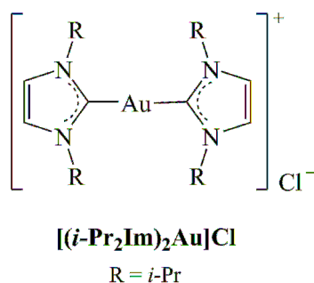
Figure 12 : Exemple de complexe or(I)-carbène.
