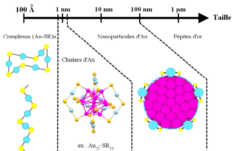
Figure 4 : Echelle de taille des complexes d'or-thiolates 10 sous forme cyclique (haut) et linéaire (bas), des clusters d'or 23 et des nanoparticules d'or 21 . Sur les schémas, l' Au^I , l' Au^0 et les ligands thiolates sont représentés respectivement par des sphères bleues, roses et jaunes. Les substituants R sur les thiolates ont été retirés pour plus de clarté.
