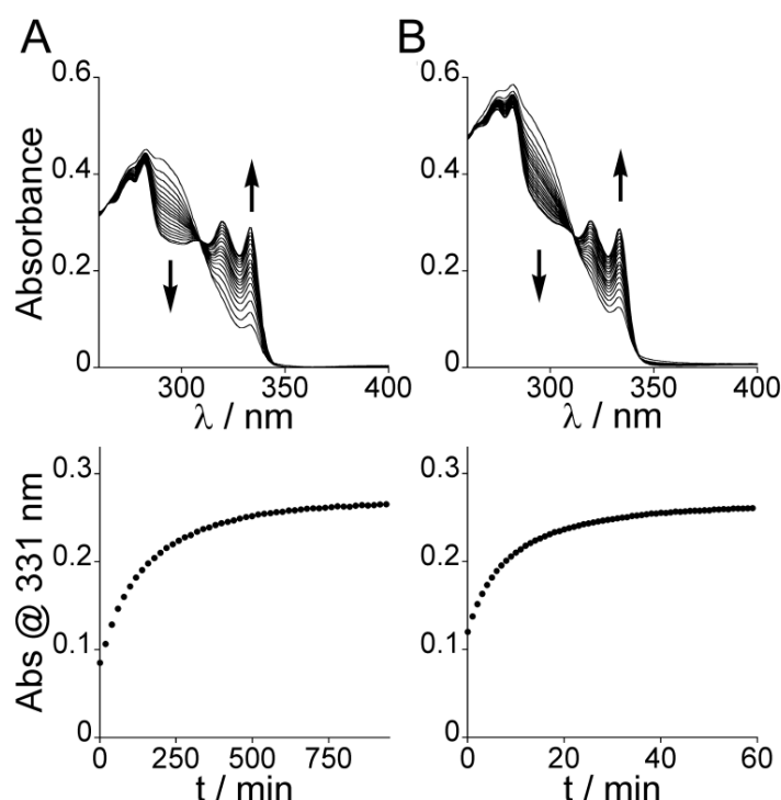
Figure 61 : Suivi au cours du temps de la réaction entre Zn II -L ZR (20 μM) et Au III Terpy (55 μM en (a) et 70 μM en (b)) en présence de glutathion (1 mM en (a)) ou de β-mercaptoéthanol (1 mM en (b)) par UV-Vis en tampon phosphate 20 mM à pH 7,0 et 298 K. En haut, évolution des spectres d'absorbance et en bas, évolution de l'absorbance à 331 nm, les premiers spectres d'absorbance sont enregistrés à 7 s pour (a) et 3 s pour (b).
