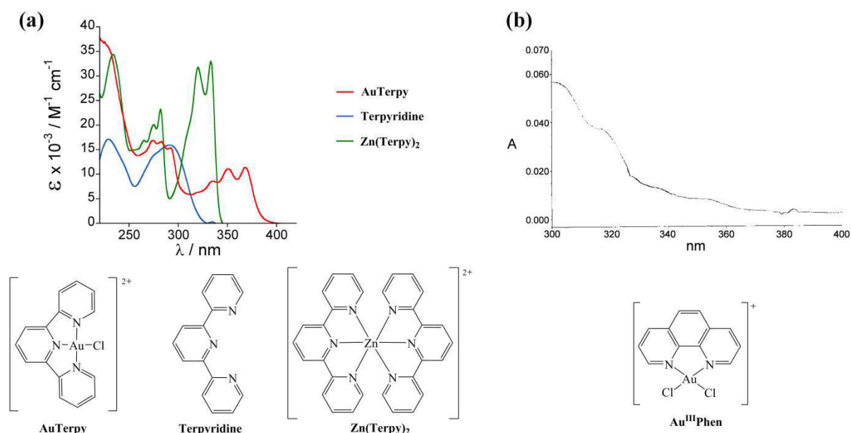
Figure 46 : En haut, spectres d'absorbance (a) d' Au^{III} Terpy (en rouge), de la terpyridine (en bleu) et de Zn^{II}(\text{Terpy})_2 (en vert) en tampon phosphate (20 mM) à pH 7,0 et 298 K et (b) d' Au^{III} Phen (7,5 \mu\text{M} ) en tampon physiologique (tampon phosphate 50 mM, NaCl 4 mM à pH 7,4), d'après Messori et al. 4 En bas, formules chimiques de ces composés.
