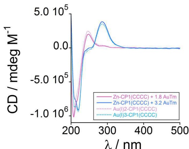
Figure 96 : Spectres CD obtenus après réaction de \text{Zn}^{\text{II}}\text{-CP1(CCCC)} ( \sim 20 \mu\text{M} ) avec l' \text{Au}^{\text{I}}\text{Tm} (1,8 éq. en rose et 3,2 éq. en bleu en traits pleins). Ces spectres sont superposés à ceux des complexes \text{Au}^{\text{I}}_n\text{-CP1} ( n = 2 en rose et n = 3 en bleu) caractérisés dans la partie précédente (en pointillés). Les réactions ont été réalisées en tampon phosphate 20 mM à pH 7,0 et 298 K. Les spectres ont été corrigés de la dilution ; trajet optique = 0,4 cm.
