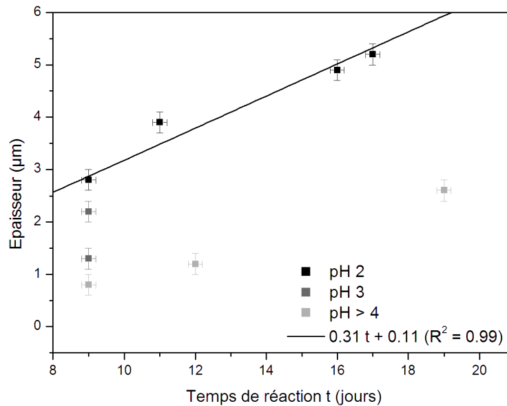
FIGURE III.9: Évolution de l'épaisseur des revêtements de boehmite en fonction du temps de réaction et du pH des expériences MPA. On remarque que plus le temps de réaction est grand, plus l'épaisseur des revêtements est importante. De plus, l'épaisseur est d'autant plus grande que le pH est faible.
