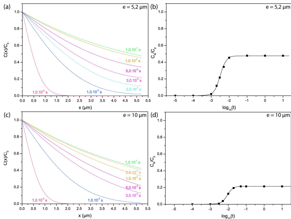
FIGURE IV.9: Influence de la vitesse de dissolution. On étudie ici l'évolution de la concentration en H^+ dans deux revêtements d'épaisseur égale à 5,2 \mu\text{m} et 10 \mu\text{m} . La porosité est fixée à 22%. (a), (c) Profils de concentrations : le rapport C(x)/C_0 est représenté en fonction de x pour différents temps t . (b), (d) Évolution du rapport C_N/C_0 en fonction de \log(t) .
