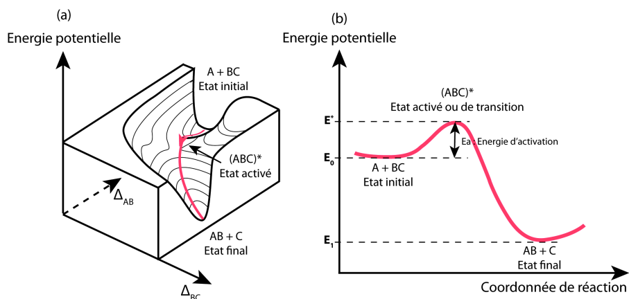
FIGURE VI.4: (a) Diagramme d'équipotentielle. \Delta_{AB} et \Delta_{BC} représentent les distances entre les atomes A, B et C. Le chemin réactionnel du processus élémentaire VI.1 est représenté en rouge. Celui-ci est le chemin le moins coûteux en énergie. (b) Représentation de l'évolution de l'énergie potentielle au cours du processus élémentaire (VI.1).
