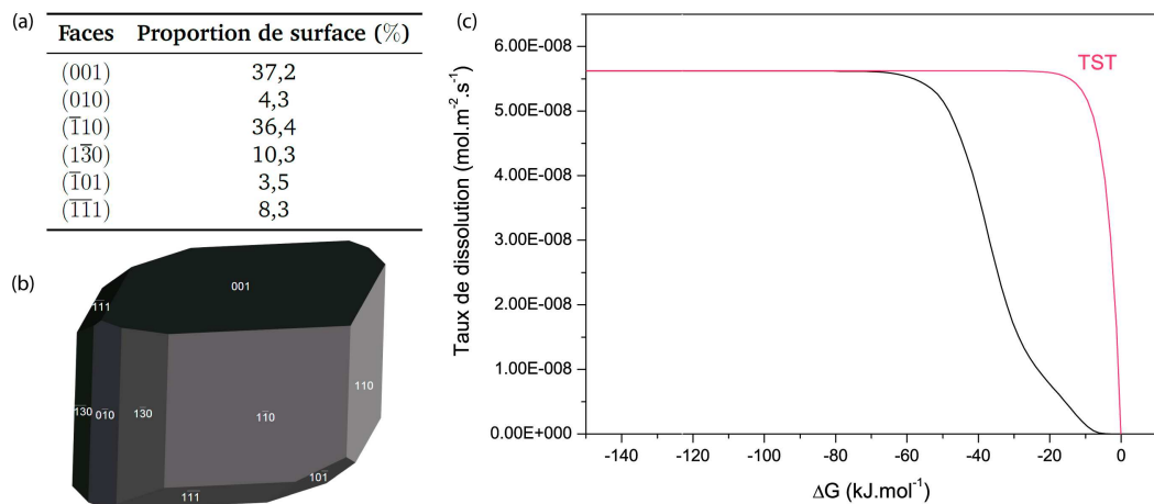
FIGURE VIII.6: Morphologie moyenne possible pour représenter la poudre de feldspath potassique utilisée. (a) Proportion de surface de chaque face. (b) Aspect possible de l'habitus d'un grain. (c) Relation r - \Delta_r G correspondant à l'habitus moyen choisi pour représenter la poudre. A -52 \text{ kJ.mol}^{-1} , le taux de dissolution de cet habitus est de 5.410^{-8} \text{ mol.m}^{-2}.\text{s}^{-1} . Cela correspond au taux de dissolution mesuré sur la poudre.
