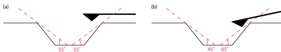
FIGURE C.1: Schémas illustrant l'angle limite mesurable en AFM lorsque (a) l'inclinaison de la pointe est nulle et (b) la pointe est inclinée de 10^\circ par rapport à l'horizontale.
