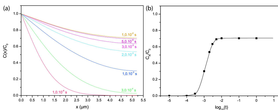
FIGURE IV.7: Résultats du modèle dans le cas d'un revêtement de 5,2 \mu\text{m} d'épaisseur et de porosité constante égale à 22% recouvrant l'orthose dans des conditions chimiques comparables à celles de Soultz-sous-Forêts (i.e. pH 5,3 à 180^{\circ}\text{C} ). (a) Profils de concentrations : le rapport C(x)/C_0 est représenté en fonction de x pour différents temps t . (b) Évolution du rapport C_N/C_0 en fonction de \log(t) . C_N représente la concentration en \text{H}^+ au sein de la maille dernière maille N du revêtement.
