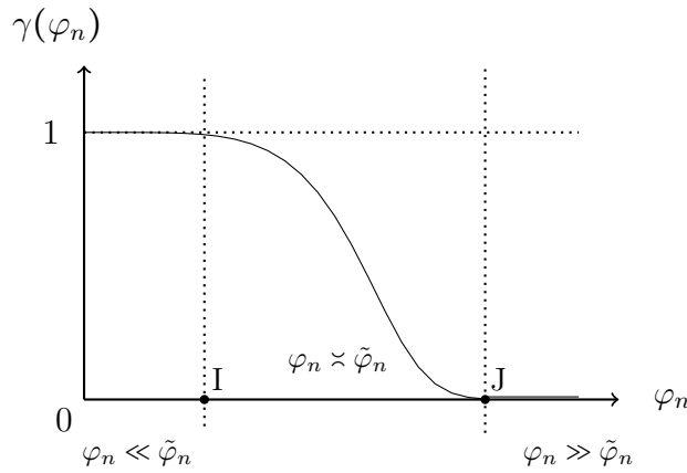
Figure 1.1 – Variation de l'erreur totale \gamma en fonction du rayon \varphi_n , qui caractérise l'écart entre l'hypothèse nulle et l'hypothèse alternative.
