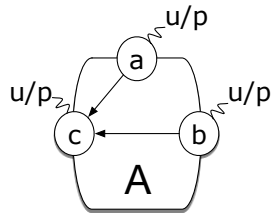
(d) Context-insensitive abstraction of the flow of information.
