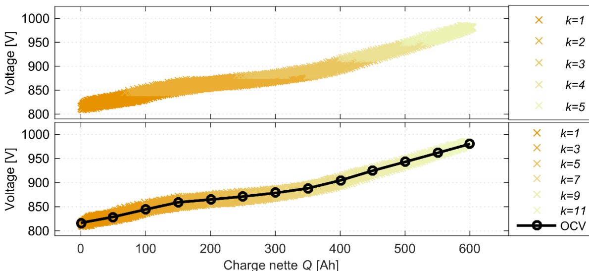
Figure 55. Échantillons de la tension sur la charge nette de la batterie dans le système industriel. En haut : échantillons bruts avec un rendement de 100 %. En bas : échantillons répartis par plage de charge nette avec la courbe linéaire par morceaux issue de la régression.
