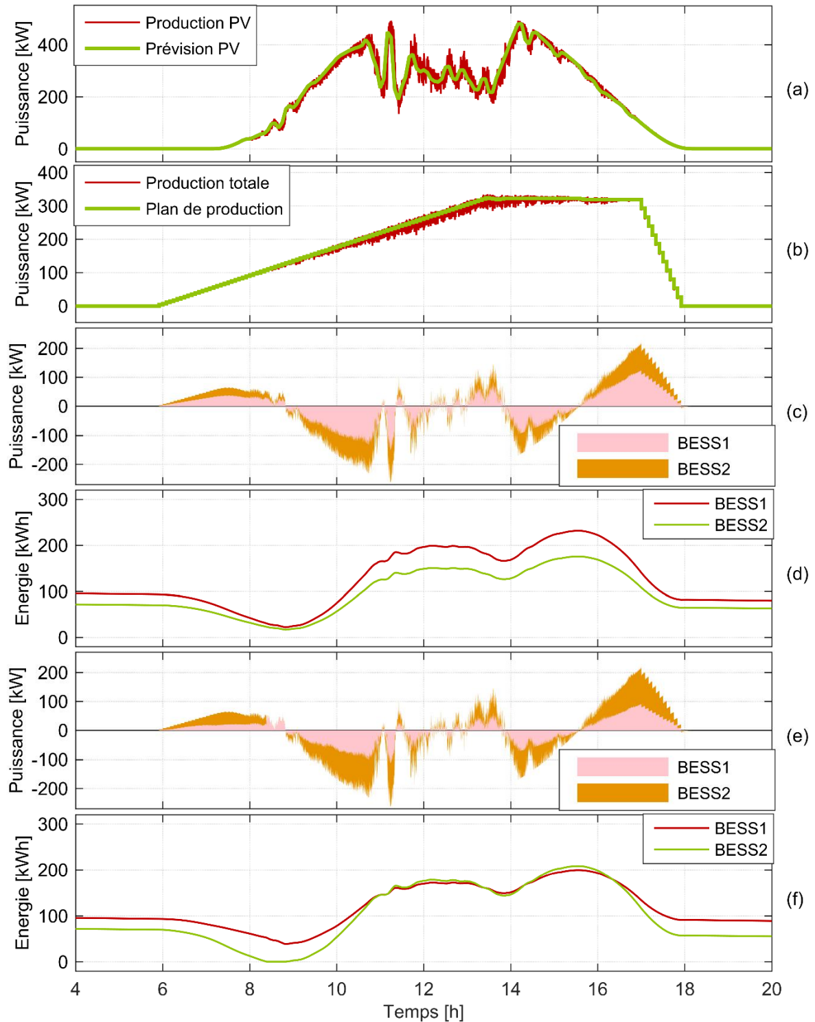
Figure 93. Fonctionnement de la centrale selon la répartition de la puissance. (a) Prévision photovoltaïque et capacité disponible. (b) Plan de production et production réalisée. Répartition selon les puissances disponibles : (c) puissance des systèmes de stockage, (d) énergie stockée. Répartition optimisée : (e) puissance des systèmes de stockage, (f) énergie stockée.
