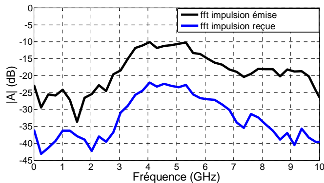
Figure 4.21: Spectres des impulsions émise et reçue (antenne PulsON, d_{ug} = 0\text{cm} ).
