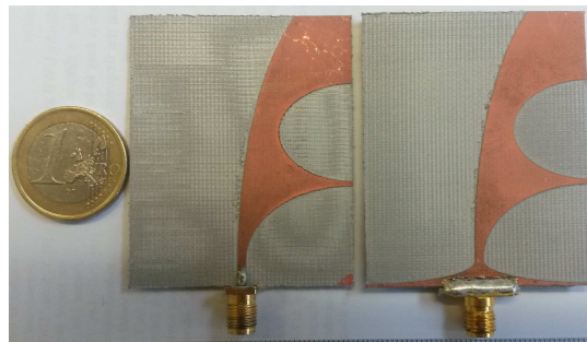
Figure 2.40: Prototypes réalisés de l'AVA-FLE.
