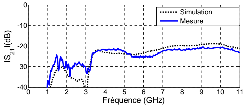
Figure 2.45 : Amplitude de la fonction de transfert du système.
