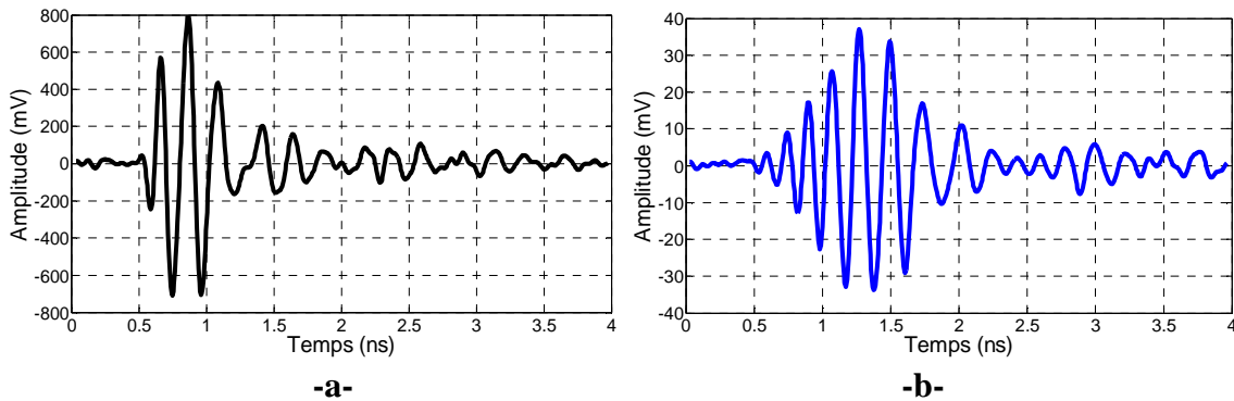
Figure 4.20: Impulsions : a) émise (générateur) et b) reçue (antenne PulsON, d_{ug} = 0\text{ cm} , d_{ag} = 1\text{ m} ).
