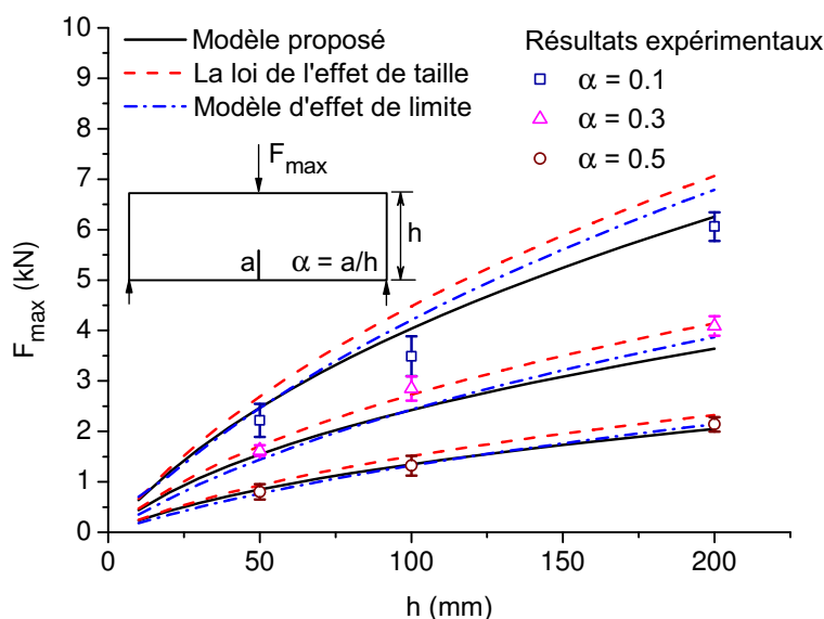
Figure 1: Prédications du modèle de la charge de rupture F_{max} par rapport à la hauteur de la poutre h en comparaison avec les prédictions de la loi de l'effet de la taille, les prévisions du modèle d'effet de bord, et les résultats des essais des échantillons de pâte de ciment durcie.
