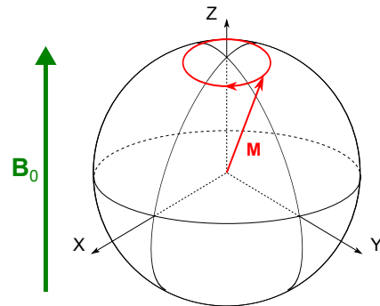
Fig. 2.2. Schéma de précession libre de l'aimantation macroscopique en absence de relaxation.
