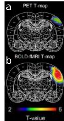
Fig. 1.11. Comparaison du changement de perfusion moyen, suite à une excitation électrique des vibrisses de rat, entre une acquisition a. PET [^{15}O] - H_2O et une acquisition b. BOLD, adapté de WEHRL et al. (2014)
