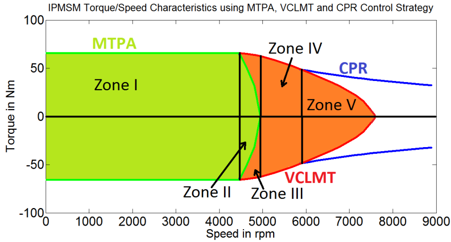
Figure II.7 : Caractéristiques Couple/Vitesse de l'IPMSM proposé
