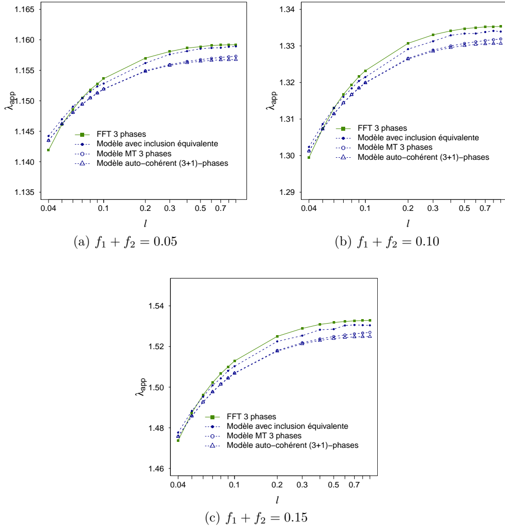
Figure 5.5 – Comparaison (en échelle logarithmique) des modèles auto-cohérent (3+1)-phases, de Mori-Tanaka (3 phases), avec inclusion équivalente et la FFT (en W.K^{-1}.m^{-1} )
