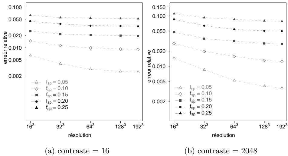
Figure 1.15 – Erreur relative du tenseur d'élasticité selon la fraction volumique de la sphère f_{sp} (contraste de 16 et 2048, résolution de 16^3 à 192^3 )
