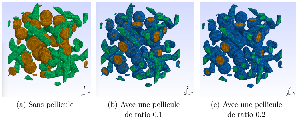
Figure 2.16 – Inclusions non pelliculées et pelliculées
