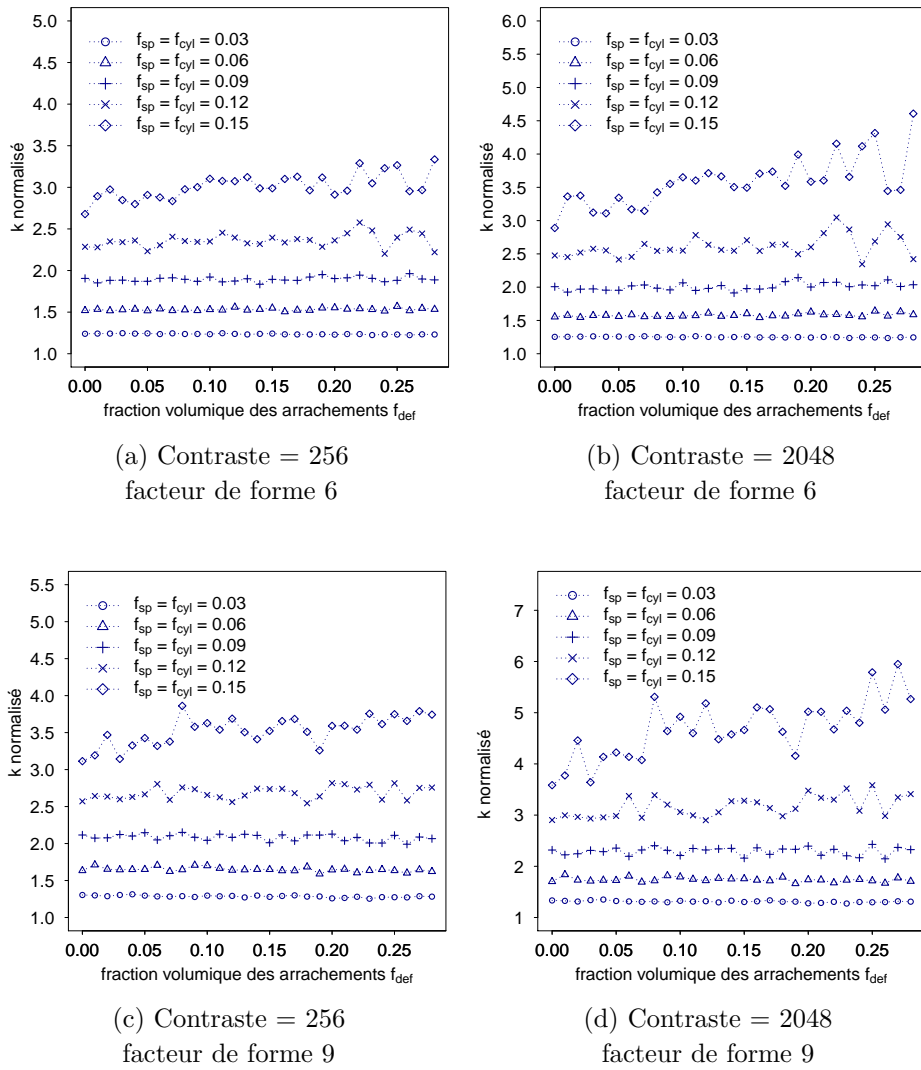
Figure 4.19 – Évolution du coefficient de compressibilité homogénéisé k d'un matériau composite à inclusions cylindriques (de facteur de forme 6 et 9) et sphériques en fonction de la fraction volumique des arrachements ( f_{cyl} = f_{sp} = 0.03, 0.06, 0.09, 0.12, 0.15 , n_{cyl} = n_{sp} = 20 , contraste = 256, 2048)
