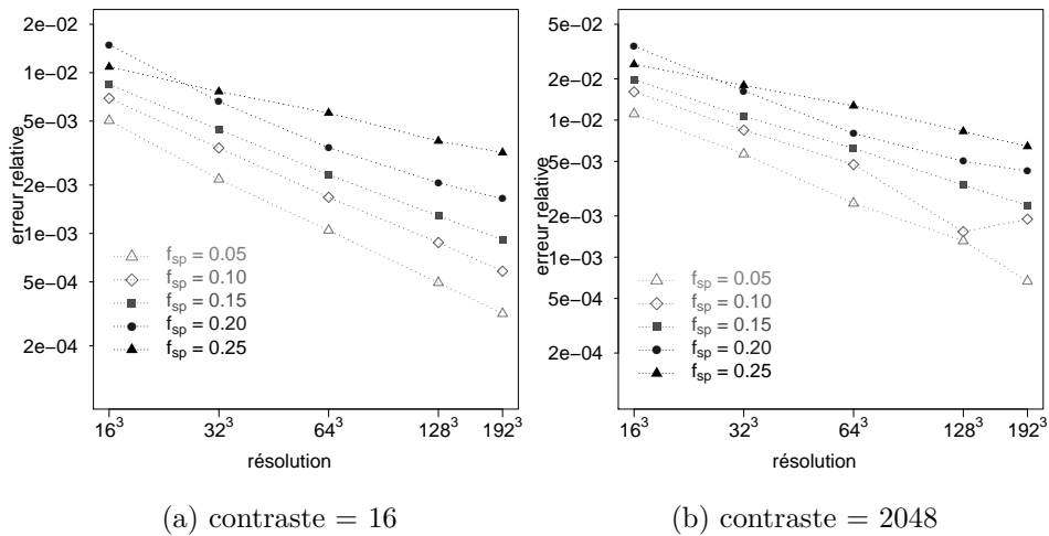
Figure 1.13 – Erreur relative du module de compressibilité effectif selon la fraction volumique de la sphère f_{sp} (contraste de 16 et 2048, résolution de 16^3 à 192^3 )
