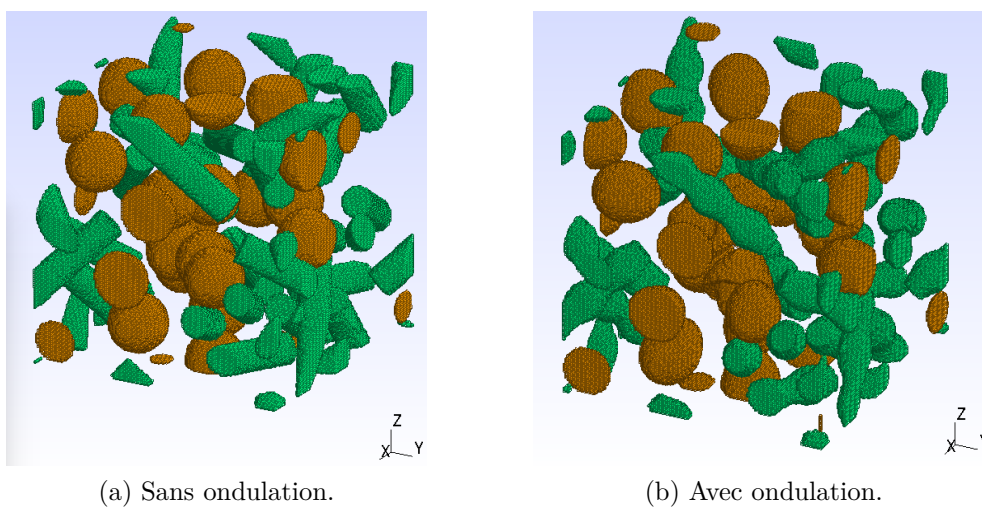
Figure 2.10 – Comparaison d'un VER sans et avec ondulation des inclusions.
