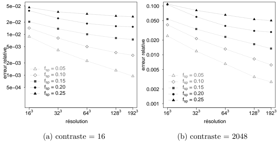
Figure 1.14 – Erreur relative du module de cisailage effectif selon la fraction volumique de la sphère f_{sp} (contraste de 16 et 2048, résolution de 16^3 à 192^3 )
