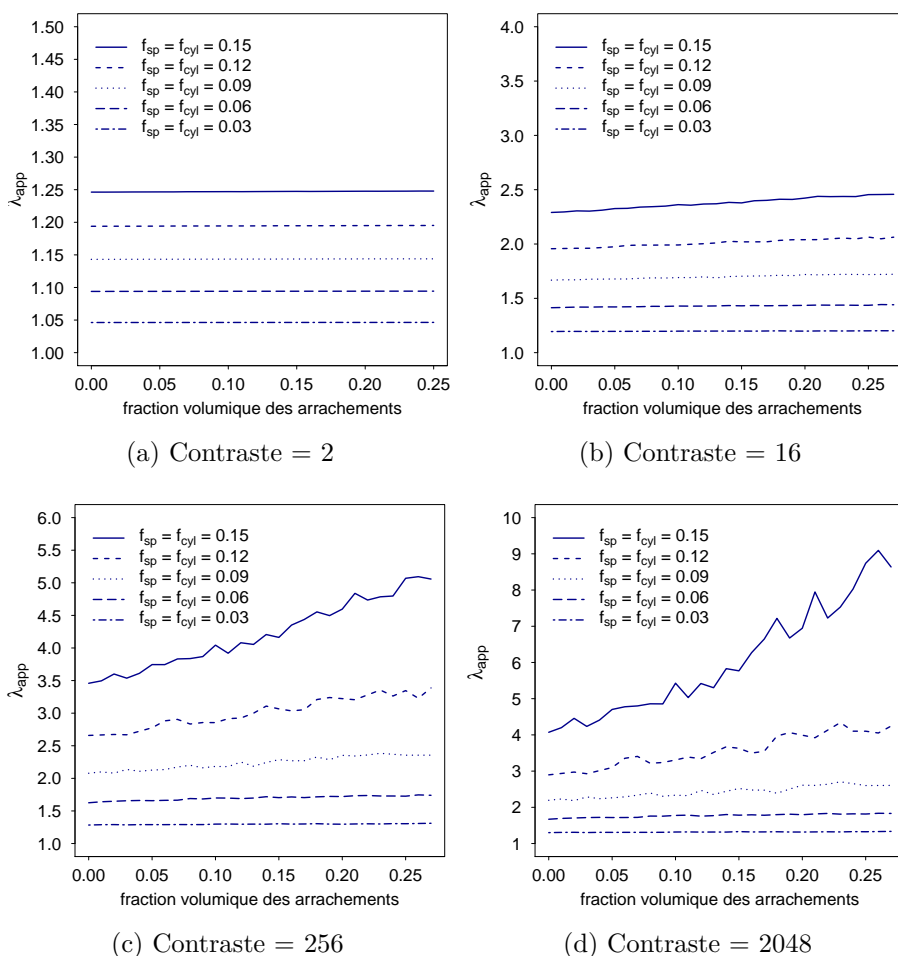
Figure 3.9 – Évolution de la conductivité thermique apparente normalisée d'un matériau composite à inclusions cylindriques de facteur de forme 3 et sphériques en fonction de la fraction volumique des arrachements ( f_{cyl} = f_{sp} = 0.03, 0.06, 0.09, 0.12, 0.15 , n_{cyl} = n_{sp} = 20 , contraste = 2, 16, 256, 2048)
