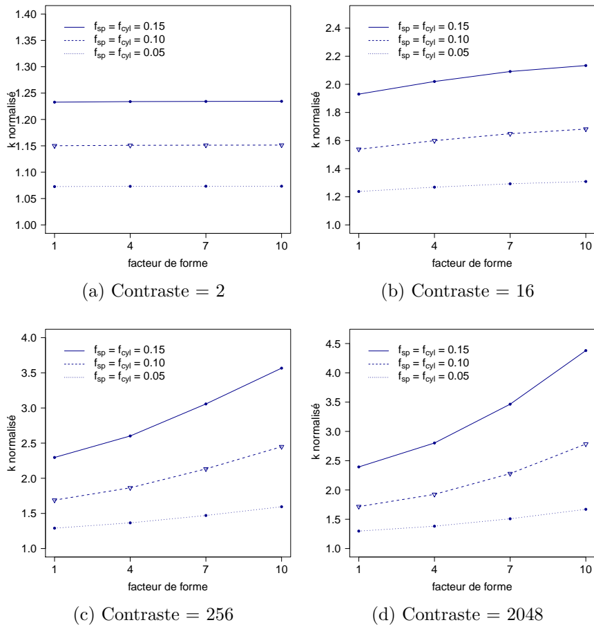
Figure 4.7 – Évolution du coefficient de compressibilité homogénéisé d’un matériau composite à inclusions cylindriques et sphériques ( n_{cyl} = n_{sp} = 20 ) en fonction du facteur de forme ( f_{cyl} = f_{sp} = 0.05, 0.1, 0.15 , contraste = 2, 16, 256, 2048)
