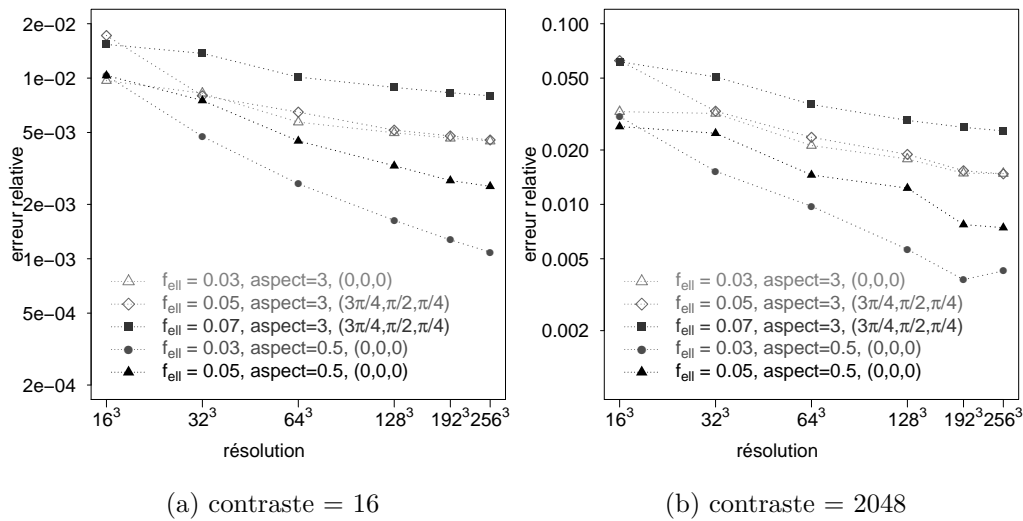
Figure 1.7 – Erreur relative de \lambda_{app} pour les cinq ellipsoïdes (contraste de 16 et 2048, résolution de 16^3 à 256^3 )
