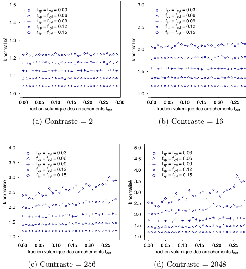
Figure 4.17 – Évolution du coefficient de compressibilité homogénéisé k d'un matériau composite à inclusions cylindriques de facteur de forme 3 et sphériques en fonction de la fraction volumique des arrachements ( f_{cyl} = f_{sp} = 0.03, 0.06, 0.09, 0.12, 0.15 , n_{cyl} = n_{sp} = 20 , contraste = 2, 16, 256, 2048)
