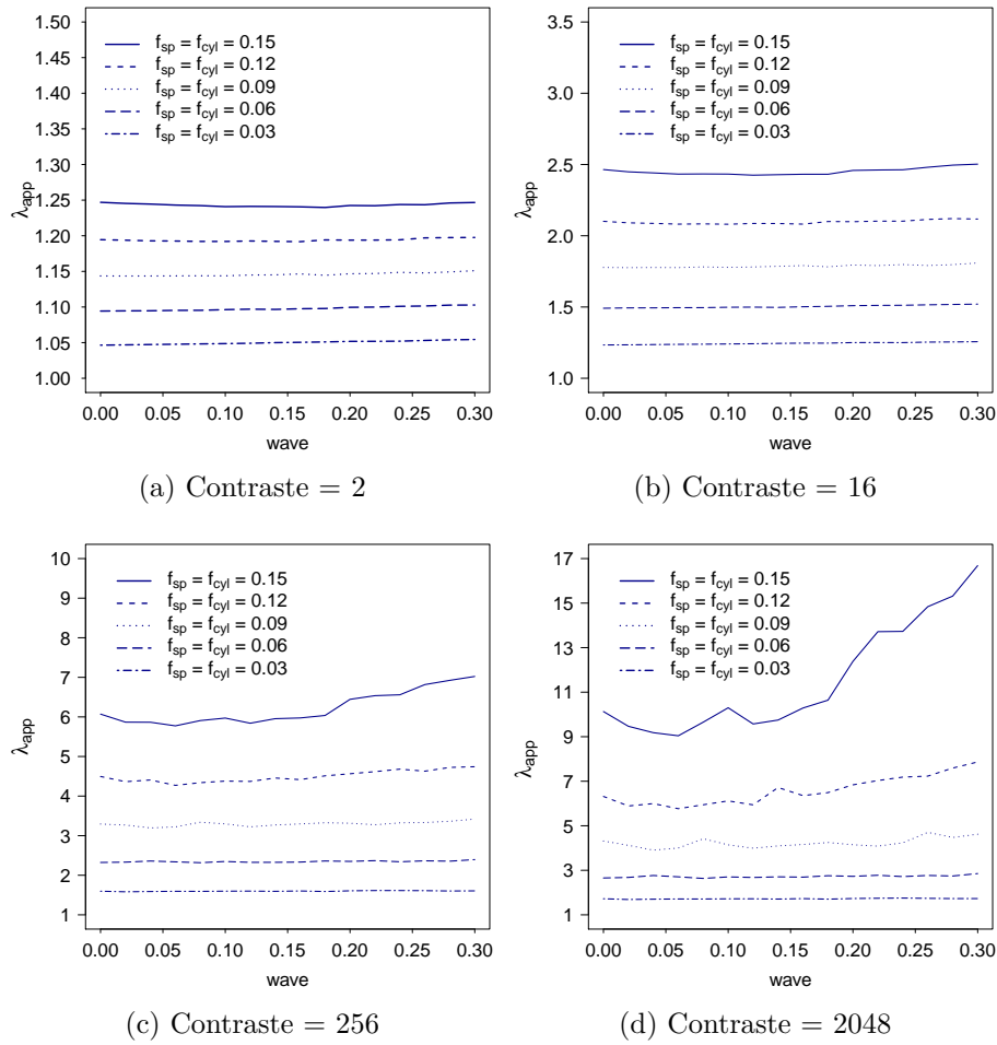
Figure 3.8 – Évolution de la conductivité thermique apparente normalisée d'un matériau composite à inclusions cylindriques de facteur de forme 9 et sphériques en fonction de l'amplitude d'ondulation des surfaces des inclusions ( f_{cyl} = f_{sp} = 0.03, 0.06, 0.09, 0.12, 0.15 , n_{cyl} = n_{sp} = 20 , contraste = 2, 16, 256, 2048)
