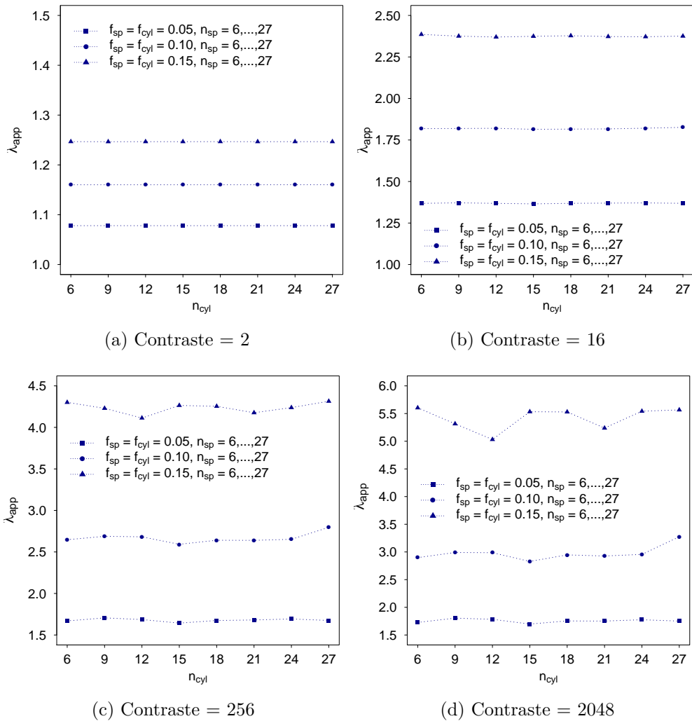
Figure 3.4 – Évolution de la conductivité thermique apparente normalisée d'un matériau composite à inclusions cylindriques et sphériques en fonction du nombre d'inclusions (facteur de forme = 5, contraste = 2, 16, 256, 2048)
