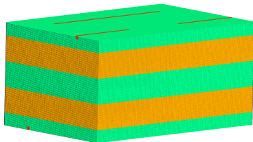
(a) Vue générale du stratifié cousu
