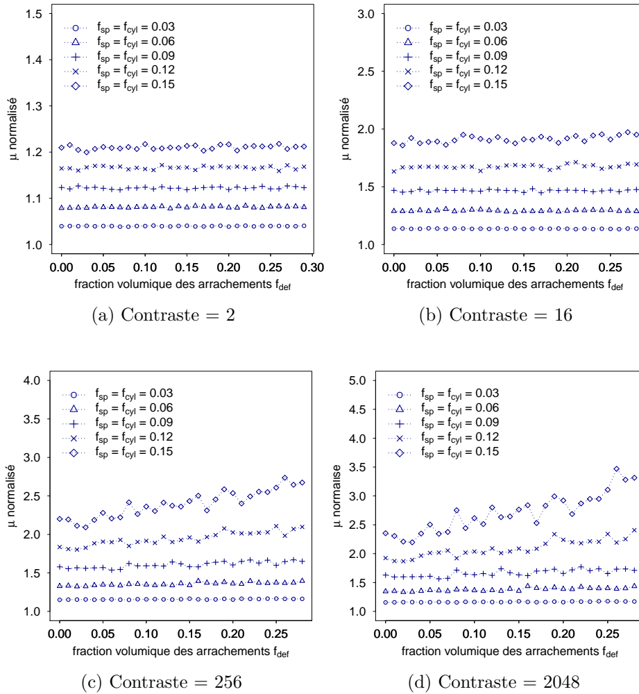
Figure 4.18 – Évolution du coefficient de cisaillement homogénéisé \mu d'un matériau composite à inclusions cylindriques de facteur de forme 3 et sphériques en fonction de la fraction volumique des arrachements ( f_{cyl} = f_{sp} = 0.03, 0.06, 0.09, 0.12, 0.15 , n_{cyl} = n_{sp} = 20 , contraste = 2, 16, 256, 2048)
