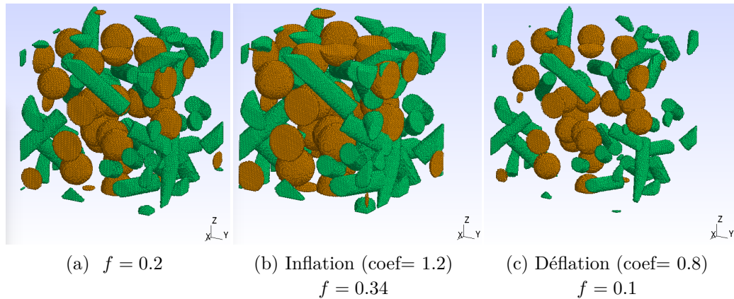
Figure 2.17 – Inflation et déflation des inclusions d'un VER
