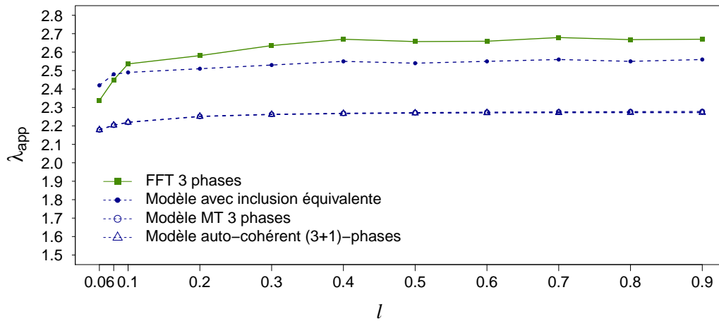
Figure 5.7 – Évolution de la conductivité thermique apparente en fonction du ratio d'épaisseur l \geq 0.06 de la pellicule en 256^3 (en W.K^{-1}.m^{-1} )
