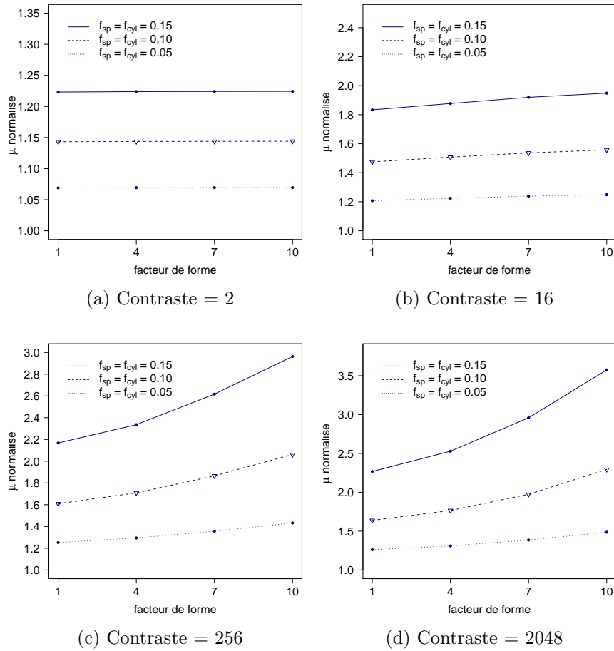
Figure 4.8 – Évolution du coefficient de cisaillement homogénéisé d'un matériau composite à inclusions cylindriques et sphériques ( n_{cyl} = n_{sp} = 20 ) en fonction du facteur de forme ( f_{cyl} = f_{sp} = 0.05, 0.1, 0.15 , contraste = 2, 16, 256, 2048)
