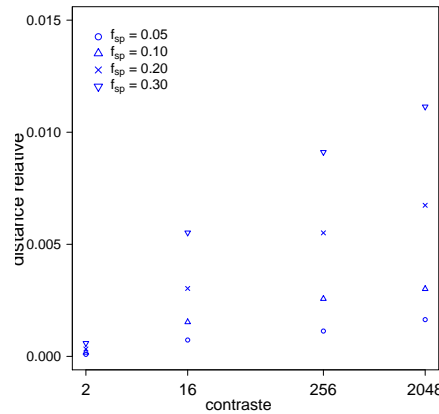
Figure 4.1 – Évolution de la distance relative à l'isotropie en fonction du contraste pour un échantillon de n = 10 VER à inclusions sphériques ( n_{sp} = 20 , f_{sp} = 0.05, 0.1, 0.2, 0.3 ).
