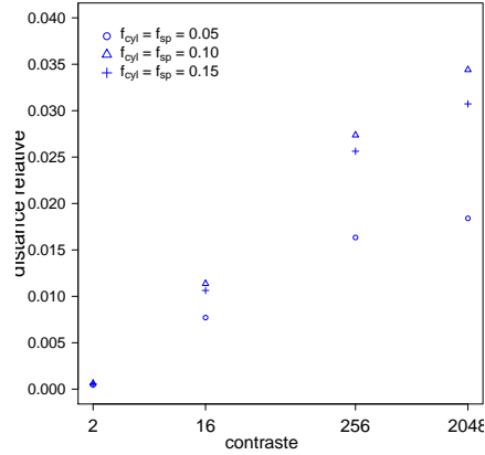
Figure 4.3 – Évolution de la distance relative à l’isotropie en fonction du contraste pour un échantillon de n = 10 VER à inclusions sphériques et cylindriques ( n_{sp} = n_{cyl} = 20 , f_{sp} = f_{cyl} = 0.05, 0.1, 0.15 , facteur de forme = 5).
