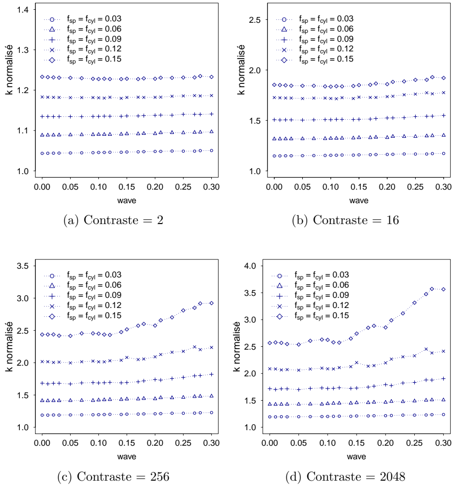
Figure 4.13 – Évolution du coefficient de compressibilité homogénéisé d'un matériau composite à inclusions cylindriques de facteur de forme 3 et sphériques en fonction de l'amplitude d'ondulation des surfaces des inclusions ( f_{cyl} = f_{sp} = 0.03, 0.06, 0.09, 0.12, 0.15 , n_{cyl} = n_{sp} = 20 , contraste = 2, 16, 256, 2048)
