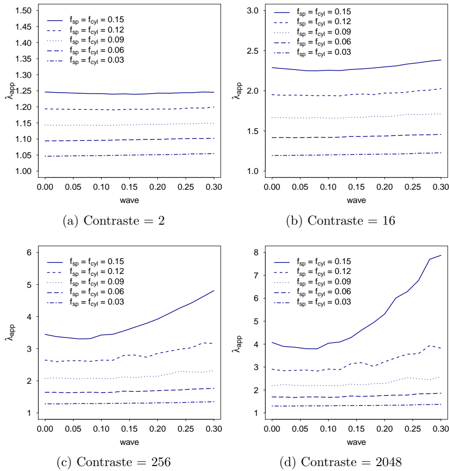
Figure 3.7 – Évolution de la conductivité thermique apparente normalisée d'un matériau composite à inclusions cylindriques de facteur de forme 3 et sphériques en fonction de l'amplitude d'ondulation des surfaces des inclusions ( f_{cyl} = f_{sp} = 0.03, 0.06, 0.09, 0.12, 0.15 , n_{cyl} = n_{sp} = 20 , pour des contrastes = 2, 16, 256, 2048)
