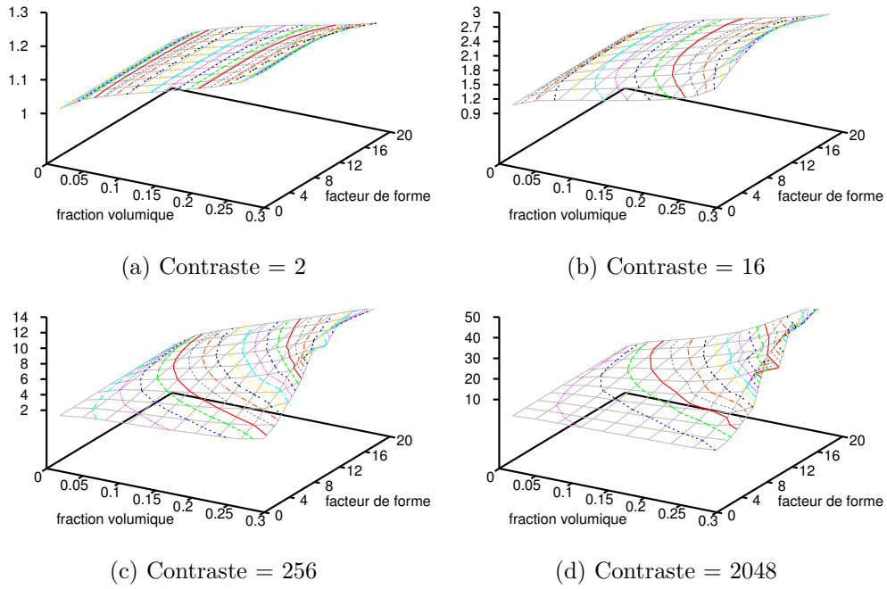
Figure 3.2 – Évolution de la conductivité thermique apparente normalisée d'un matériau composite à inclusions cylindriques ( n_{cyl} = 20 ) en fonction de la fraction volumique ( f_{cyl} ) et du facteur de forme, pour des contrastes = 2, 16, 256, 2048
