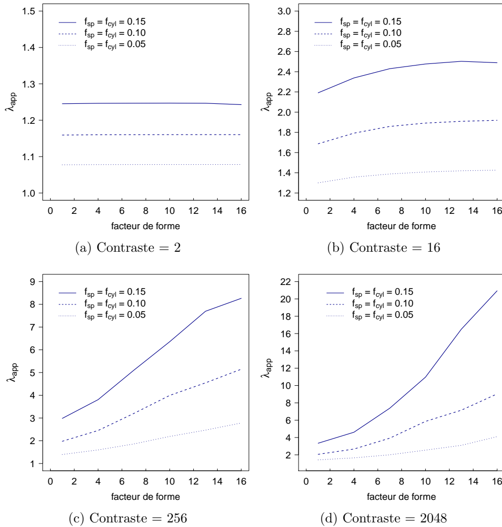
Figure 3.3 – Évolution de la conductivité thermique apparente normalisée d'un matériau composite à inclusions cylindriques et sphériques ( n_{cyl} = n_{sp} = 20 ) en fonction du facteur de forme, pour des contrastes = 2, 16, 256, 2048
