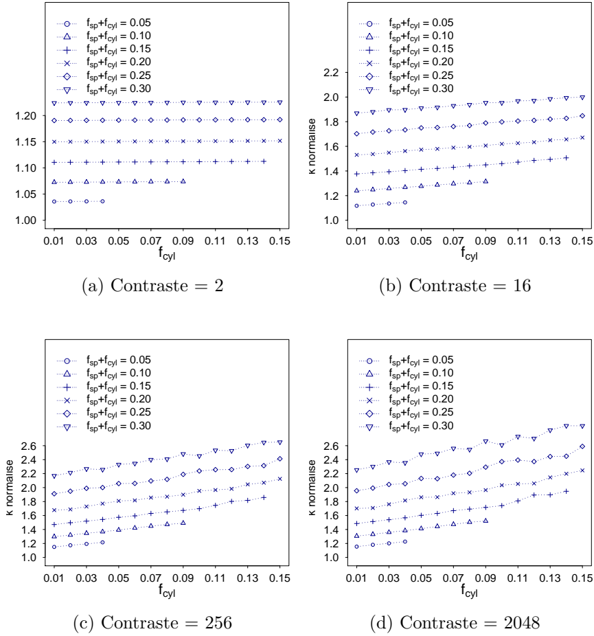
Figure 4.11 – Évolution du coefficient de compressibilité homogénéisé d'un matériau composite à inclusions cylindriques et sphériques en fonction des fractions volumiques f_{cyl} et f_{sp} respectives ( n_{cyl} = n_{sp} = 20 , facteur de forme = 5, contraste = 2, 16, 256, 2048)
