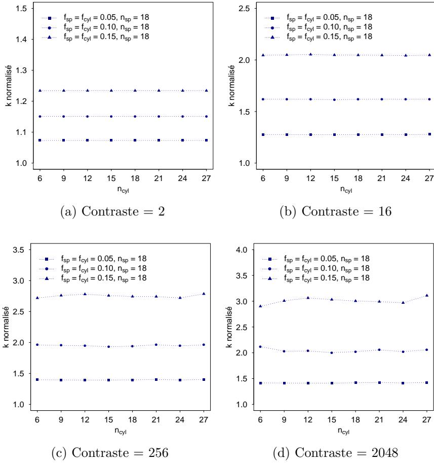
Figure 4.9 – Évolution du coefficient de compressibilité homogénéisé d'un matériau composite à inclusions cylindriques et sphériques en fonction de n_{cyl} à n_{sp} fixé à 18 ( f_{cyl} = f_{sp} = 0.05, 0.1, 0.15 , facteur de forme = 5, contraste = 2, 16, 256, 2048)
