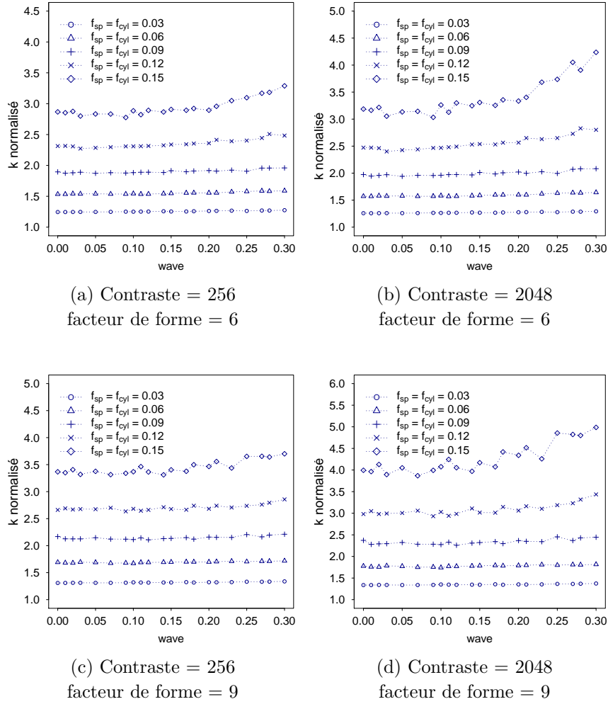
Figure 4.15 – Évolution du coefficient de compressibilité homogénéisé d'un matériau composite à inclusions cylindriques (de facteur de forme 6 et 9) et sphériques en fonction de l'amplitude d'ondulation des surfaces des inclusions ( f_{cyl} = f_{sp} = 0.03, 0.06, 0.09, 0.12, 0.15 , n_{cyl} = n_{sp} = 20 , contraste = 256, 2048)
