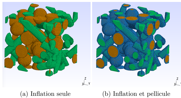
Figure 2.18 – Comparaison en vue 3D du VER généré composé de 20 sphères et 20 cylindres d'inflation de facteur 1.2 sans et avec pellicule de ratio 0.3, f = 0.34 .
