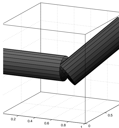
Figure E.10 – Deux cylindres, intersection de type d1 ou d2 .
