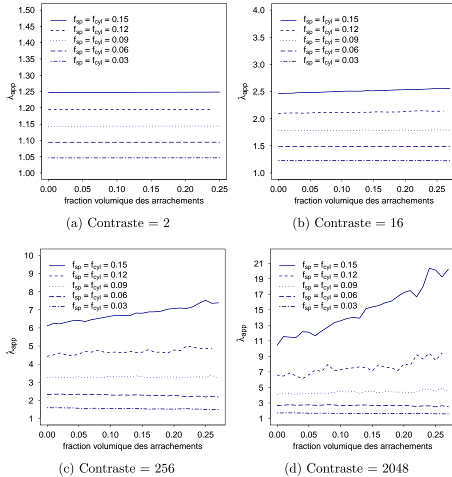
Figure 3.10 – Évolution de la conductivité thermique apparente normalisée d'un matériau composite à inclusions cylindriques de facteur de forme 9 et sphériques en fonction de la fraction volumique des arrachements ( f_{cyl} = f_{sp} = 0.03, 0.06, 0.09, 0.12, 0.15 , n_{cyl} = n_{sp} = 20 , contraste = 2, 16, 256, 2048)
