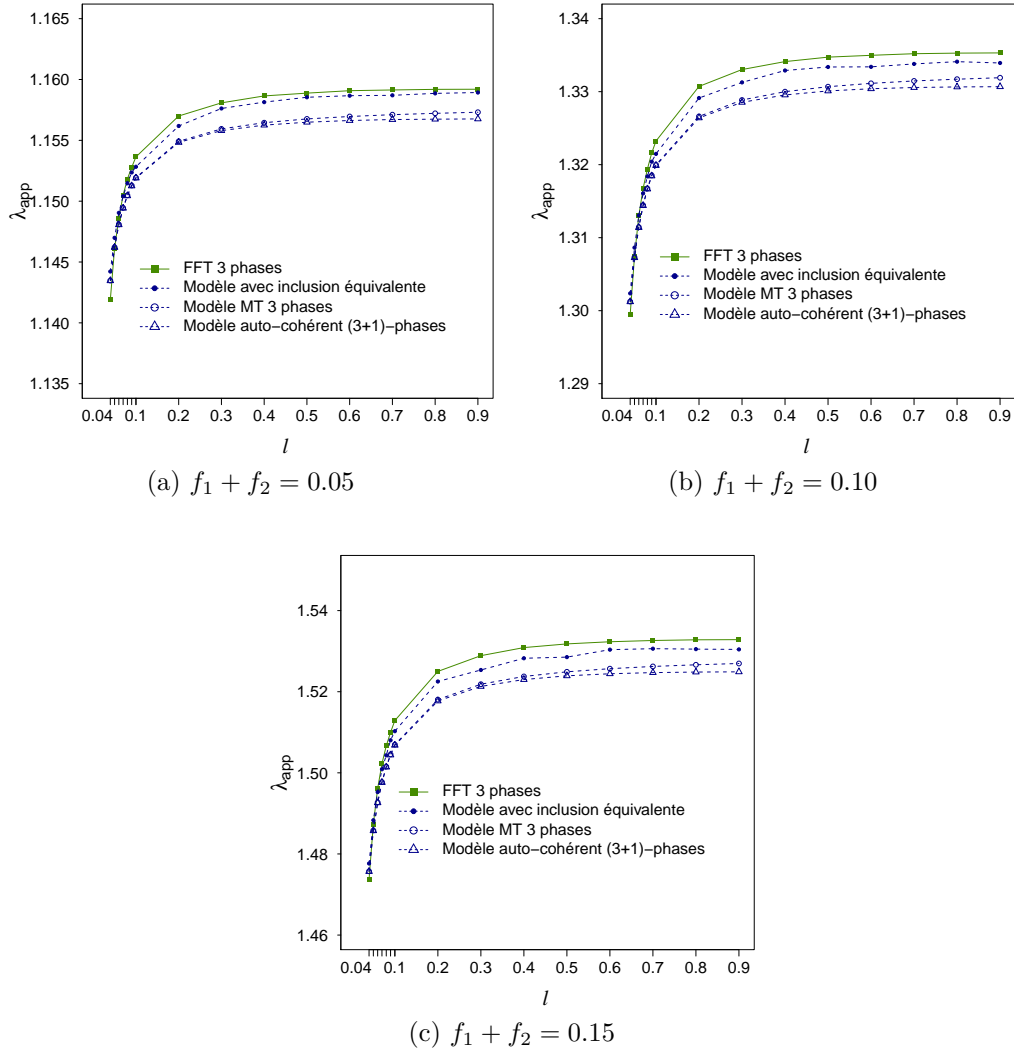
Figure 5.4 – Comparaison des modèles auto-cohérent (3+1)-phases, de Mori-Tanaka (3 phases), avec inclusion équivalente et la FFT (en W.K^{-1}.m^{-1} )
