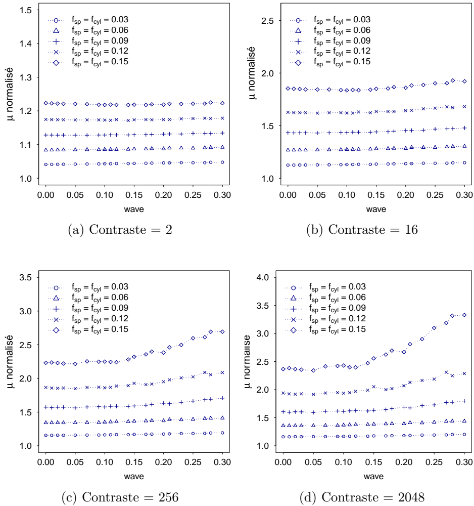
Figure 4.14 – Évolution du coefficient de cisaillement homogénéisé d'un matériau composite à inclusions cylindriques de facteur de forme 3 et sphériques en fonction de l'amplitude d'ondulation des surfaces des inclusions ( f_{cyl} = f_{sp} = 0.03, 0.06, 0.09, 0.12, 0.15 , n_{cyl} = n_{sp} = 20 , contraste = 2, 16, 256, 2048)
