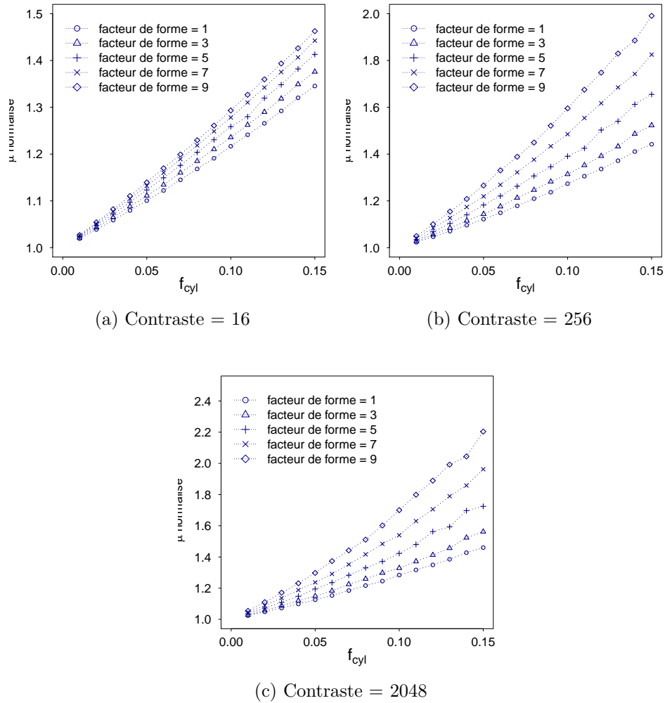
Figure 4.6 – Évolution du coefficient de compressibilité homogénéisé d'un matériau composite à inclusions cylindriques ( n_{\text{cyl}} = 20 ) en fonction de la fraction volumique et du facteur de forme (contraste = 16, 256, 2048)
