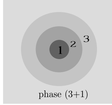
Figure 5.3 – Modèle auto-cohérent (3+1)-phases
