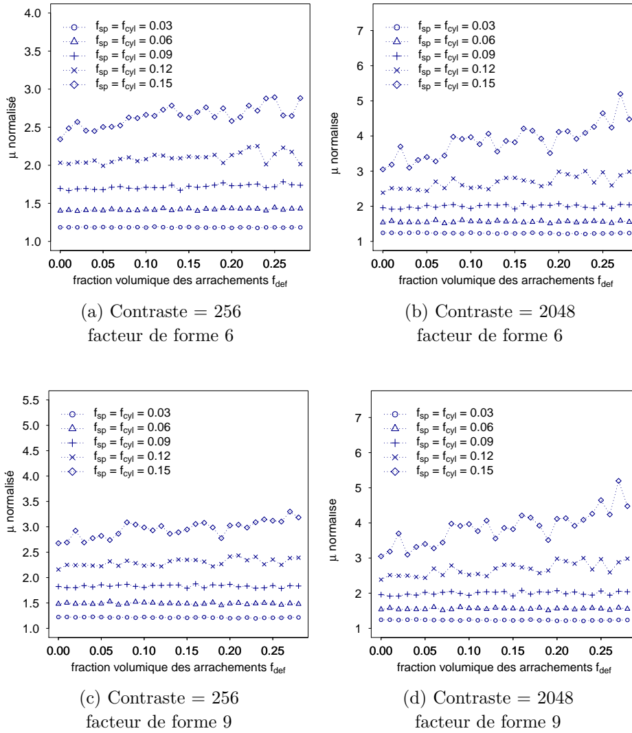
Figure 4.20 – Évolution du coefficient de cisaillement homogénéisé \mu d'un matériau composite à inclusions cylindriques (de facteur de forme 6 et 9) et sphériques en fonction de la fraction volumique des arrachements ( f_{cyl} = f_{sp} = 0.03, 0.06, 0.09, 0.12, 0.15 , n_{cyl} = n_{sp} = 20 , contraste = 256, 2048)
