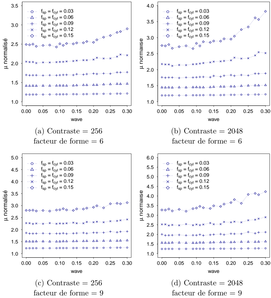
Figure 4.16 – Évolution du coefficient de cisaillement homogénéisé d'un matériau composite à inclusions cylindriques (de facteur de forme 6 et 9) et sphériques en fonction de l'amplitude d'ondulation des surfaces des inclusions ( f_{cyl} = f_{sp} = 0.03, 0.06, 0.09, 0.12, 0.15 , n_{cyl} = n_{sp} = 20 , contraste = 256, 2048)
