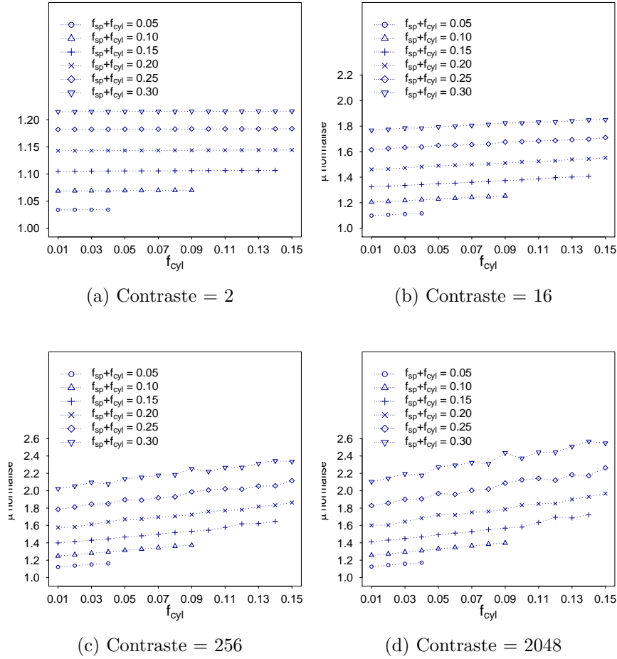
Figure 4.12 – Évolution du coefficient de cisaillement homogénéisé d'un matériau composite à inclusions cylindriques et sphériques en fonction des fractions volumiques f_{cyl} et f_{sp} respectives ( n_{cyl} = n_{sp} = 20 , facteur de forme = 5, contraste = 2, 16, 256, 2048)
