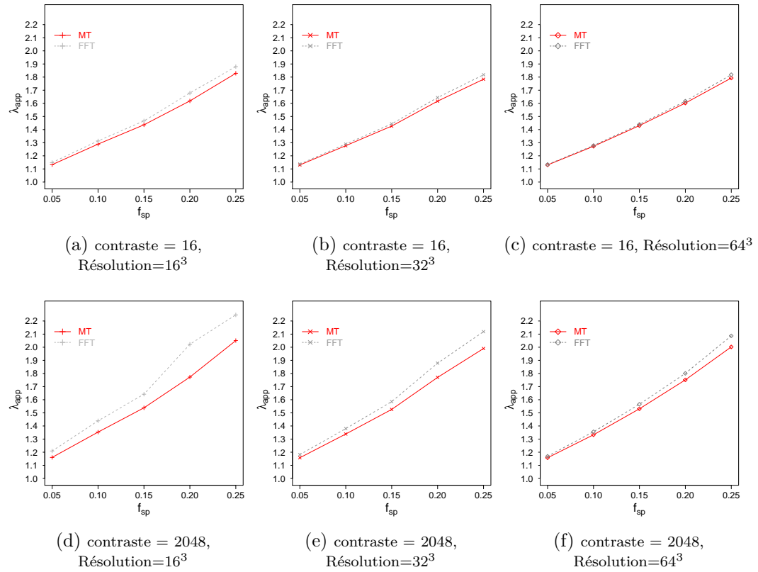
Figure 1.3 – Comparaison de \lambda_{app} entre le modèle de Mori-Tanaka (en rouge) et le calcul numérique par le schéma accéléré (en gris) en fonction de la fraction volumique de la sphère f_{sp} (contraste de 16 et 2048, résolution de 16^3 à 64^3 )
