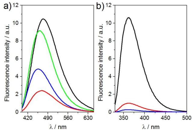
Figure R10. Spectres d'émission des séquences (-)PBS marquées avec d^{th}G - (a) et d2Ap - (b). (a) nucléoside d^{th}G libre (noir), d^{th}G7(-)PBS (rouge), d^{th}G7(-)/(+)PBS (bleu) et d^{th}G7(-)/T12(+)PBS (vert); (b) nucléoside d2Ap libre (noir), d2Ap7(-)PBS (rouge), et d2Ap7(-)/T12(+)PBS (bleu).
