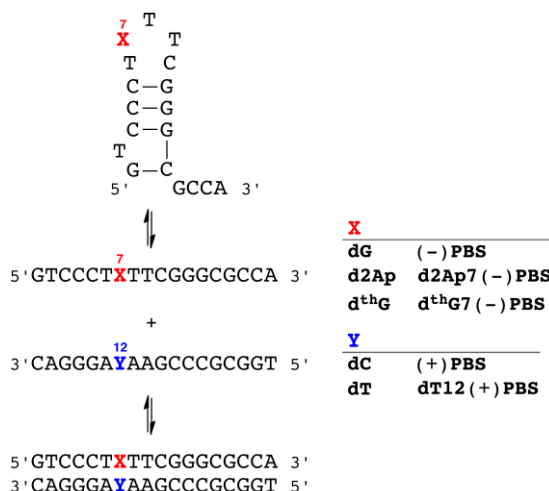
Figure R9. Séquence de l'amorce du site de liaison de (-)PBS montrée en simple brin, (milieu), tige boucle (haut) et en duplex avec (+)PBS (bas). Sont aussi montrées les séquences spécifiquement modifiées contenant d2Ap et d th G.
