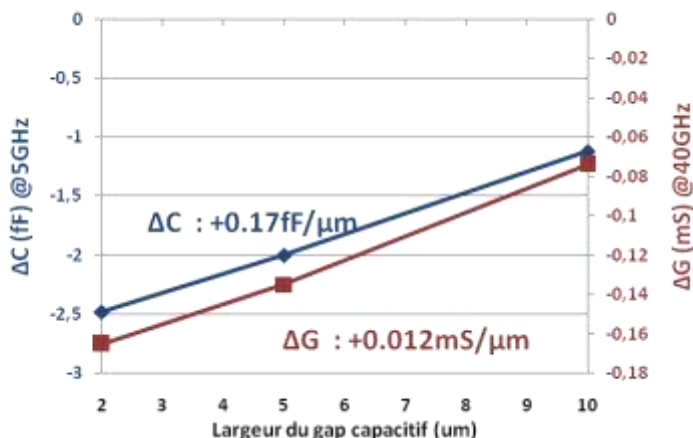
Figure II. 29 Tableau des contrastes \Delta C et \Delta G à 5 GHz et 40 GHz respectivement (gauche) et les contrastes \Delta C et \Delta G versus la largeur du gap capacitif (droite)
