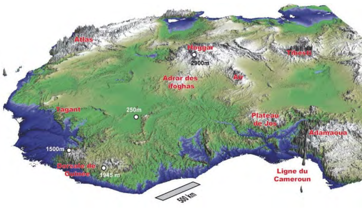
Figure 2-2 Vue oblique vers le NE de la topographie NW de l'Afrique (Grimaud, 2014).
