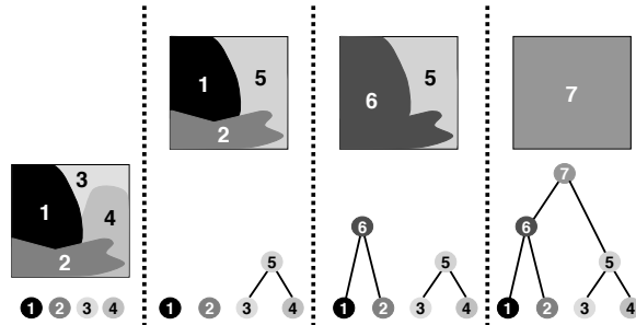
FIGURE 3 – Exemple de construction d'Arbre Binaire de Partitions
