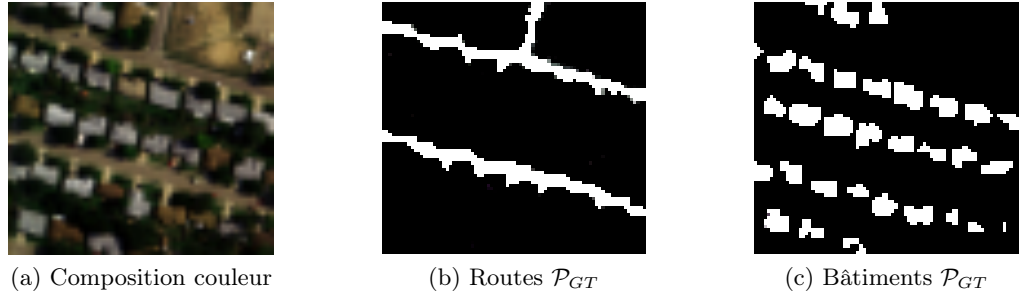
FIGURE 13 – Données Hydice
