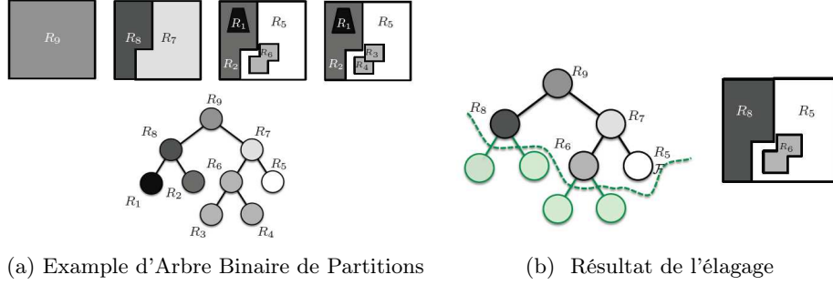
FIGURE 4 – Exemple d’élague de l’Arbre Binaire de Partitions
