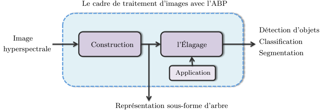
FIGURE 5 – Le traitement d'images hyperspectral en utilisant l'ABP
