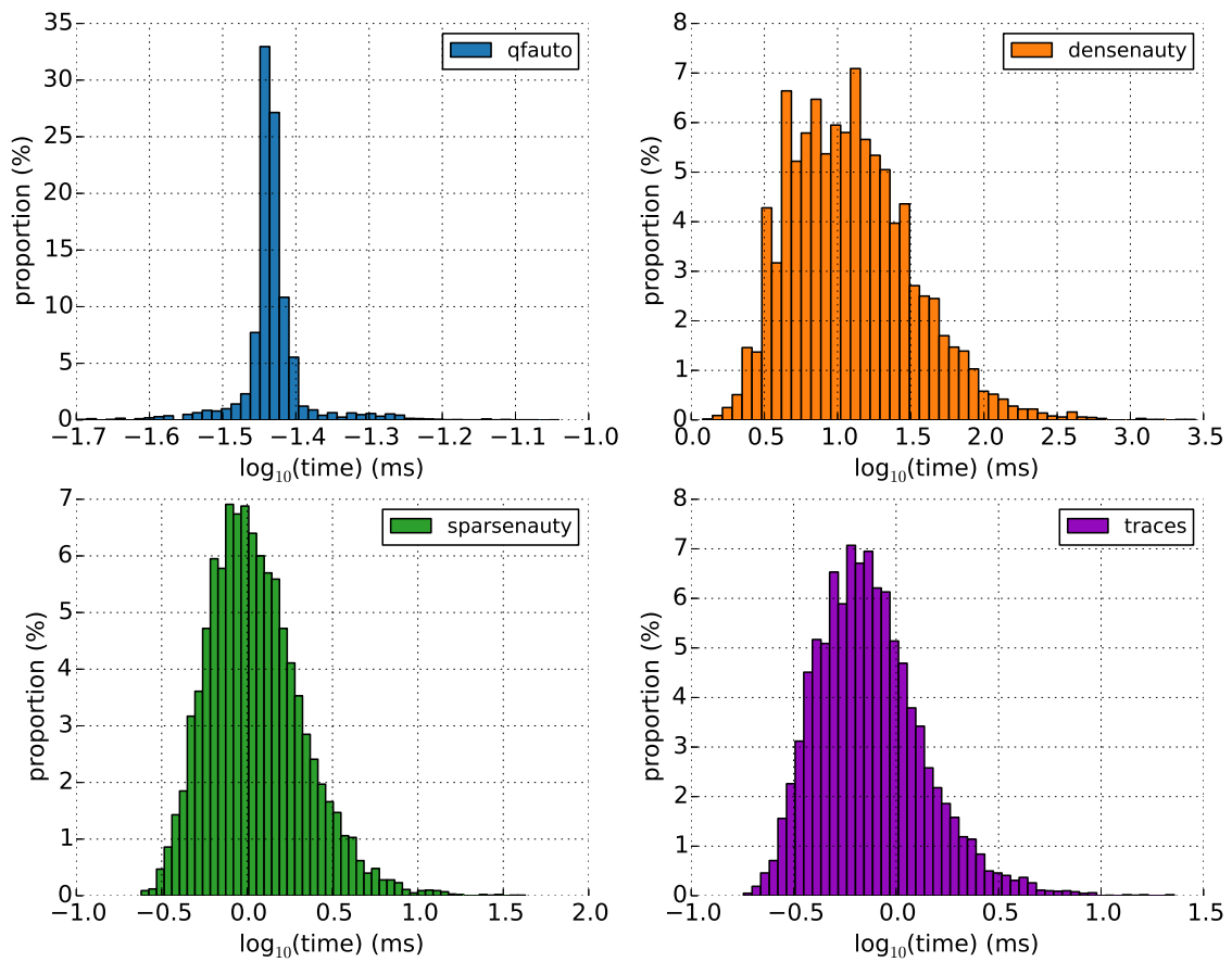
Fig. V.12 – Comparaison des temps de calculs sur 10000 réseaux aléatoires de dimension 20.
