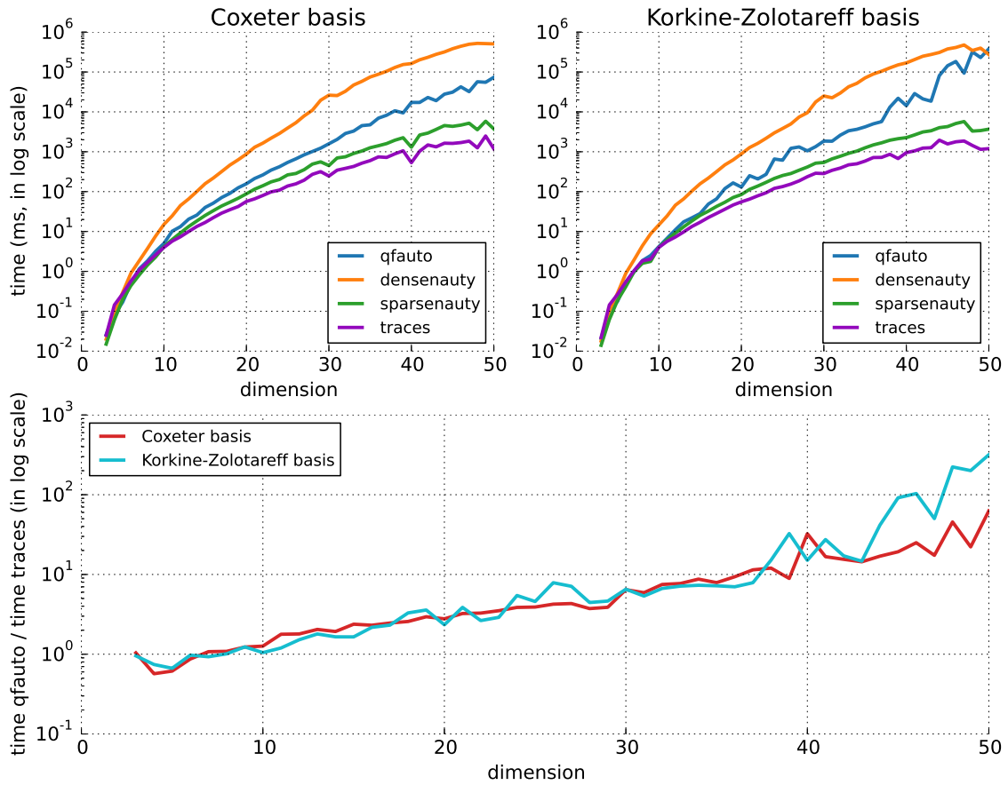
Fig. V.9 – Comparaison des temps de calculs sur deux bases différentes du réseau \mathbb{D}_n pour 3 \leq n \leq 50 . Le graphe inférieur représente le rapport temps de calcul de qfauto / temps de calcul de Traces.
