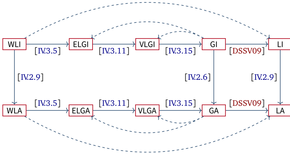
Fig. IV.11 – Résumé des réductions obtenues. Les flèches correspondent à des réductions polynomiales, les flèches en traits pointillés à des réductions triviales.
