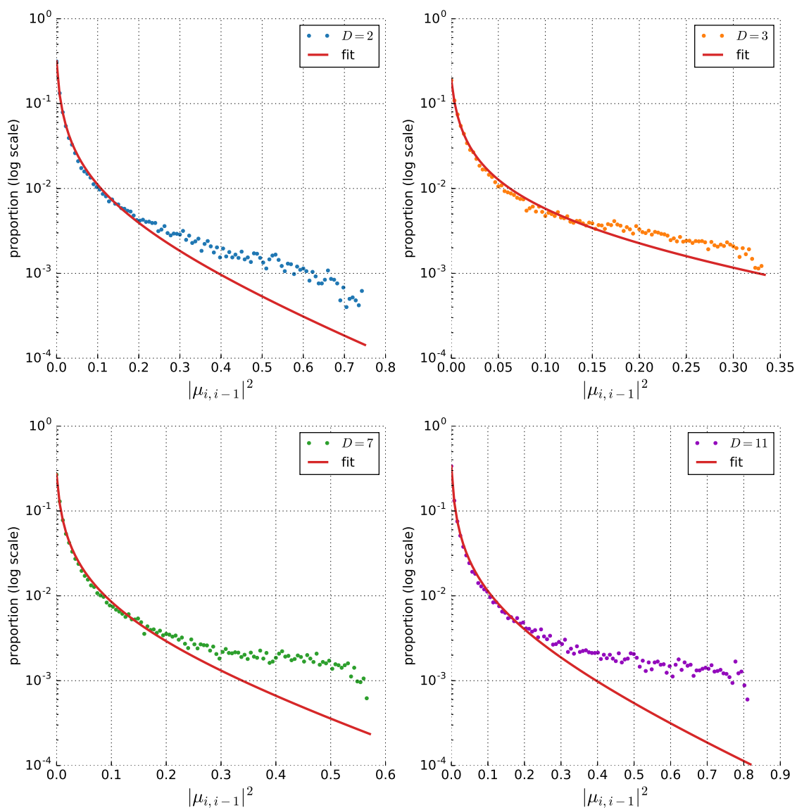
Fig. 1.7 – Distribution et interpolations obtenues pour K = \mathbb{Q}(i\sqrt{D}) avec D \in \{2, 3, 7, 11\} et \delta = 0,99 (échelles logarithmiques).
