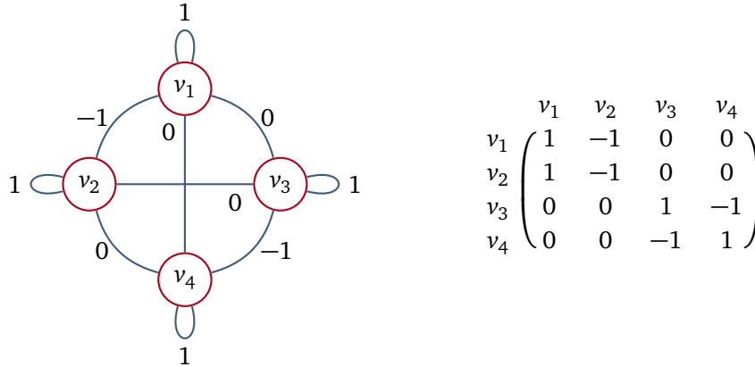
Fig. IV.5 – Le graphe étiqueté G(\mathbb{Z}^2, \mathcal{B}) et sa matrice d'incidence.
