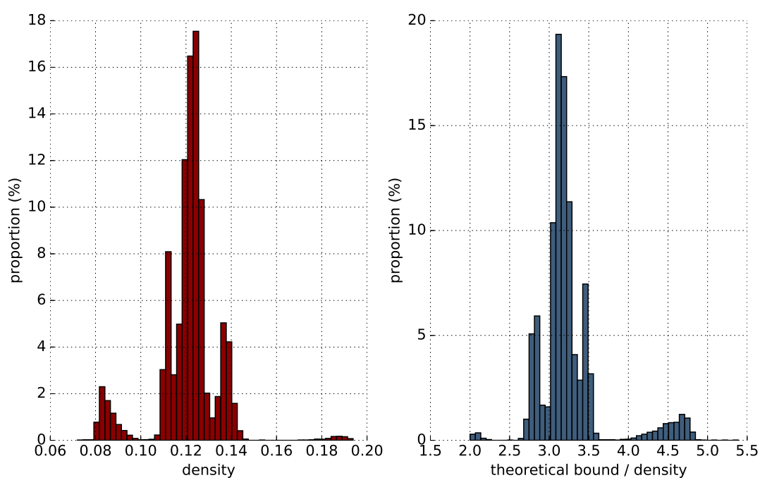
Fig. IV.8 – Densité des graphes associés aux 10916 réseaux parfaits de dimension 8 et comparaison avec la borne théorique (IV.2).
