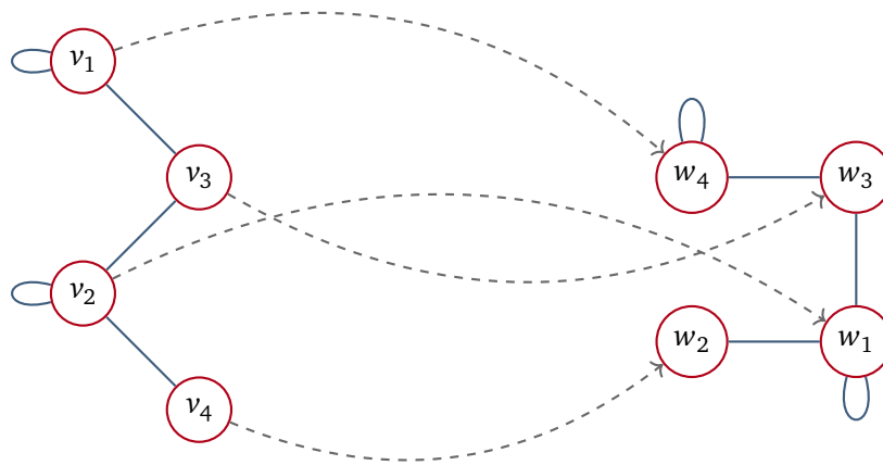
Fig. IV.2 – Exemple de graphes isomorphes.
