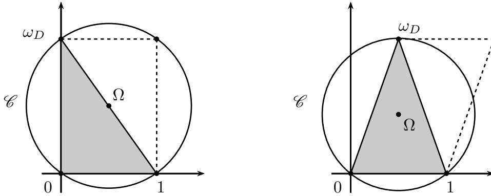
Fig. 1.2 – Centre du cercle inscrit du demi-parallélogramme fondamental de \mathcal{O}_K pour d \equiv 1, 2 \pmod{4} (à gauche) et d \equiv 3 \pmod{4} (à droite).
