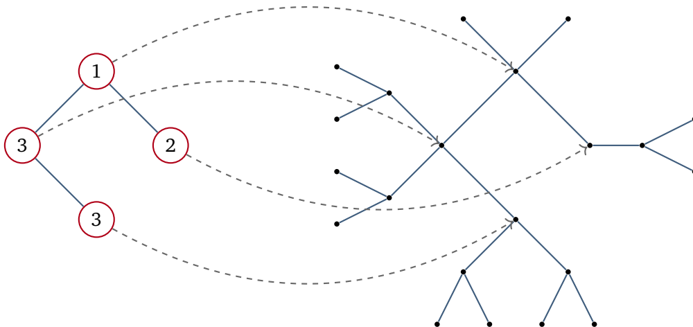
Fig. IV.10 – Exemple de décoloration d'un graphe.
