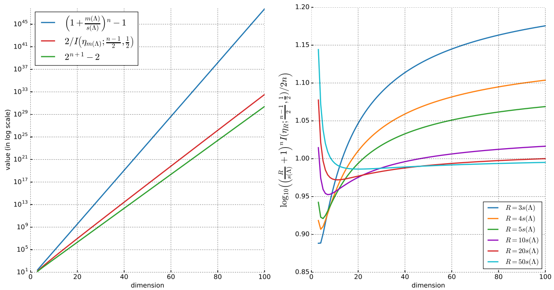
Fig. IV.12 – Comparaison des bornes obtenues. À gauche, les bornes (IV.5) et (IV.8) (pour R = m(\Lambda) ), ainsi que la borne (IV.7) (échelle logarithmique). À droite, logarithme du rapport des bornes (IV.6) et (IV.10) pour différentes valeurs de R = \|\mathcal{B}\|_\infty .
