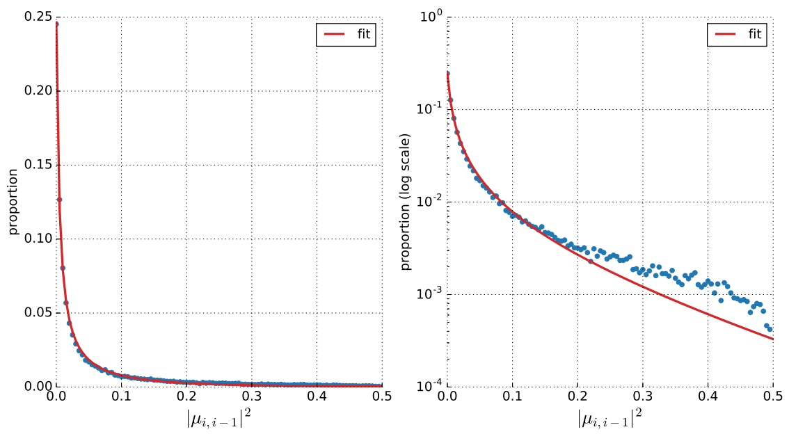
Fig. I.6 – Distribution et interpolations obtenues pour K = \mathbb{Q}(i) et \delta = 0,99 . Échelle linéaire à gauche, logarithmique à droite.
