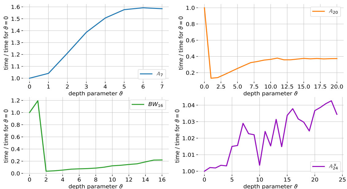
Fig. V.6 – Influence du paramètre de profondeur sur le temps de calcul total du groupe des K_{\mathbb{R}} -automorphismes de A_7 , A_{20} , BW_{16} et A_{24}^V vus comme réseaux algébriques sur \mathbb{Q}(i)_{\mathbb{R}}^n .
