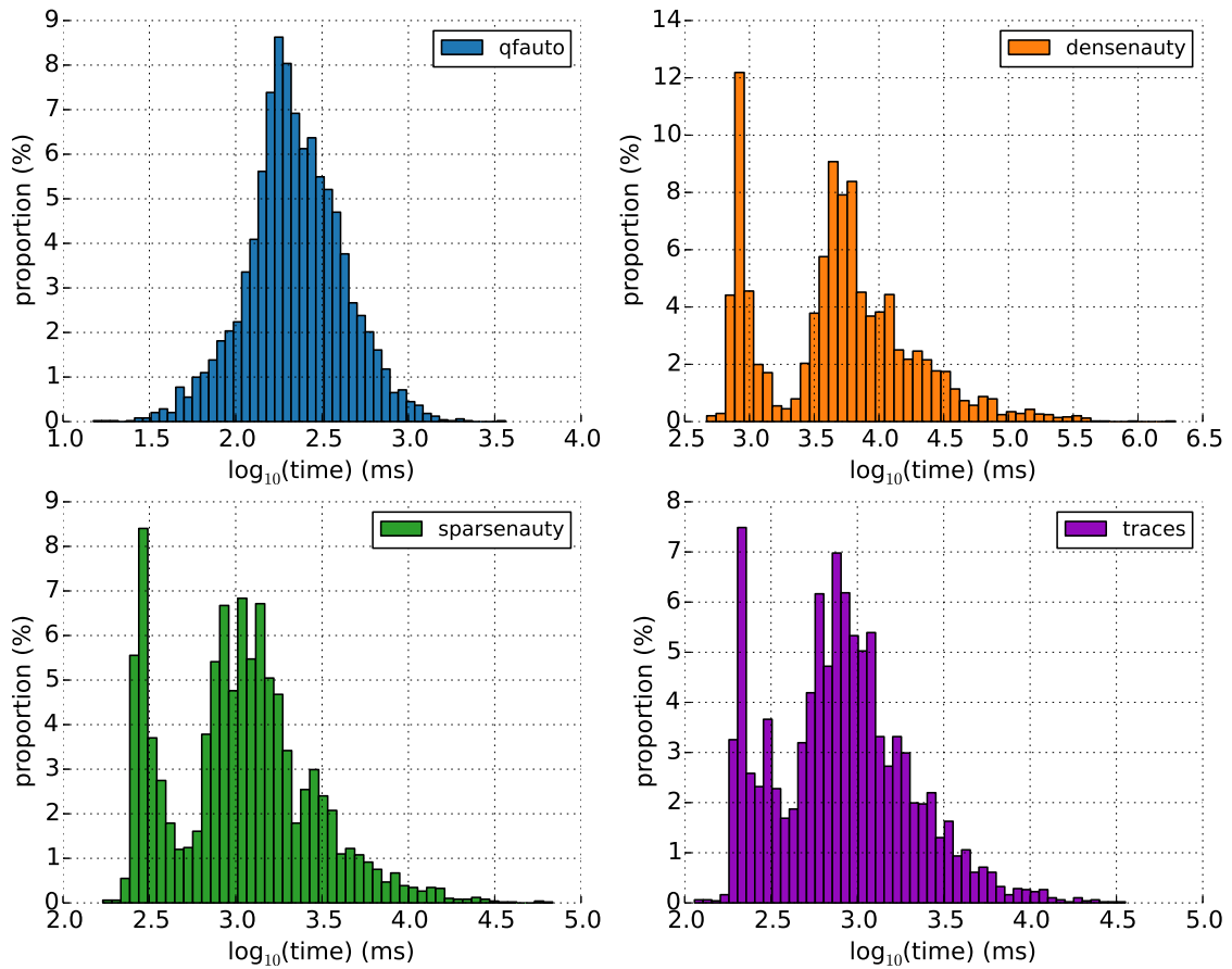
Fig. V.11 – Comparaison des temps de calculs sur les réseaux parfaits de dimension 8.
