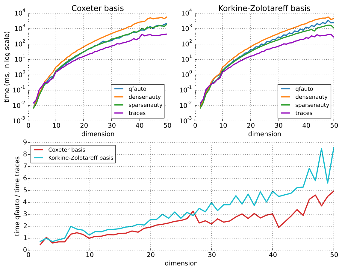
Fig. V.8 – Comparaison des temps de calculs sur deux bases différentes du réseau \mathbb{A}_n pour 2 \leq n \leq 50 . Le graphe inférieur représente le rapport temps de calcul de qfauto / temps de calcul de Traces.
