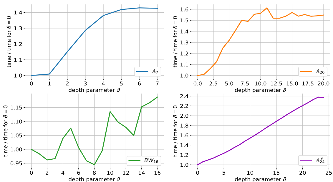
Fig. V.7 – Influence du paramètre de profondeur sur le temps de précalcul lors de la détermination du groupes des K_{\mathbb{R}} -automorphismes de A_7 , A_{20} , BW_{16} et A_{24}^V vus comme réseaux algébriques sur \mathbb{Q}(i)_{\mathbb{R}}^n .
