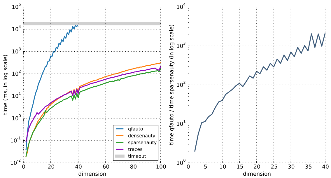
Fig. V.10 – Comparaison des temps de calculs sur les réseaux \mathbb{Z}^n pour 2 \leq n \leq 100 . À droite, le rapport temps de calcul de qfauto / temps de calcul de sparsenauty.
