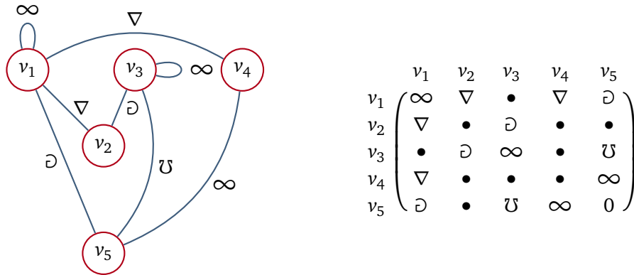
Fig. IV.3 – Exemple de matrice d'incidence associée à un graphe étiqueté.
