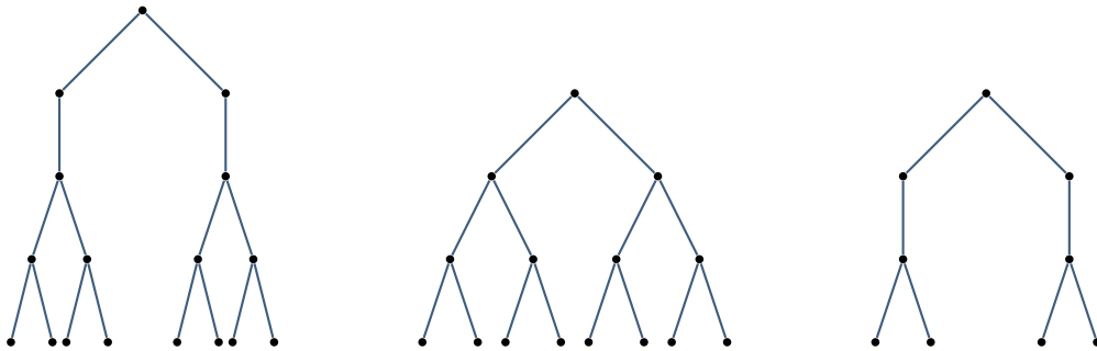
Fig. IV.9 – De gauche à droite, les arbres T_{13} , T_7 et T_6 .
