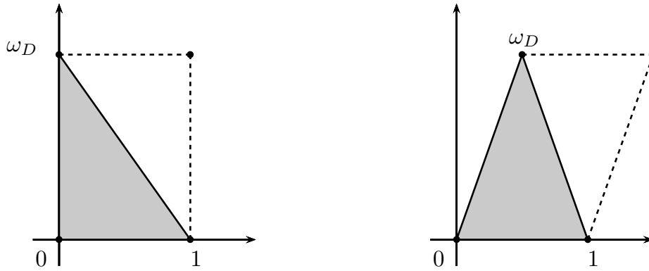
Fig. I.1 – Parallélogramme fondamental de \mathcal{O}_K pour d \equiv 1, 2 \pmod{4} (à gauche) et d \equiv 3 \pmod{4} (à droite).
