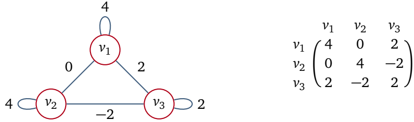
Fig. IV.4 – Le graphe étiqueté G_S et sa matrice d'incidence.
