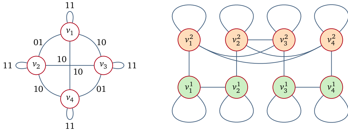
Fig. IV.7 – À gauche, le graphe G(\mathbb{Z}^2, \mathcal{B}) après réétiquetage binaire, à droite le graphe coloré associé.
