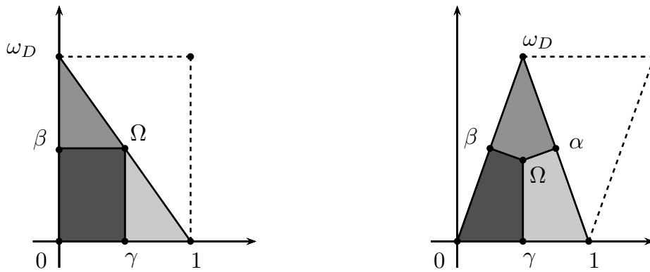
Fig. 1.3 – Partition du demi-parallélogramme fondamental de \mathcal{O}_K pour d \equiv 1, 2 \pmod{4} (à gauche) et d \equiv 3 \pmod{4} (à droite).
