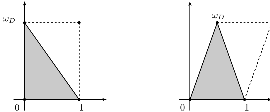
Fig. I.1 – Parallélogramme fondamental de \mathcal{O}_K pour d \equiv 1, 2 \pmod{4} (à gauche) et d \equiv 3 \pmod{4} (à droite).
