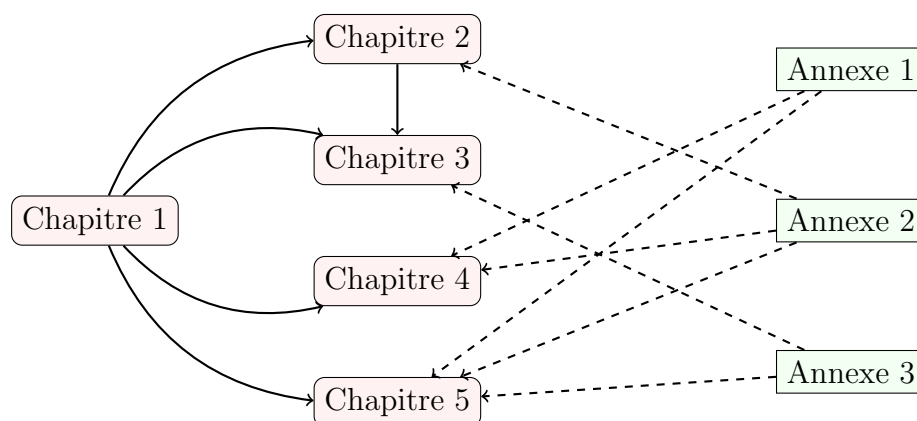
Figure 3: Le graphe de dépendance des chapitres.
