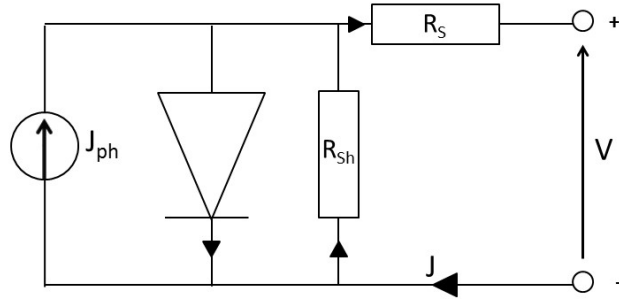
FIGURE 3.10 – Schéma équivalent d'une cellule photovoltaïque avec les résistances parasites
