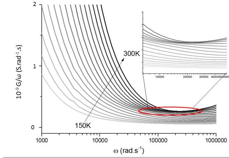
FIGURE 4.17 – Mesures de conductance G/\omega de l'échantillon à base de CZTSSe3
