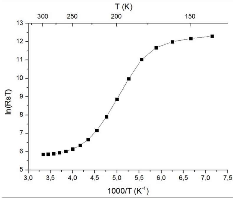
FIGURE 4.24 – Diagramme d'Arrhenius de R_S de CZTSSe1
