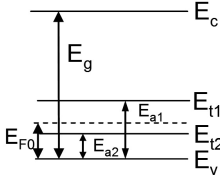
FIGURE 5.1 – Diagramme de bande de l'absorbeur en présence de deux défauts profonds.
