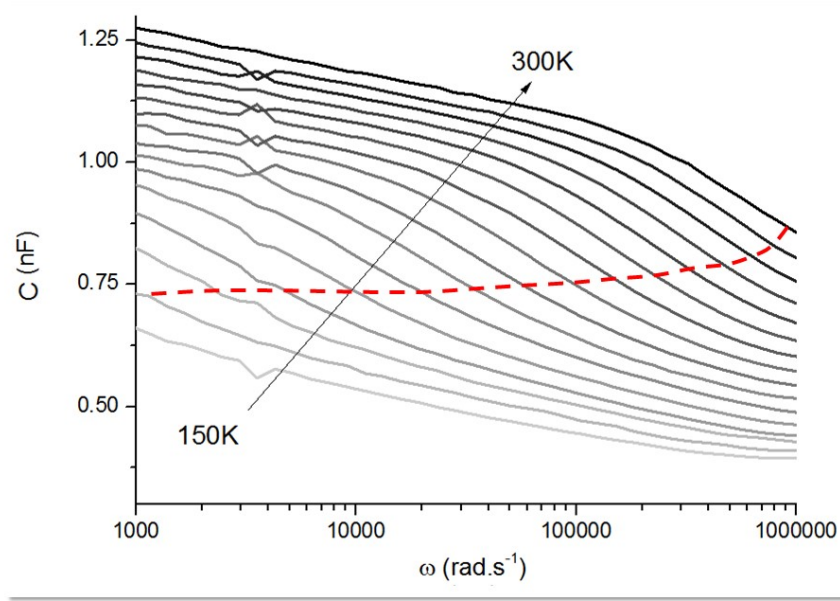
FIGURE 4.15 – Mesures C(\omega) de l'échantillon CZTSSe3
