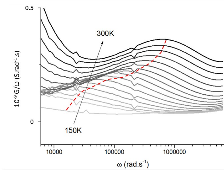
FIGURE 4.11 – Mesures de conductance G(\omega)/\omega de l'échantillon à base de CIGS. La courbe en pointillé représente un guide pour les yeux pour évaluer le déplacement du pic en fréquence pour les différentes températures.
