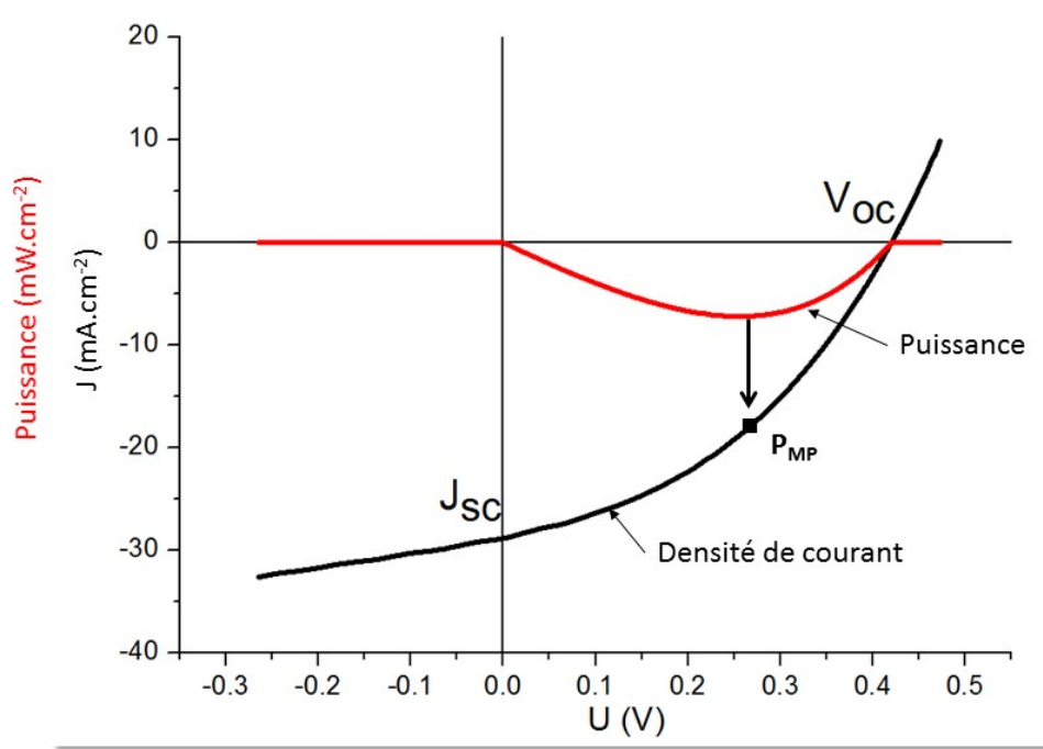
FIGURE 3.12 – Mesure J(V) sous éclaircissement d’une cellule de CZTSSe synthétisée au laboratoire
