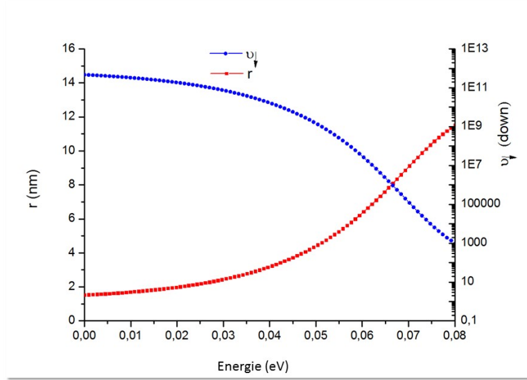
FIGURE 6.19 – Rayon de localisation et probabilité de transition vers un état plus profond en fonction de l'énergie de l'état initial compté à partir de l'énergie de mobilité ( \Gamma=50 meV, N_C=5.10^{20}\text{cm}^{-3} )
