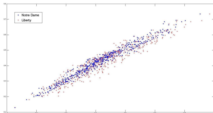
FIGURE 4.4 – Courbe représentant la fréquence que la réponse d’un test soit 1 dans les bases Notre Dame (en bleu) et Liberty (en rouge) en fonction de la fréquence que la réponse d’un test soit 1 dans Yosemite
