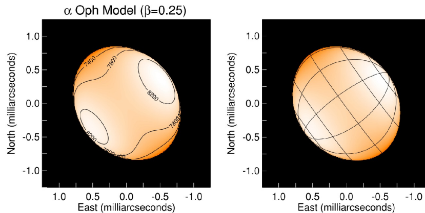
FIGURE 4.2 – Meilleur modèle d’assombrissement gravitationnel pour Rasalhague. À gauche, les contours indiquent les niveaux de température de surface, à droite sont tracés méridiens et parallèles. Figure tirée de ZHAO et al. (2009).
