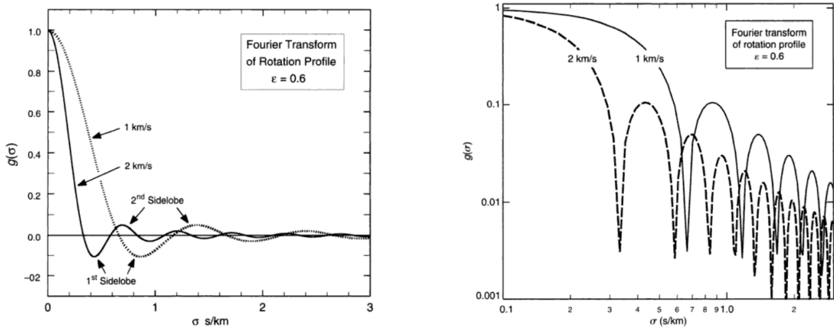
FIGURE 1.2 – Transformée de Fourier d’un profil de raie élargi par rotation, en échelle linéaire (à gauche) et log-log (à droite), pour des vitesses de rotation de 1 et 2 km·s -1 . La largeur spectrale des lobes dépend grandement de la vitesse de rotation. Figures tirées de GRAY (2008).
