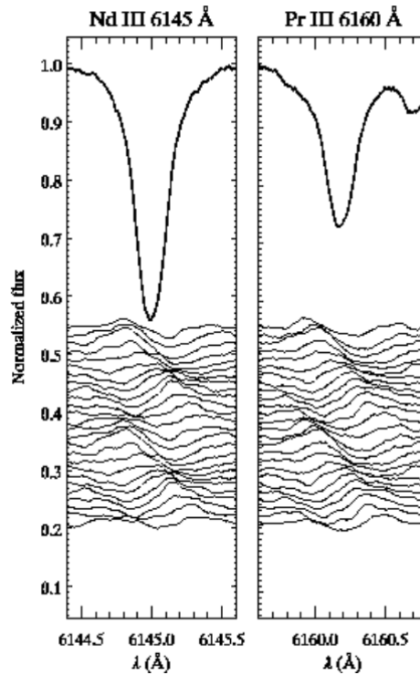
FIGURE 1.8 – Variations du profil de raie causées par une oscillation. Les courbes montrent le profil moyen des raies de NdIII à 6145 Å et PrIII à 6160 Å dans l'étoile \gamma Equ. Les traits plus fins en dessous montrent une série temporelle de la variation à intervalles réguliers, obtenue en soustrayant le profil moyen au profil mesuré à chaque temps. Figure adaptée de KOCHUKHOV et al. (2007).
