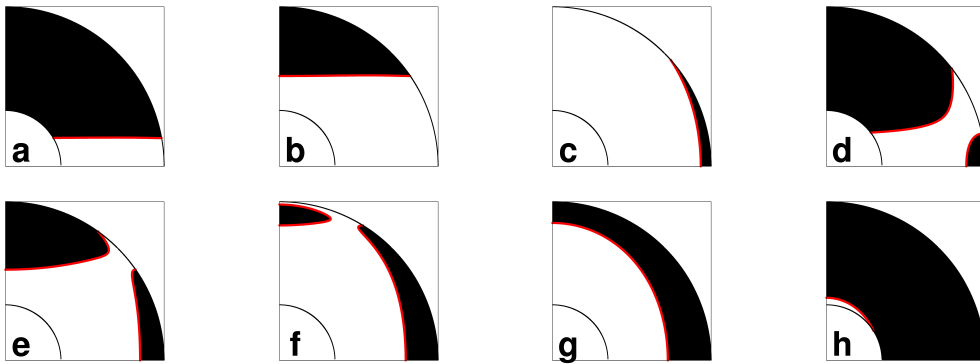
FIGURE 3.1 – Le graphe du haut présente une carte des différentes catégories de modes ax-symétriques dans l'espace de paramètres (N^2, \omega) , pour une coquille de rapport d'aspect \eta = 0,35 . Le domaine jaune contient les modes H (se propageant dans toute la coquille), alors que les aires blanches correspondent aux modes HT (se propageant dans une partie de la coquille seulement, et présentant donc des surfaces de retournement). La zone noircie correspond aux configurations où aucun mode ne se propage. Les courbes pointillées violettes correspondent à l'apparition d'une surface de retournement à r = \eta ou 1, et \sin^2 \theta = 0 ou 1, et délimitent les différentes géométries des domaines de propagation dans la coquille pour les modes HT. Pour chaque sous-domaine, une lettre indique la géométrie présentée dans la miniature correspondante. Dans ces miniatures, le domaine où les ondes peuvent se propager est indiqué en blanc, celui où les ondes sont évanescentes en noir, la ligne rouge correspondant à la surface de retournement \Delta = 0 sur laquelle les caractéristiques se réfléchissent. Au-dessus de la courbe grise, les modes sont potentiellement déstabilisés par l'instabilité ABCD pour \mathcal{P} = 10^{-5} (voir section 3.3 et équation 3.33).
