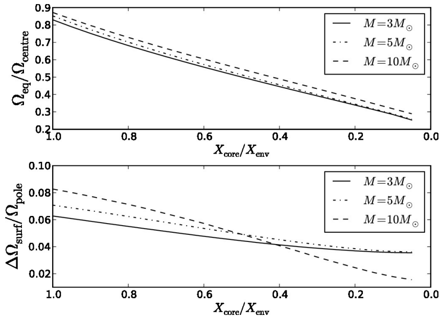
FIGURE 2.2 – Évolution de la rotation différentielle le long de la séquence principale. En haut : rotation différentielle entre centre et surface. En bas : écart entre la rotation maximale et minimale à la surface, rapportée à la rotation du pôle. L’abondance relative d’hydrogène au cœur X_c est un indicateur de l’âge de l’étoile. Résultats obtenus par ESPINOSA LARA et RIEUTORD (2013), à partir de modèles de structure ESTER.
