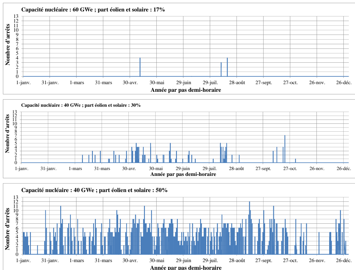
Figure II—39 : Nombre de réacteurs arrêtés à chaque demi-heure de l'année, en fonction de la capacité nucléaire et de la part d'éolien et de solaire
