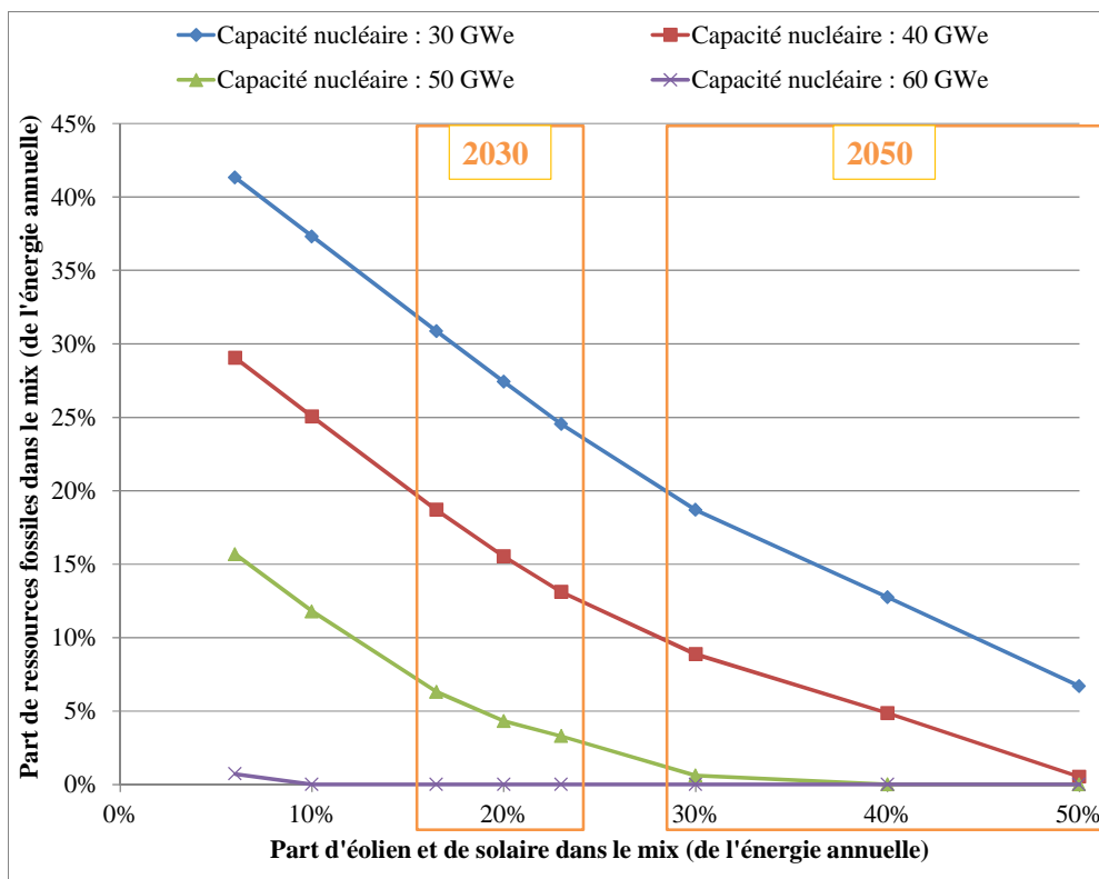
Figure II—22 : Part d'énergie fossile dans la production électrique française en fonction du taux de pénétration de l'éolien, du solaire et des capacités nucléaires installées
