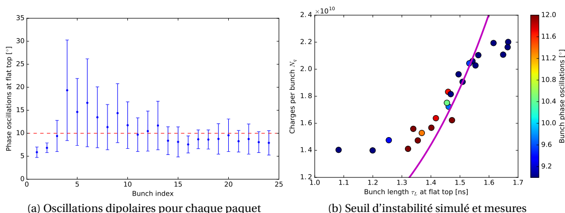
Figure A.6 – Stabilité des paquets d’ions en fonction de leur position le long du faisceau (gauche). Les premiers paquets correspondent à ceux les plus courts et les moins intenses, qui sont ceux les plus instables (droite, accord avec la perte d’amortissement de Landau). Le seuil d’instabilité (magenta) est obtenu en simulations avec le modèle d’impédance du SPS présent.
