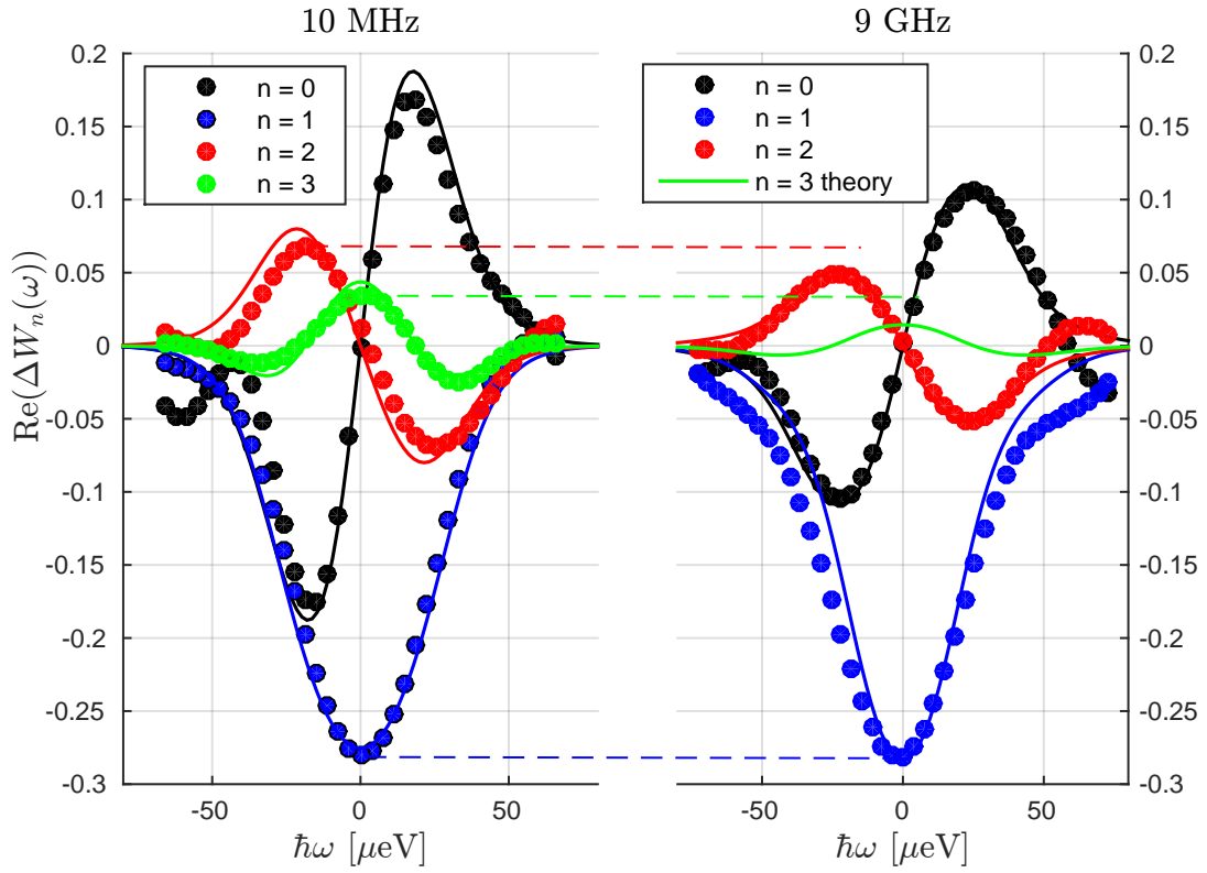
FIGURE 10: Gauche- \text{Re}(\Delta W_n(\omega)) (après déconvolution) pour n de 0 à 3 pour une excitation sinusoïdale à 10 MHz d'amplitude 33 \pm 2 \mu V . Droit- Idem pour une excitation à 9 GHz d'amplitude V_{exc} = 31 \pm 1 \mu V . Les lignes correspondent aux prédictions théoriques. Les lignes horizontales sont des guides pour l'œil qui permettent de comparer les niveaux relatifs des harmoniques. Les poids à n = 1 sont comparables mais on voit qu'il faut en fait plus d'harmoniques pour reconstruire une harmonique basse fréquence que haute fréquence.
