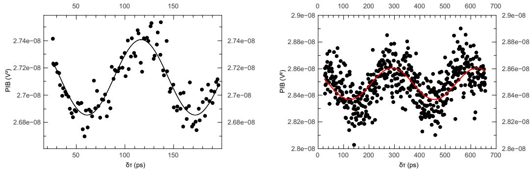
FIGURE 9: Gauche - Bruit intégré sur la bande de mesure avec une excitation en sinus à 9 GHz dans les deux entrées en fonction du déphasage entre ces sinus. Un biais DC de 3,65 \mu\text{V} est appliqué sur l'entrée 2. Cela permet de mesurer à -3,65 \mu\text{eV} l'harmonique à 9 GHz de la fonction de Wigner (soit \Delta\mathcal{W}_{1,1}(-3,65\mu\text{eV}) ) créée par l'excitation sinus à 9 GHz en entrée 1. Droite - Même chose mais avec d'un côté une excitation à 1,75 GHz et de l'autre une excitation à 3,5 GHz et un biais DC à 34 \mu\text{V} . Cela permet de sonder à -34 \mu\text{eV} la deuxième harmonique (à 3,5 GHz) de la fonction de Wigner (soit \Delta\mathcal{W}_{1,2}(-34\mu\text{eV}) ) créée par une excitation sinus à 1,75 GHz.
