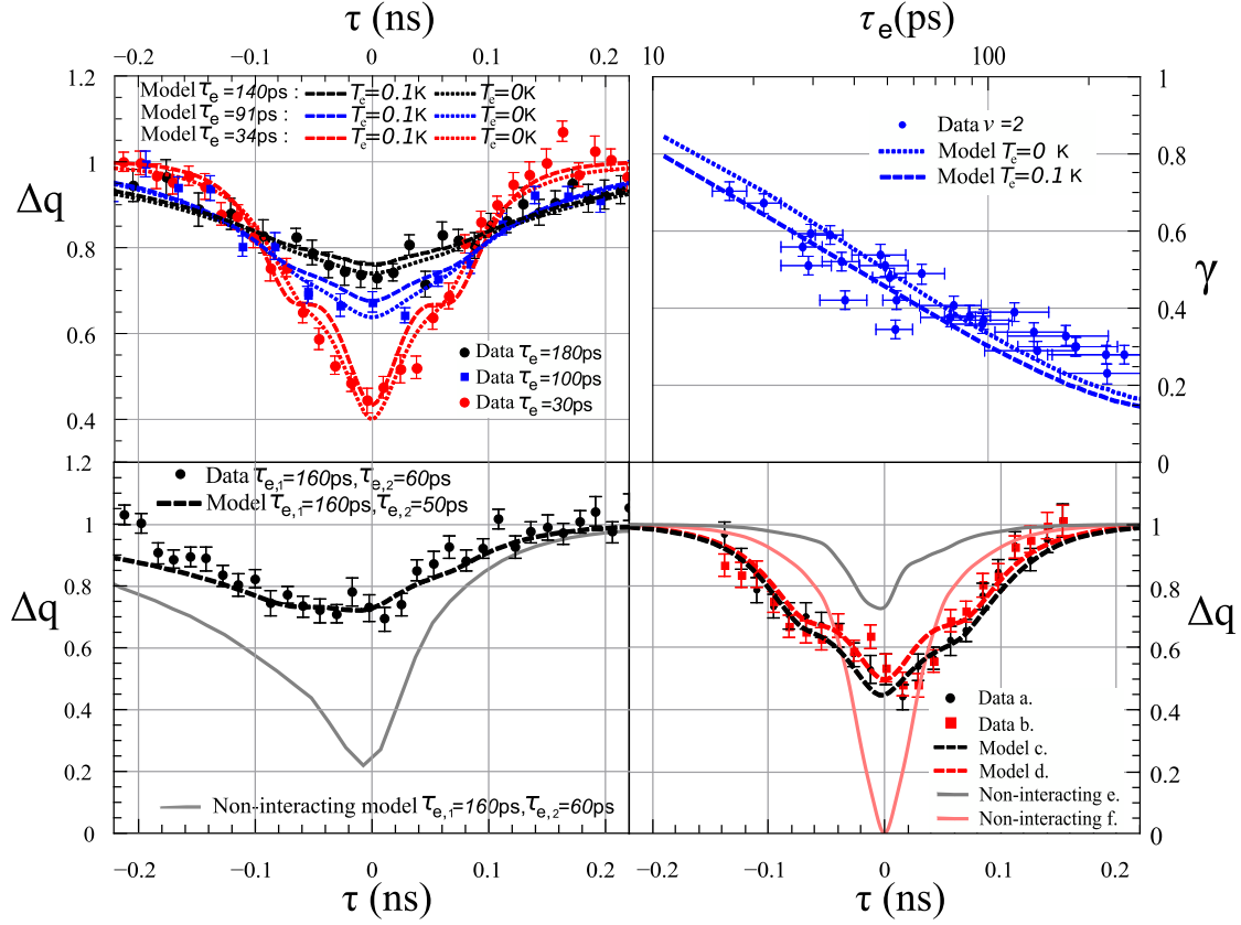
FIGURE 8: Comparaison entre prédictions et mesures à \nu = 2 . Haut-gauche \Delta q(\tau) pour différents temps d'émission \tau_e . La théorie prenant en compte les interactions Coulombiennes est représentée en ligne pointillée ( T = 0 K) et en tirets ( T = 0.1 K). Bas-gauche , \Delta q(\tau) pour des temps de sortie asymétriques. Théorie avec interactions ( T = 0.1 K) en tiret et sans interactions en noir flou. Haut-droit Contraste \gamma en fonction du temps d'émission \tau_e (en échelle log-linéaire). Les pointillés ( T = 0 ) et tirets ( T = 100 mK) représentent les prédictions théoriques avec interactions. Bas-droit (a) mesures, \tau_e = 40 ps, avec un bruit sur l'électrode de la source 2 équivalent à 400 mK; (b) mesures, \tau_e = 40 ps sans bruit rajouté; (c) théorie, T = 0.1 K, \omega_{e1} = 0.7 K, \omega_{e2} = 0.3 K, \tau_e = 40 ps; (d) théorie, T = 0.1 K, \omega_{e1} = \omega_{e2} = 0.7 K; (e) modèle sans interaction, \omega_{e1} = 0.7 K, \omega_{e1} = 0.3 K, \tau_e = 40 ps; (f) modèle sans interactions, \omega_{e1} = \omega_{e2} = 0.7 K, \tau_e = 40 ps.
