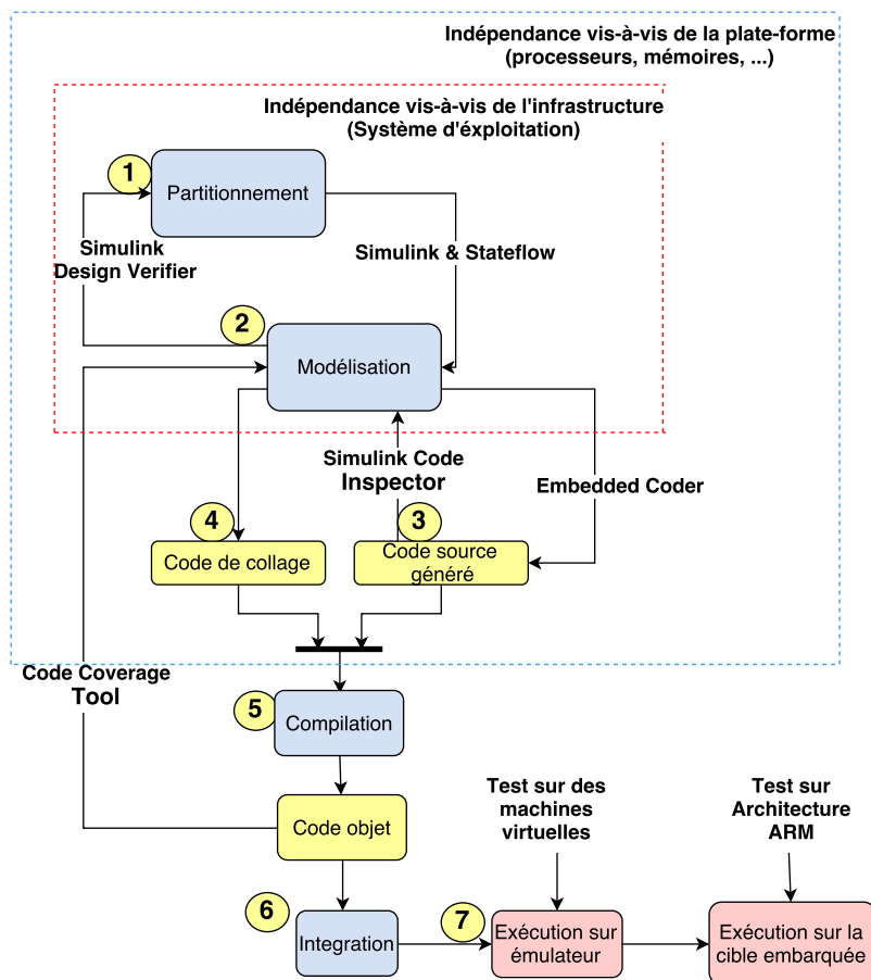
FIGURE 3.2 : Méthodologie de développement orientée modèle pour les systèmes embarqués complexes
