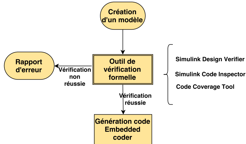
FIGURE 3.3 : Illustration de l'enchainement de la vérification du modèle jusqu'à la génération de code
