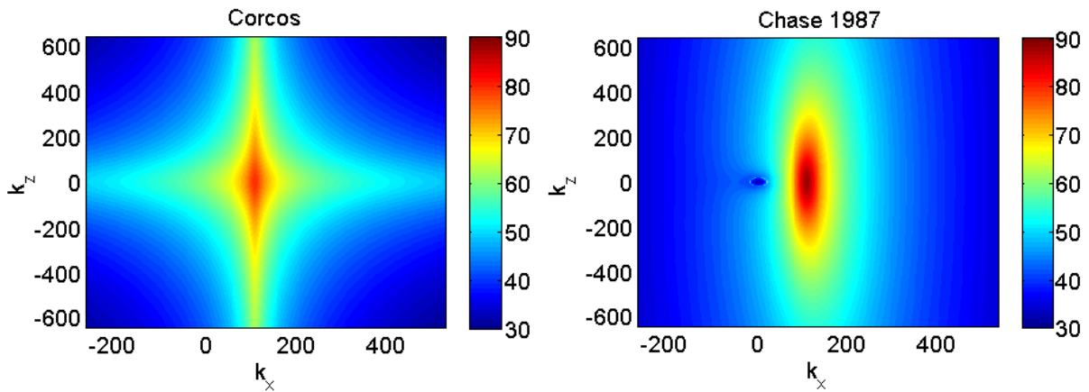
Figure 1.10 : Interspectres \Phi_{pp}(k_x, k_z, \omega) pour f = 1\text{kHz} ( \text{dB} , ref 1\mu\text{Pa}^2\text{m}^2/\text{Hz} ). Comparaison des modèles de Corcos et de Chase.
