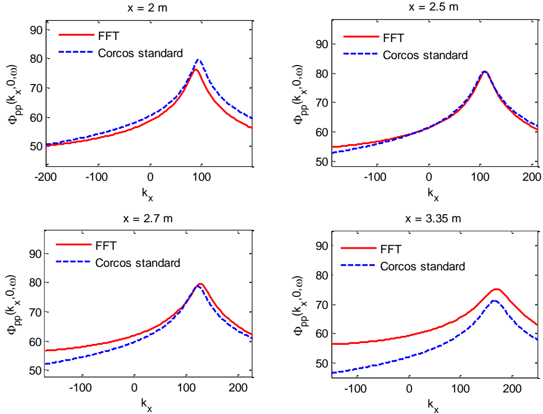
Figure 2.21 : Interspectres en nombre d'onde (dB ref 1\mu Pa^2 m^2 / Hz ) pour les positions en gradient adverse à f = 1 \text{ kHz} . Comparaison entre les spectres issus de la TF spatiale des mesures approchées, et les spectres calculés par le modèle de Corcos en nombre d'onde à partir des paramètres standards (modèle de Smol'yakov pour U_c , et \alpha_x = 0.11 , \alpha_z = 0.77 ).
