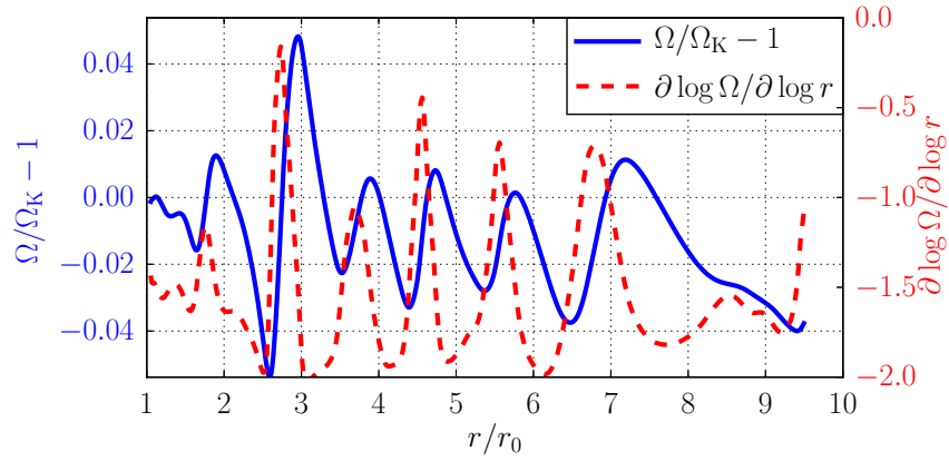
FIGURE VIII.27. – Profils radiaux dans le run 'R1 – P2', moyennés sur la hauteur du disque entre 500T_0 et 70T_0 : déviations au profil de rotation képlérienne ( trait bleu ) et cisaillement adimensionné ( tirets rouges ).
