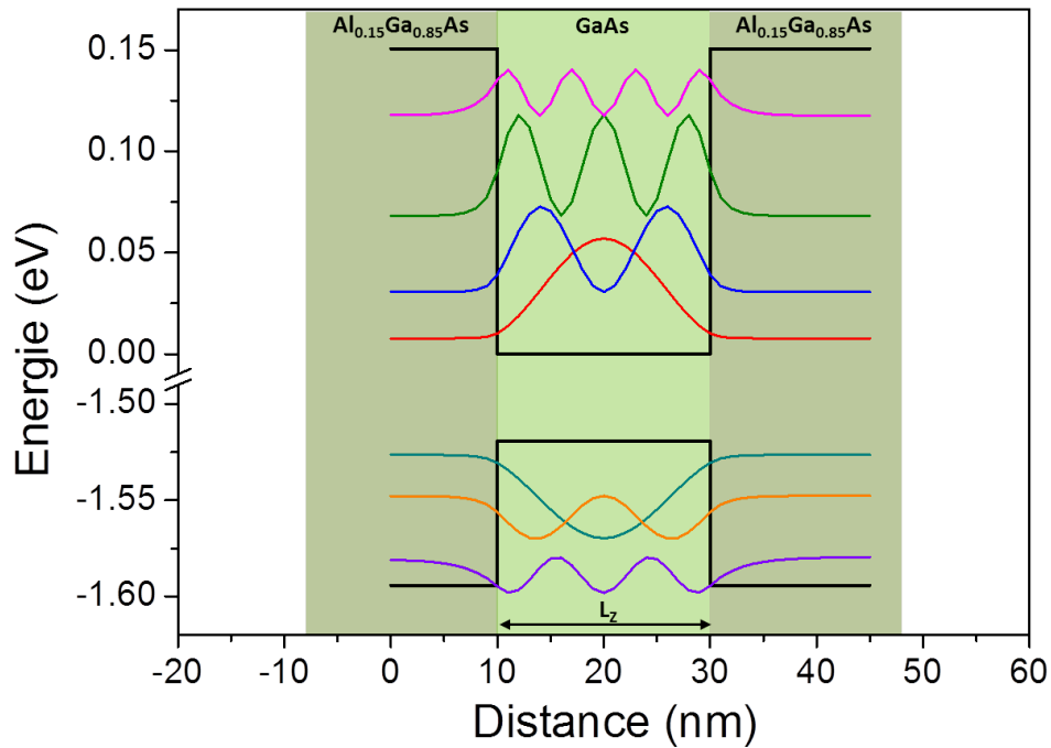
FIGURE I.2 – Modules au carré des fonctions d'onde des états confinés dans la bande de conduction et dans la bande de valence (trous légers) d'un puits quantique GaAs/Al_{0.15}Ga_{0.85}As de taille L_z .
