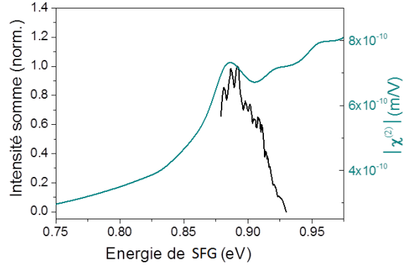
FIGURE V.36 – Intensité de la SFG en fonction de l'énergie de la SFG pour le LCQ MIR basé sur InP à 250 K. Comparée au module de \chi^{(2)} calculé.
