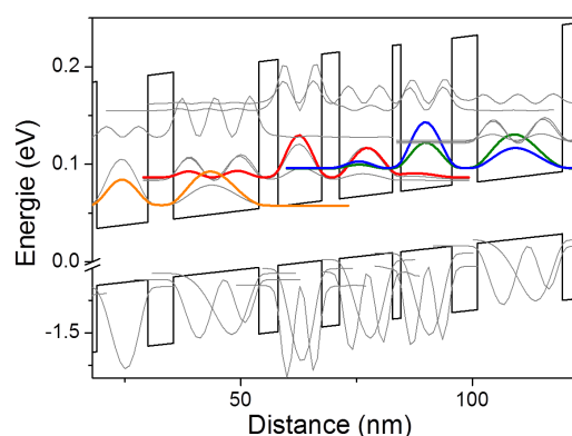
FIGURE VI.9 – Structure de bandes du LCQ THz L773, électrons et trous lourds.
