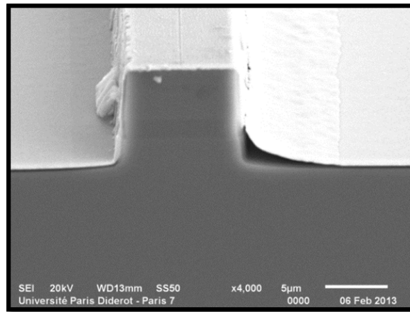
FIGURE IV.8 – Exemple de photo au microscope électronique du LCQ MIR basé sur GaAs, après process.
