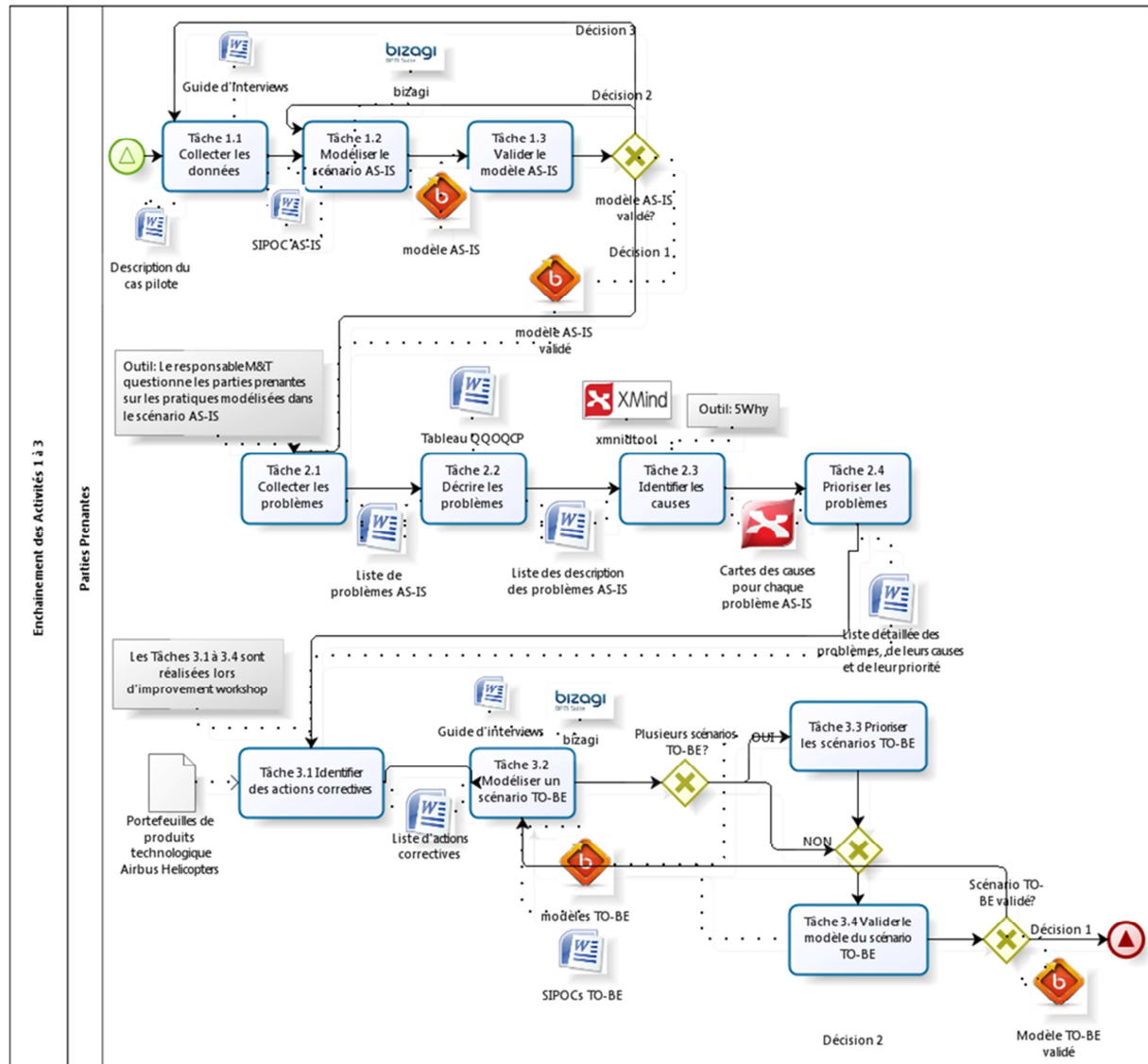
Figure 74: Modèle de l'enchaînement des tâches des Activités A1 à A3
