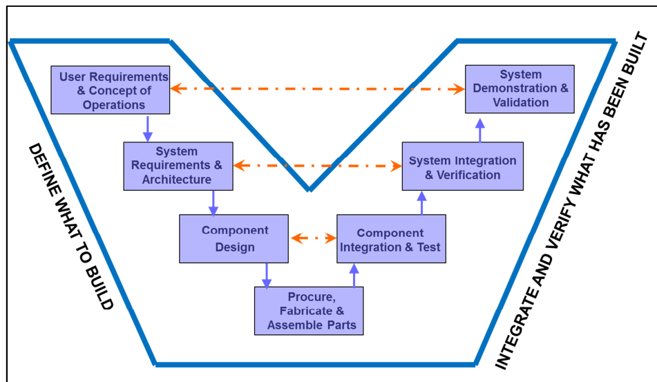
Figure 22: Processus d'ingénierie système (Sauser et al. 2010)
