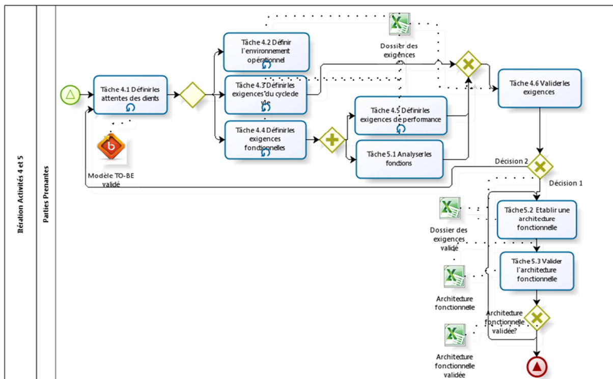
Figure 77 : Modèle des activités 4&5- Analyser les exigences et définir l'architecture fonctionnelle
