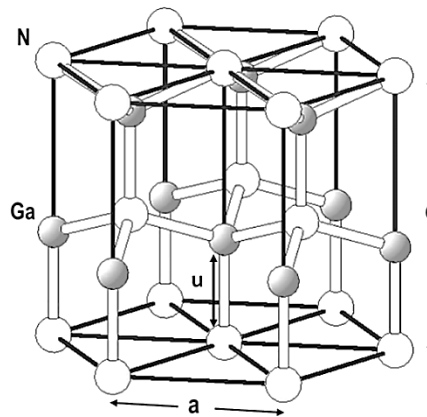
Figure 1.4: Wurtzite lattice parameter a , c and u for GaN.
