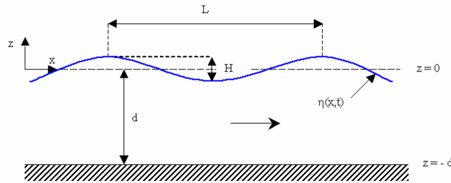
Figure 1 Notations de la houle
