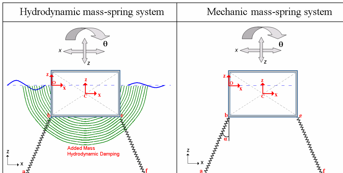
Figure 5 Représentation hydrodynamique et mécanique d'un système mass-ressort
