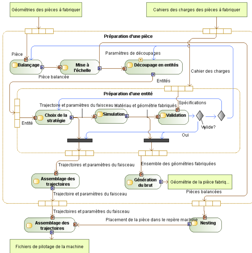
FIGURE 2.2.2 – Proposition de processus de FAO
