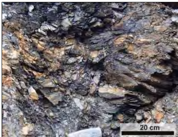
Figure I-38 : Schistes ampéliteux.
