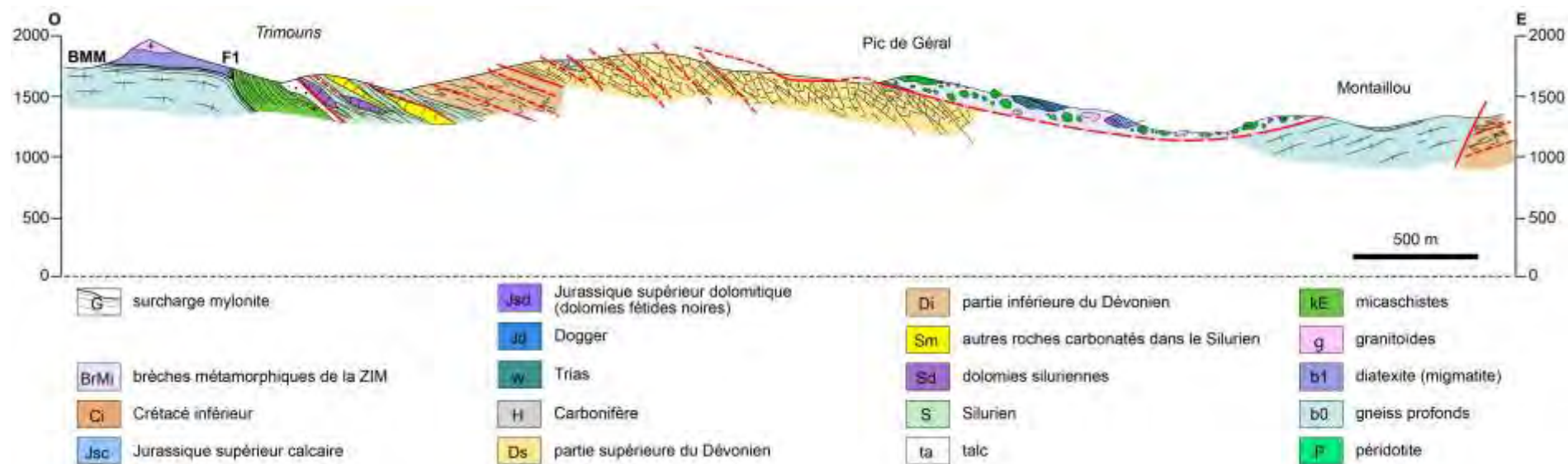
Figure II-43 : Coupe large 2 ; Trimouns - Montaillou.
