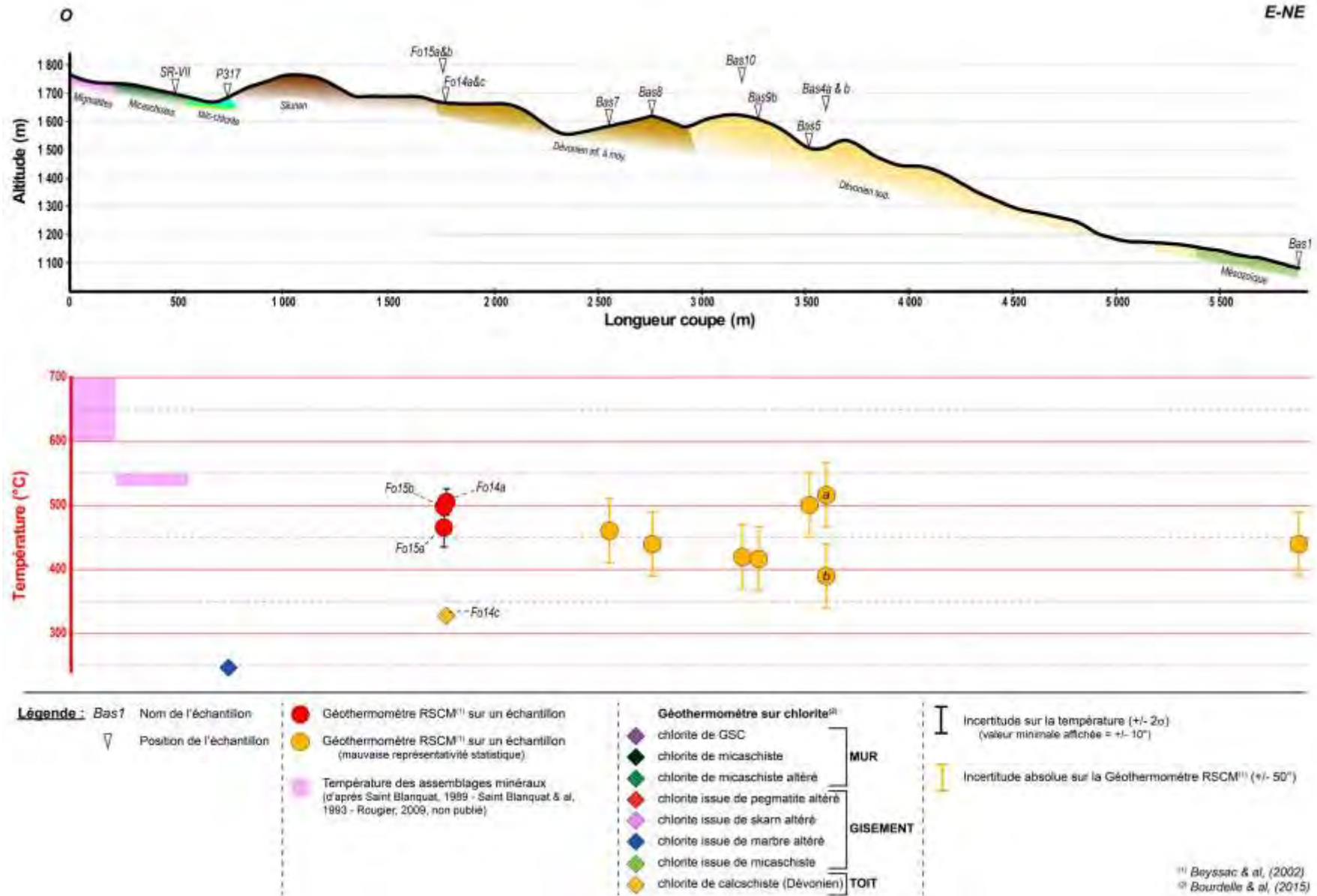
Figure III-28 : Coupe thermique Trimouns-Basque.
