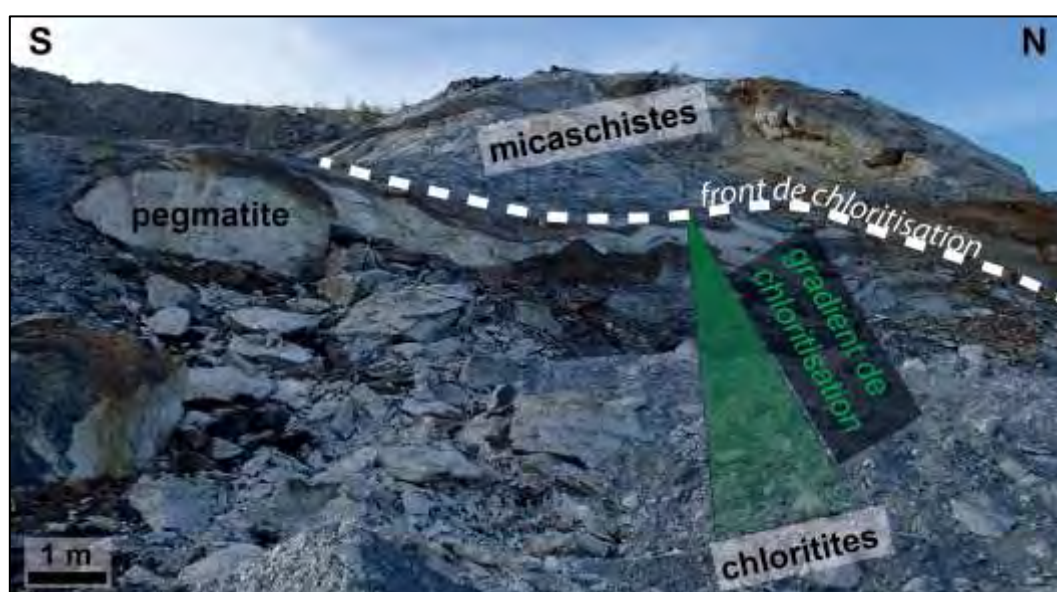
Figure I-21 : Vue des micaschistes chloritisés/gradient de chloritisation.
