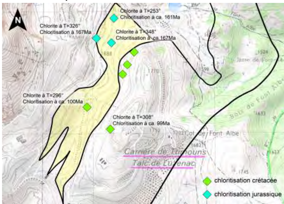
Figure V-3 : Carte des échantillons de chlorites dont la température et la date de minéralisation ont été estimées (gisement en jaune).
