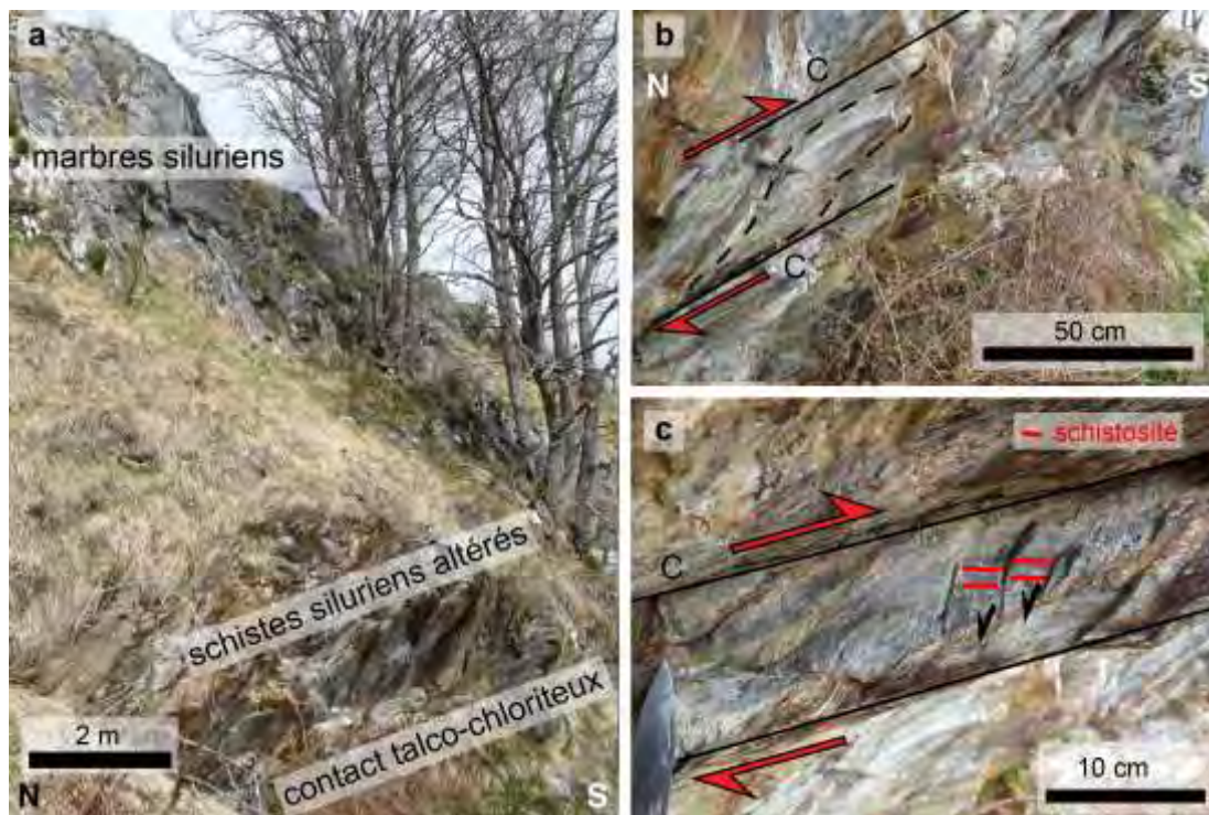
Figure II-32 : Accident talco-chloriteux à la boutonnière de Causou ; (a) en vue globale, (b) détail de la cinématique du bloc supérieur vers le sud ; et (c) zoom sur les microfailles antithétiques.
