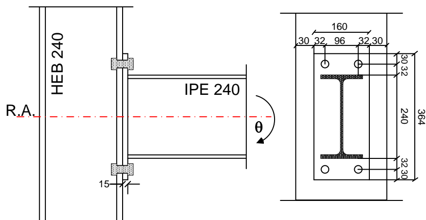
Figure 6.4: Configuration de l'assemblage traité
