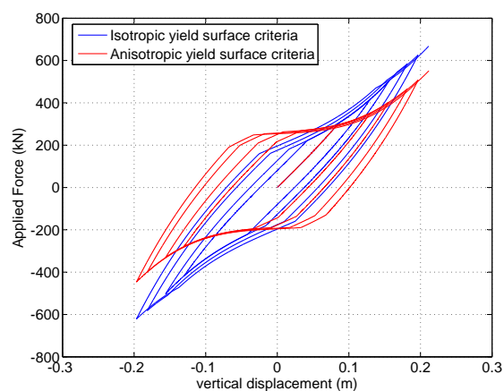
(d) q=4 - Déplacements imposés
