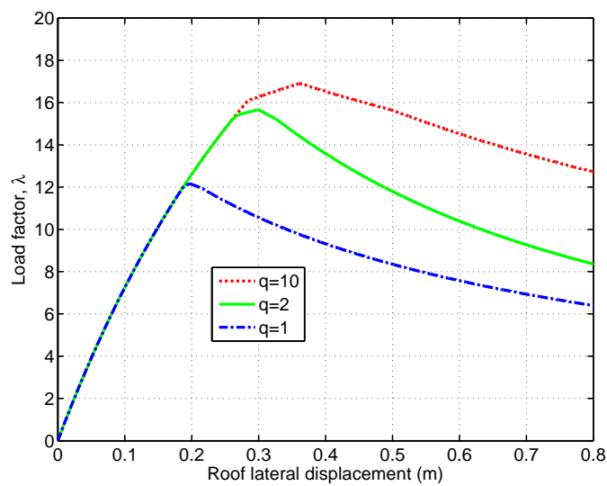
Figure 6.26: Influence du facteur q sur le niveau maximum de chargement atteint \lambda .
