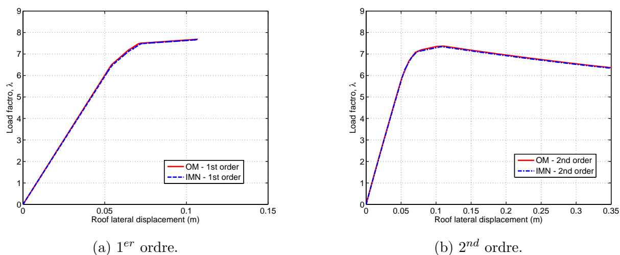
Figure 6.21: Facteur de force \lambda - déplacement latéral
