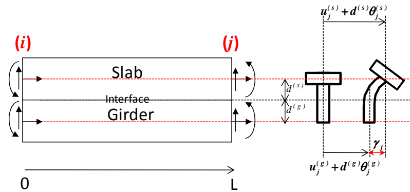
(a) Contact au nœud (i) et (j).
