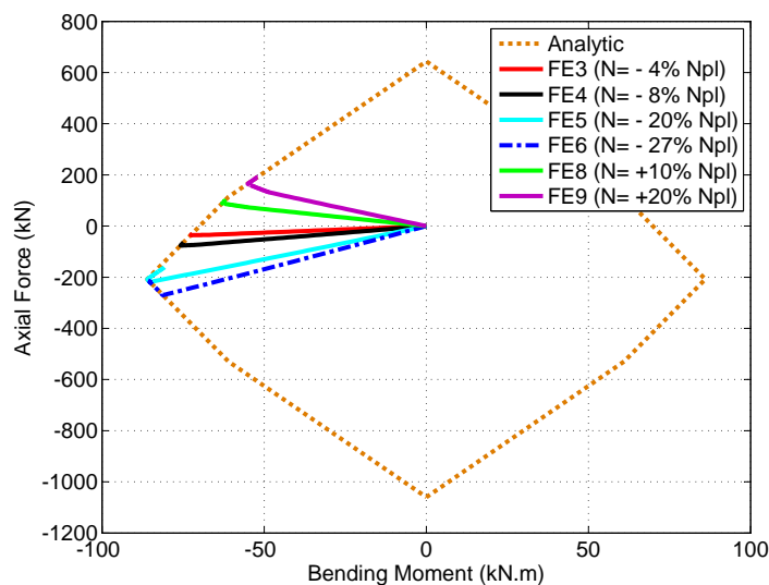
Figure 6.12: Diagramme d'interaction
