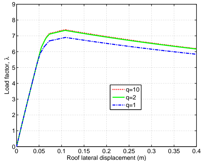
Figure 6.22: Influence du facteur q sur le niveau maximum de chargement atteint \lambda .
