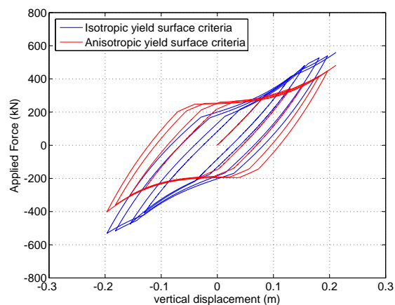
(b) q=2 - Déplacements imposés
