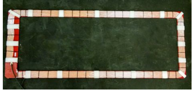
Fig. 11: Bobine de l'émetteur fixée sur la base de fibre de verre avec du ruban de tissu blanc et des bandes de plastique (en noir).
