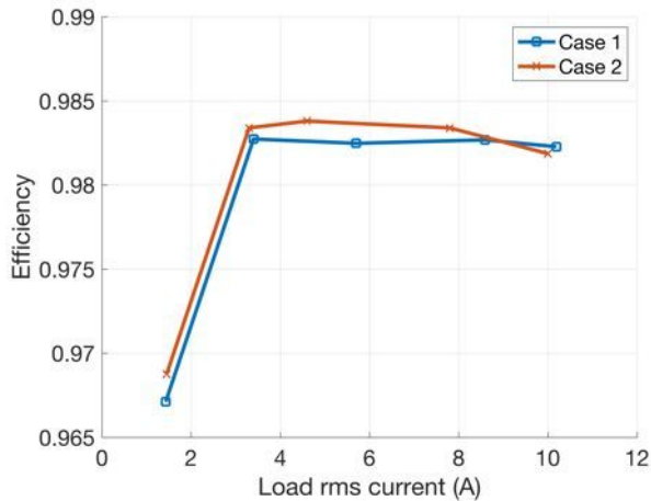
Fig. 8: Efficacité mesurée avec la méthode de l'opposition. Cas 1: IGBT turn-on en premier. Cas 2: SiC MOSFET tun-on en premier.
