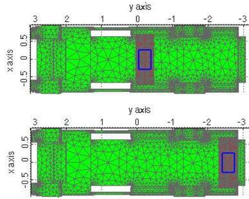
Fig. 19: Position analysée pour le montage de la structure du récepteur. Structure du récepteur en rouge. Bobine du récepteur en bleu.
