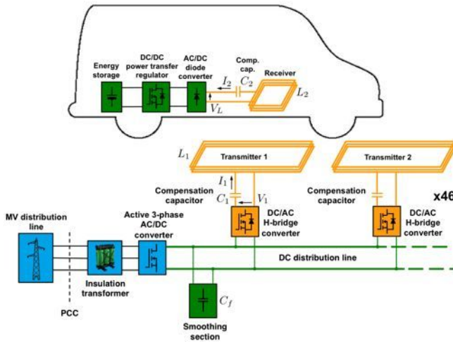
Fig. 15: Schéma de l'architecture générale du système IPT développé pour le prototype routier.
