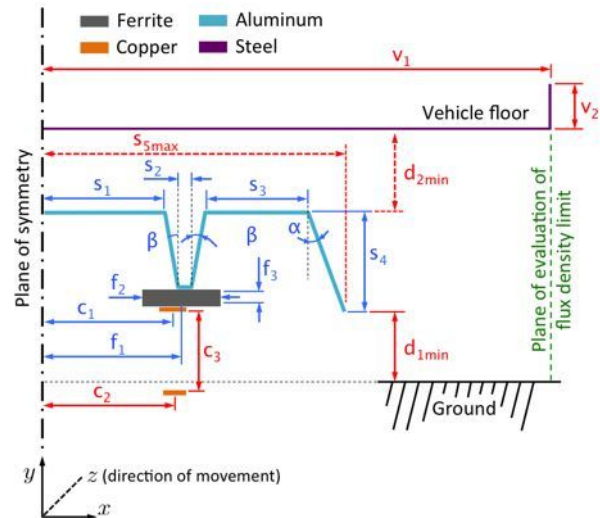
Fig. 10: Schéma de la géométrie à optimiser. Les variables d'optimisation en bleu. Paramètres fixes en rouge. Contraintes d'optimisation en rouge pointillé.
