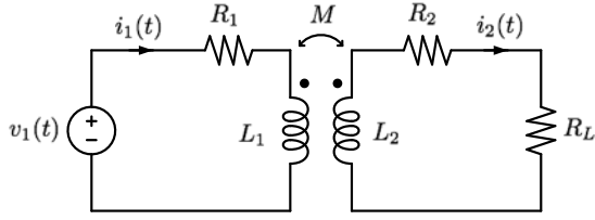
Fig. 3: Représentation de circuit du système.
