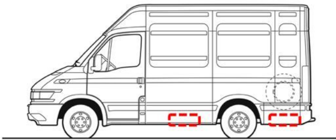
Fig. 9: Positions autorisées pour le montage de la structure du récepteur sans modification du châssis du véhicule.
