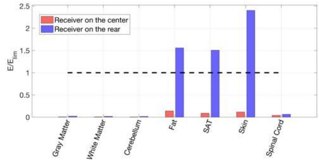
Fig. 21: Indice d'exposition sur les tissus target pour les cas pires analysés. Cas 1 en rouge et Cas 2 en bleu.
