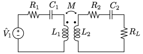
Fig. 4: Représentation de circuit du système avec les condensateurs de compensation.
