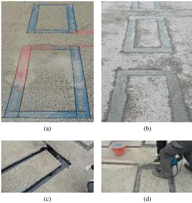
Fig. 17: Description du processus d'intégration. Coupe des bordures des trous (a). Creusement du trou dans l'asphalte routier (d). Remplissage du matériau de séparation entre la bobine et le sol (c). Dernière couche de béton (b).
