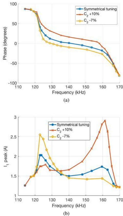
Fig. 6: Comportement du système par rapport à la fréquence d'alimentation pour différentes conditions de réglage du condensateur connecté au récepteur. La phase du courant de l'émetteur est montrée en (a) et le pic en (b).
