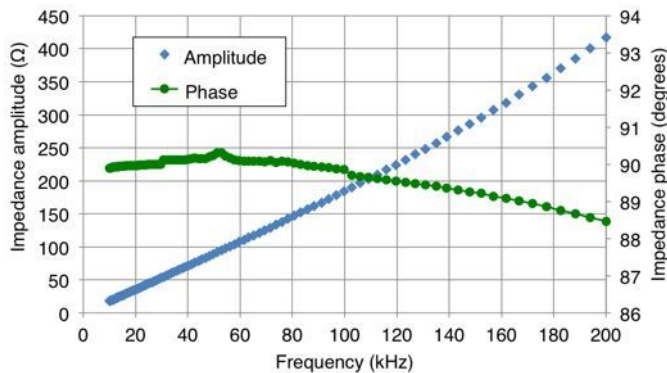
Fig. 18: Mesure d'amplitude et de phase de l'impédance de la bobine installée avec la méthode développée.
