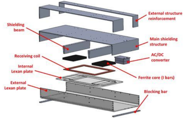
Fig. 12: Modèle CAO des principaux composants de la structure du récepteur.
