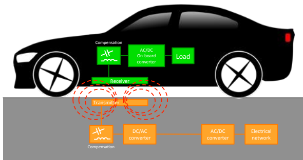
Fig. 1: Schéma générales des composantes d'un système IPT pour véhicules électriques.
