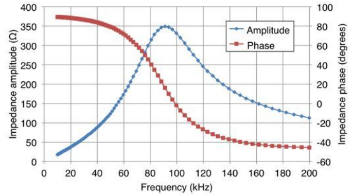
Fig. 16: Amplitude et phase de l'impédance d'un émetteur placé directement sur le pavé routier.
