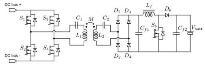
Fig. 7: Schéma fonctionnel de l'architecture globale du système IPT.
