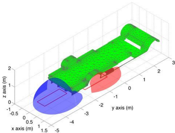
Fig. 20: Surfaces à la valeur limite de 27 \mu\text{T} de densité de champ magnétique dans le cas pires. Les deux cas sont représentés avec la relative position des bobines. Le volume rouge se réfère au cas 1 avec le récepteur monté sur le centre. Le volume bleu se réfère au cas 2 avec le récepteur monté à l'arrière.
