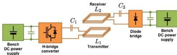
Fig. 5: Configuration pour tester le comportement en fréquence.
