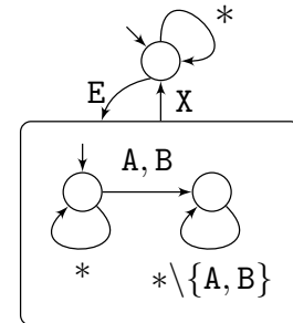
Figure 6.3 – HFA déplié.
