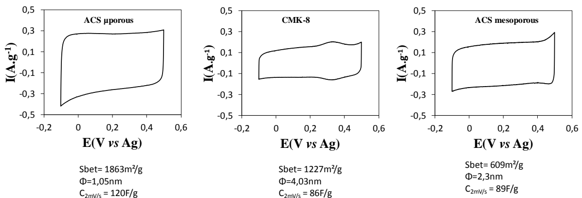
Figure 9 : Voltammogrammes cycliques des carbones ACS \mu porous CMK-8 et ACS mesoporous dans \text{H}_2\text{SO}_4 1 M enregistrés à 2 \text{ mV}.\text{s}^{-1}
