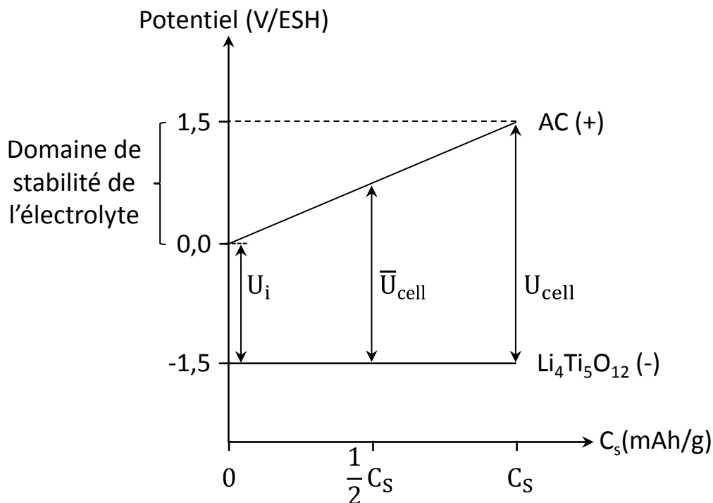
Figure 8: Principe de fonctionnement d'un système hybride
