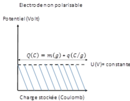
Figure 4 : Comportement d'une électrode non polarisable
