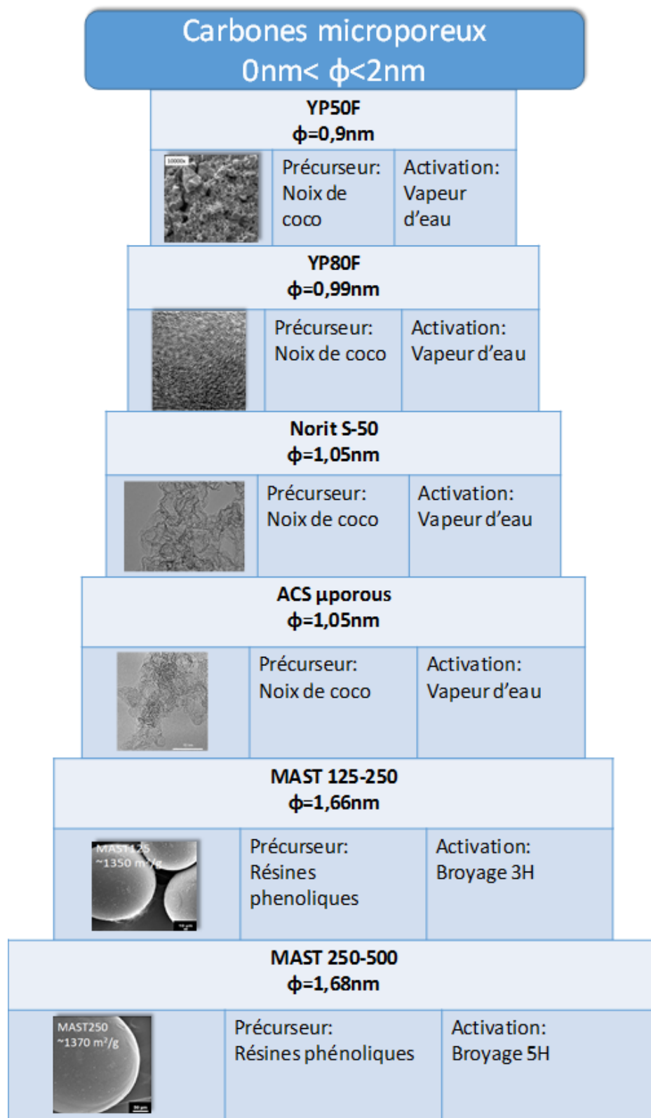
Figure 4 : Présentation des différents carbones microporeux
