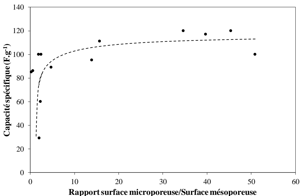
Figure 19 : Evolution de la capacité spécifique avec le rapport entre la surface microporeuse et la surface mésoporeuse
