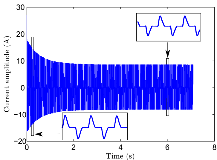
FIGURE 3.1 – Courant de mise en marche d'un aspirateur.
