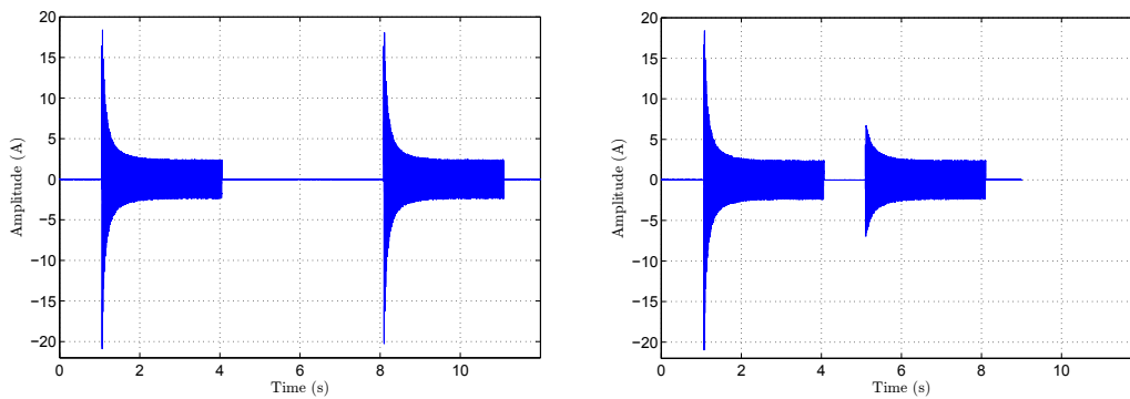
(a) Démarrages successifs lents d'une perceuse
