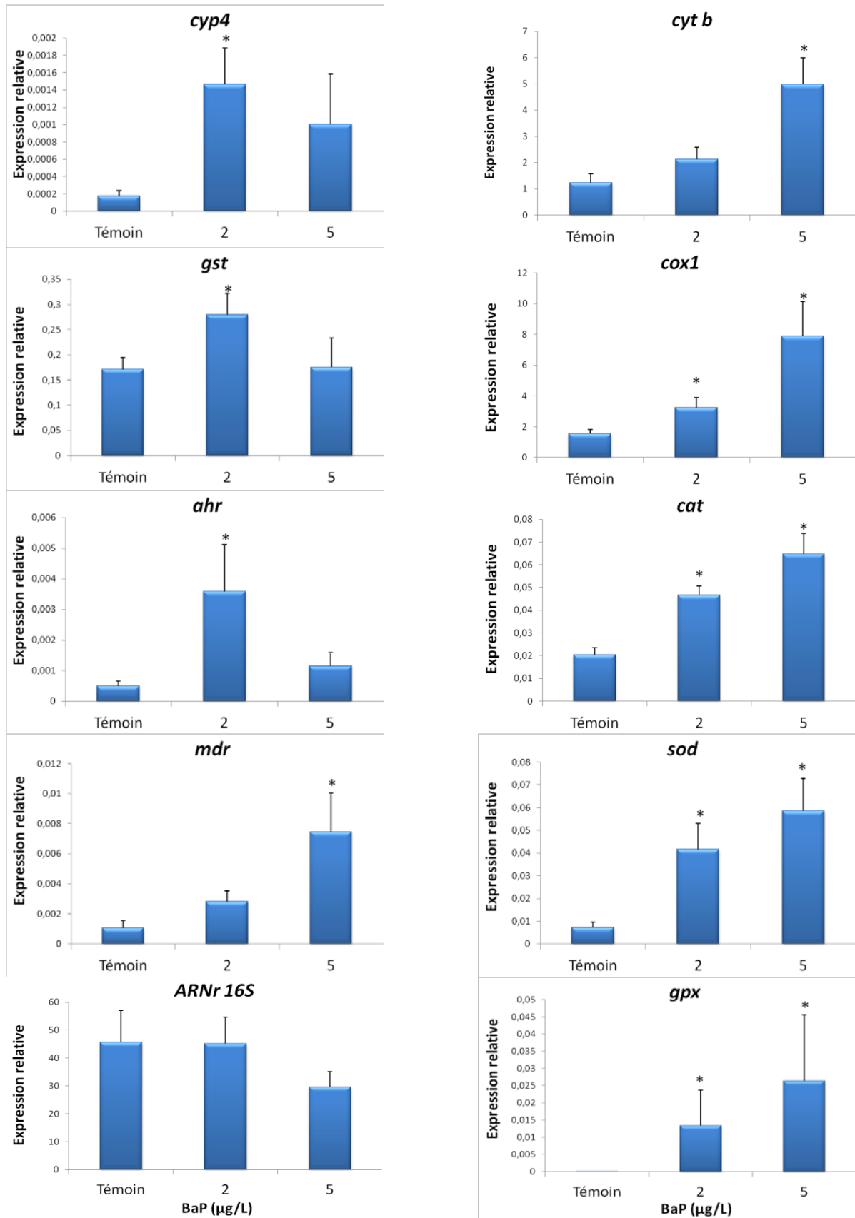
Figure 43 : Expressions génétiques relatives des 10 gènes étudiés au niveau des branchiae de R. philippinarum exposée pendant 7 jours à des concentrations subaiguës de BaP. Les résultats sont exprimés en moyenne \pm SEM ( n = 5 ). * indique une différence significative comparée au témoin selon ANOVA sur rangs et le test de Tukey, p < 0,05 .
