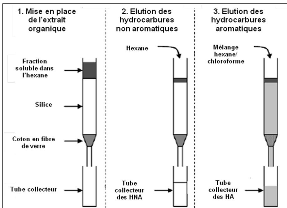
Figure 24 : Représentation schématique du fractionnement par chromatographie en Phase liquide (CPL).
