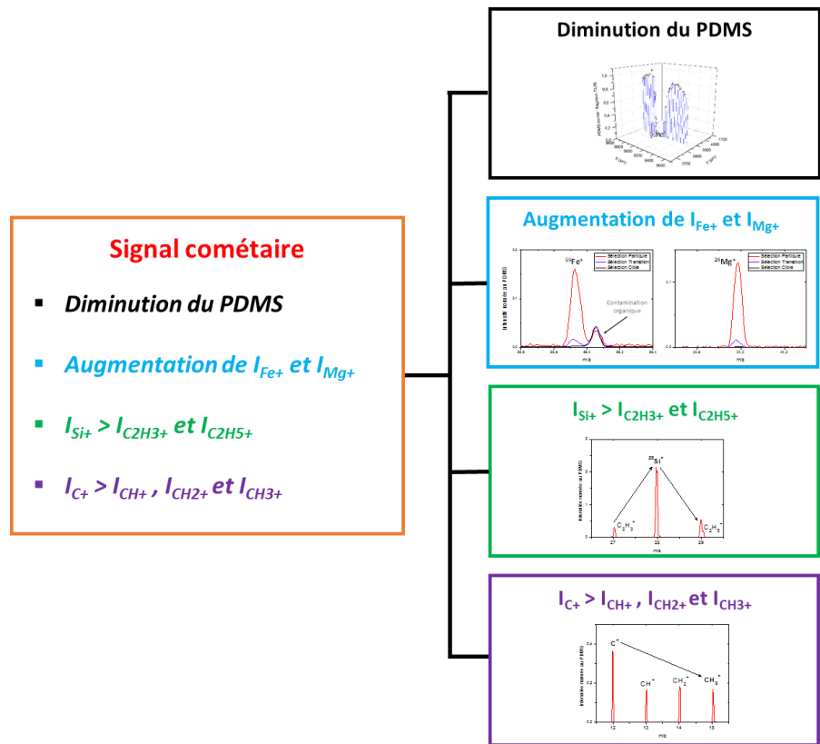
Figure 85 : Organigramme synthétisant les différentes étapes de la méthodologie de l'analyse des spectres de masse d'ions secondaires positifs acquis par l'instrument COSIMA XM. « I » représente l'intensité du signal des ions secondaires.
