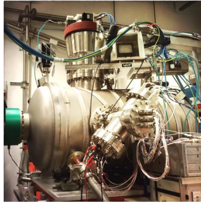
Modèle de référence COSIMA RM Au MPS Göttingen, Allemagne
