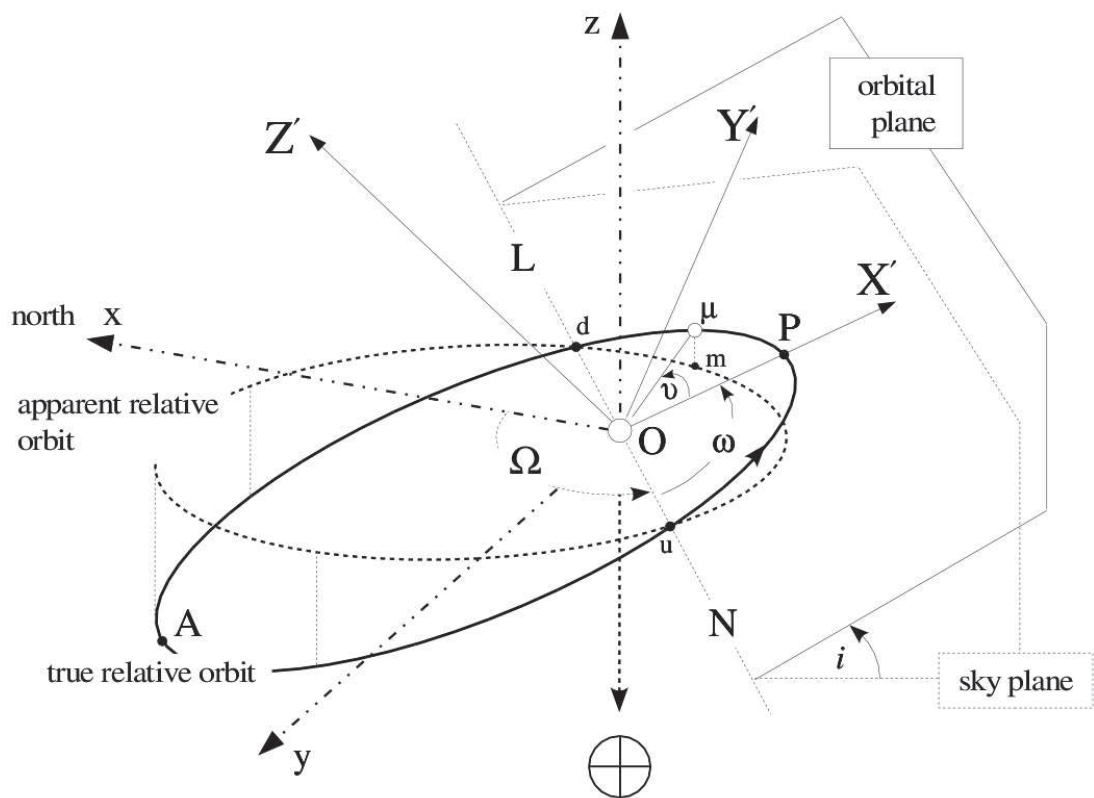
FIG. 41 – Schéma de la description des paramètres orbitaux pour un système double.
