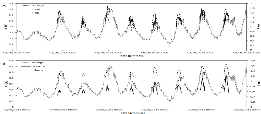
FIGURE V.10 – Zuydcoote, hauteur de houle au large et hauteur d'eau au niveau de A) ADCP B2 B) ADCP bache.
