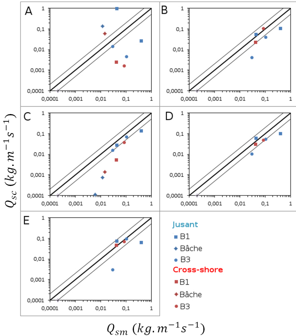
FIGURE VI.13 – Débit solide calculé en kg.m^{-1}.s^{-1} en fonction du débit solide mesuré en kg.m^{-1}.s^{-1} avec la formule de Kamphuis avec en rouge les mesures cross-shore et en bleu les mesures longshore, pour : A) \gamma = 0.25 , B) \gamma = 0.40 , C) \gamma = 0.42 avec la formule de Thornton et Guza, D) \gamma = 0.55 , E) \gamma = 0.78
