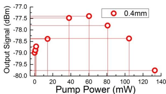
Fig. 13 : Evolution du niveau de signal ( \lambda=1550 nm) en sortie du guide SiN slot de la Fig. 10 en fonction de la puissance de pompe ( \lambda=1480 nm).
