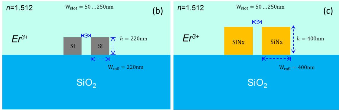
Fig. 8 : Vues de principe des configurations étudiées en vue de la réalisation d'amplificateurs à guides dopés Erbium en photonique sur silicium : familles de guides Si/SiO 2 et SiN/SiO 2 .
