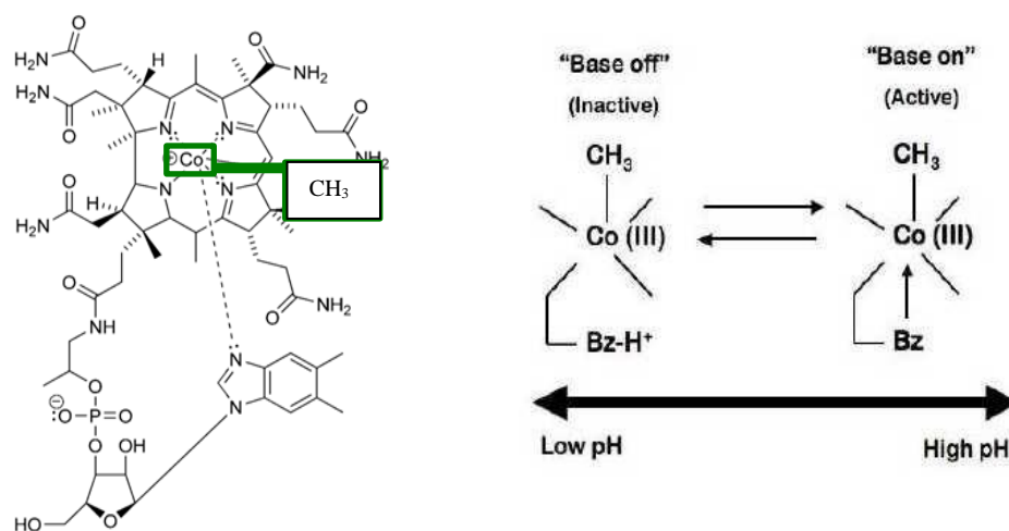
Figura 13 : Reacción de metilación del \text{Hg}^{2+} por la metilcobalamina ( \text{MeCo} , \text{CH}_3\text{B}_{12} ), estructura molecular y cambios de conformación de la MeCo en función del pH.
