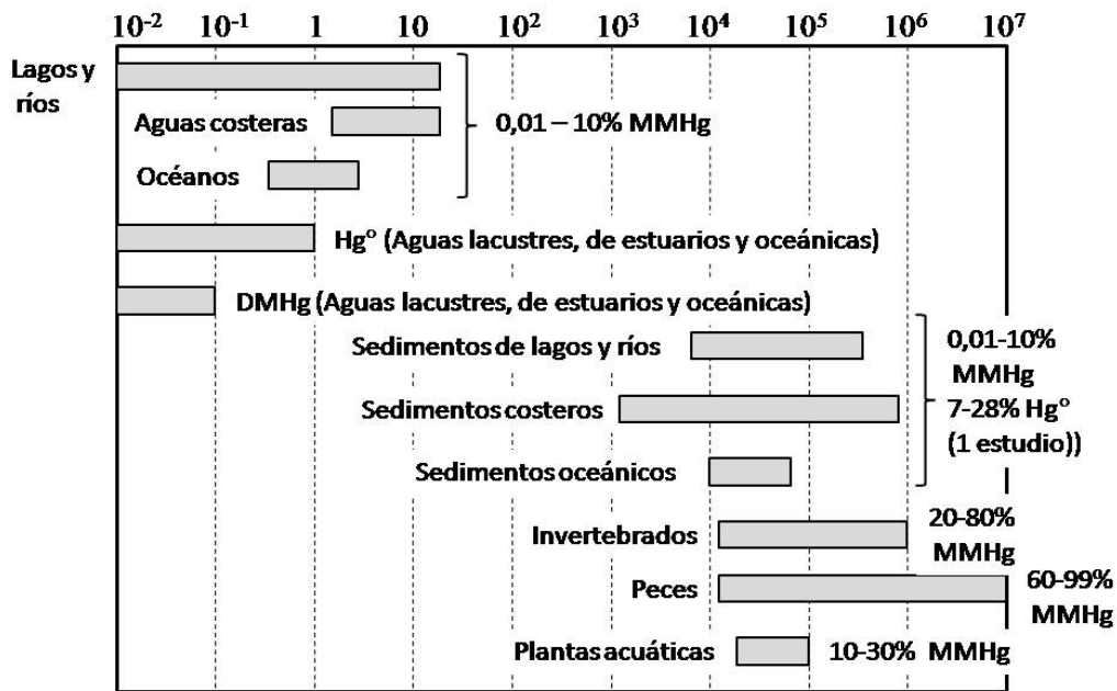
Figura 15 : Gama de concentraciones de Hg_T salvo mención contraria ( ng L^{-1} o ng Kg^{-1} de peso fresco) en el medio ambiente y proporciones de Hg orgánico (Tessier, 2004; Fitzgerald and Lamborg, 2003, Bouffard and Amyot, 2009).
