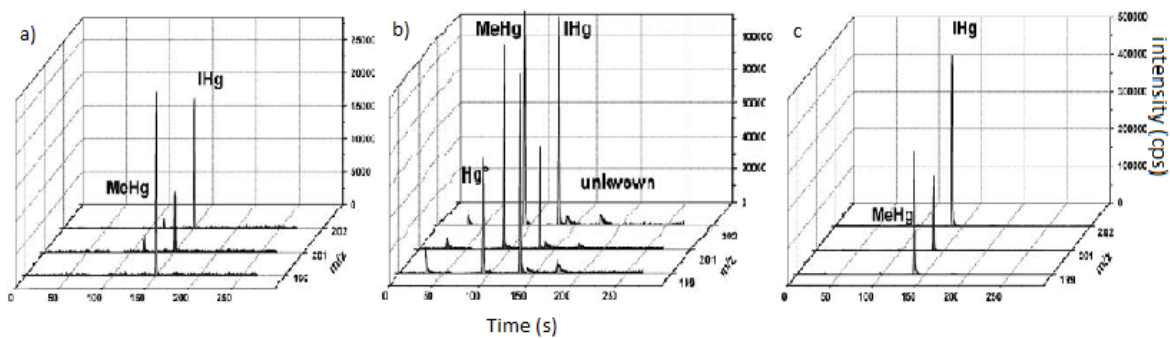
Figura 22 : Cromatogramas GC-ICPMS para la especiación de Hg después del doble dopaje con ^{199}\text{IHg} and ^{201}\text{MMHg} y etilación/propilación derivatización en (a) agua de mar (WI), (b) tejido de ostra (CRM 710), (c) sedimentos de estuario (IAEA 405) Monperrus et al., 2008.
