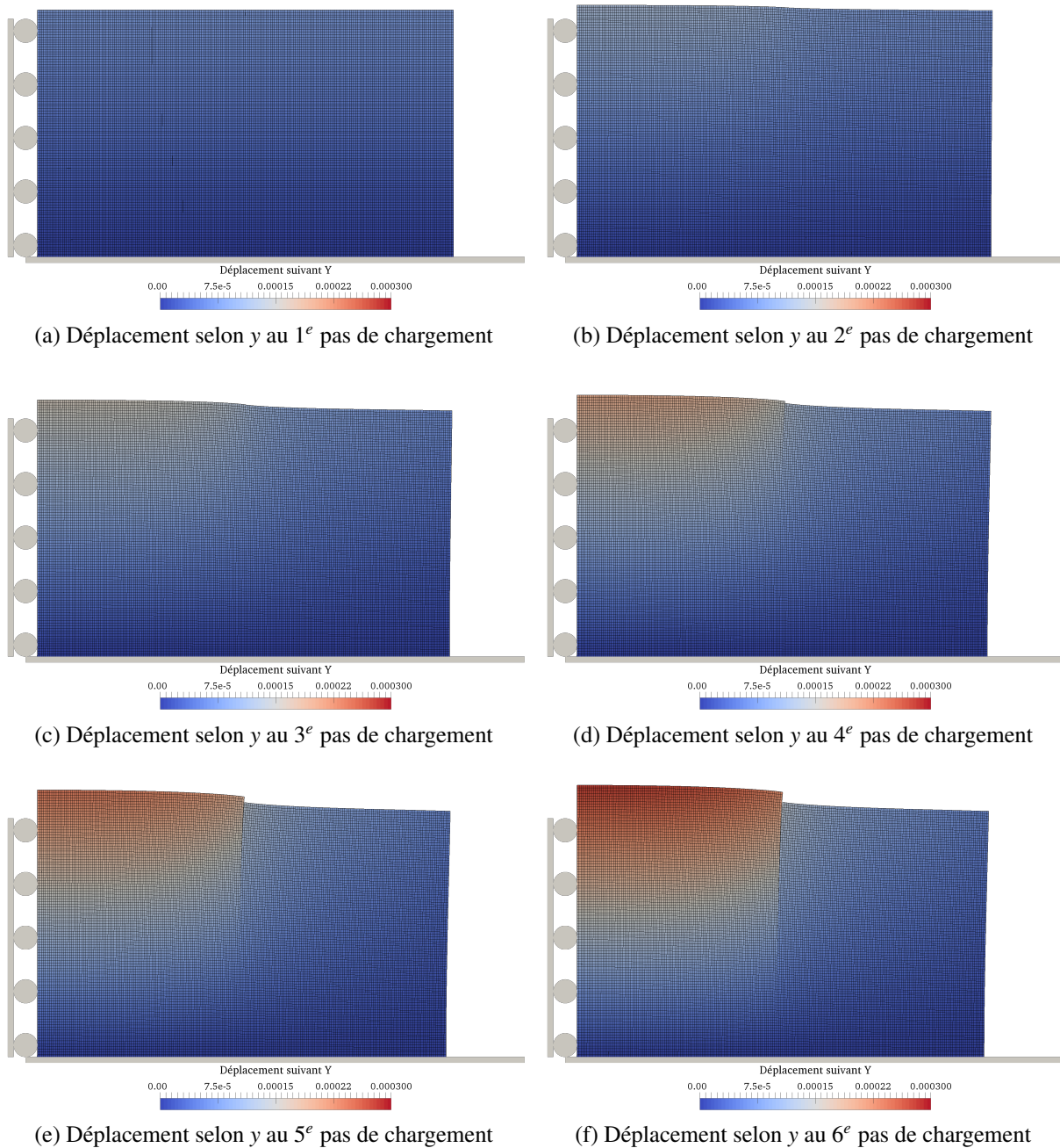
FIGURE 4.4 – Déformée ( \times 500 )
