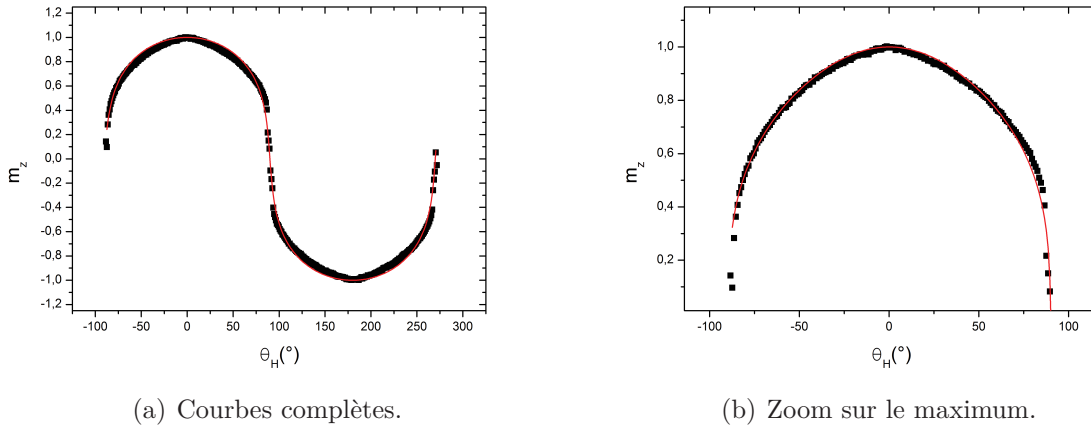
Figure IV.5 – Courbes de résistance de Hall normalisée en fonction de l’angle \theta_H entre la direction d’anisotropie magnétique facile, perpendiculaire au plan des couches minces, et la direction du champ magnétique appliqué. Les carrés noirs sont les points expérimentaux, et la ligne rouge représente la résistance normalisée calculée. Le champ magnétique constant est de +1955 Oe.
