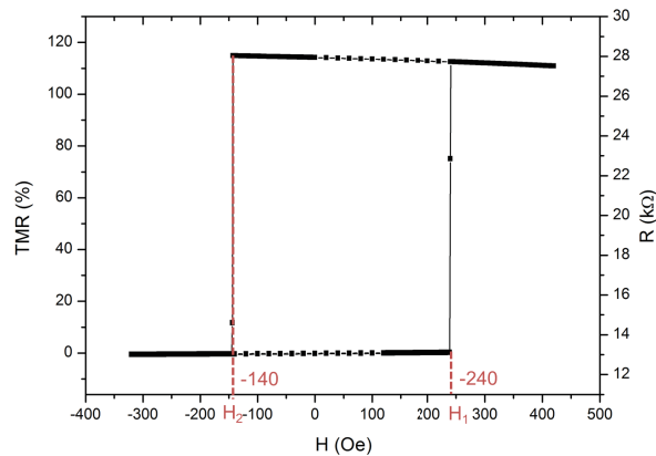
Figure II.9 – Courbe d'hystérésis mineure de la couche douce composée de 1,1 nm de CoFeB de l'empilement 8 \text{ Ta}/1,1 \text{ Co}_{40}\text{Fe}_{40}\text{B}_{20}/1,87 \text{ MgO}/1,5 \text{ Co}_{60}\text{Fe}_{20}\text{B}_{20}/0,4 \text{ Ta}/0,8 \text{ Co}/0,55 \text{ Pt}/5 \times [0,3 \text{ Co}/0,55 \text{ Pt}]/0,6 \text{ Co}/0,9 \text{ Ru}/0,6 \text{ Co}/0,55 \text{ Pt}/13 \times [0,3 \text{ Co}/0,55 \text{ Pt}]/5 \text{ Ta}/5 \text{ Ru} .
