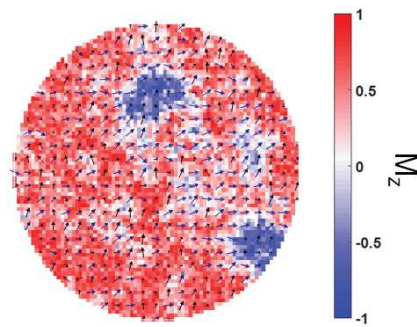
Figure III.12 – Cartographie de l'aimantation suivant e_z du plot magnétique issue des simulations numériques à 300 K en prenant \alpha = 0,1
