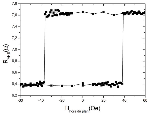
Figure II.13 – Cycle d’hystérésis du CoFeB de l’empilement 8\text{ Ta}/1,1\text{ Co}_{40}\text{Fe}_{40}\text{B}_{20}/\text{MgO}/5\text{ Ta}/5\text{ Ru} mesuré par effet Hall anomal avec une tension appliquée sur la barrière tunnel de 0,01\text{ V} .
