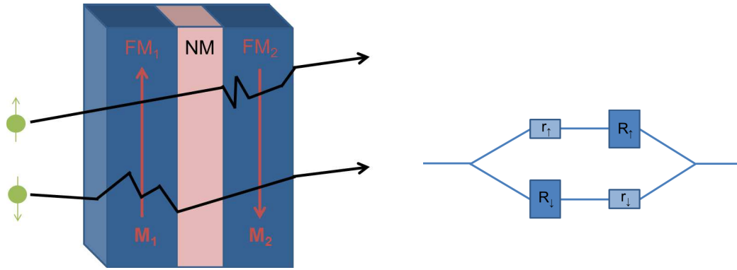
(a) Schéma du parcours des électrons dans la tricouche FM1/NM/FM2. Les cercles verts surmontés d'une flèche correspondent aux électrons avec leur spin et les courbes noires au parcours schématique des électrons.
