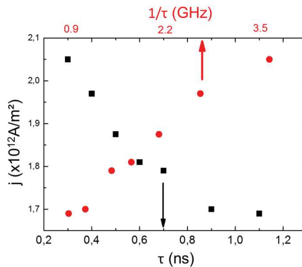
Figure III.11 – Simulation micromagnétique de la densité de courant critique de retournement de l'aimantation en fonction de l'inverse de la durée de l'impulsion de courant dans la piste de tantale en prenant en compte une température finie de 300 K. L'amortissement vaut 0,1.
