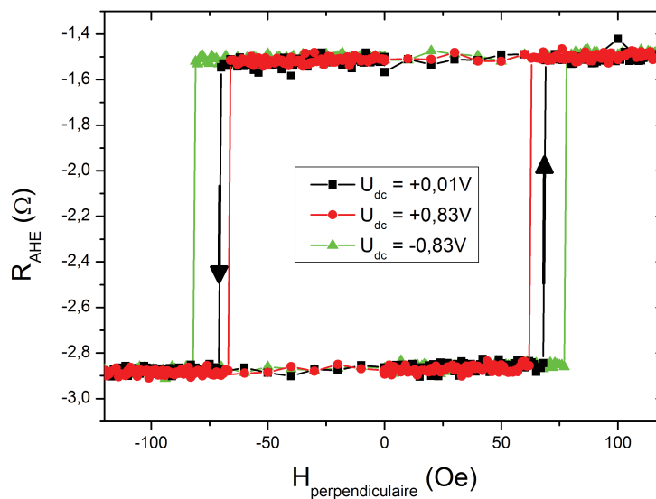
Figure IV.7 – Mesures de la résistance d'effet Hall anomal en fonction du champ magnétique appliqué perpendiculairement au plan des couches minces en présence d'une tension U_{\text{dc}} appliquée aux bornes de l'échantillon. Les différentes couleurs codent pour les différentes valeurs de tension U_{\text{dc}} et les flèches indiquent le sens dans lequel est parcouru le cycle en partant de H_{\text{perpendiculaire}} = 0 .
