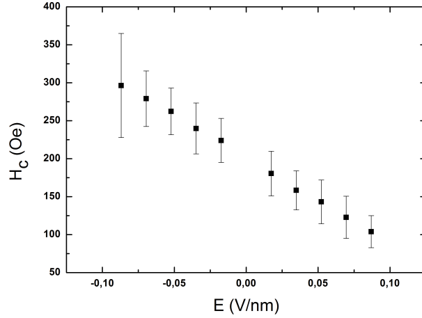
Figure IV.10 – Variations du champ coercitif en fonction du champ électrique pour une jonction tunnel magnétique. Les barres d’erreur représentent l’écart-type pour des mesures répétées 25 fois.
