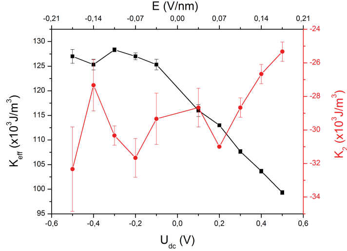
Figure IV.6 – Variations des constantes d’anisotropie magnétique K_{\text{eff}} et K_2 en fonction de la tension U_{\text{dc}} et du champ électrique E . Les barres d’erreur correspondent à l’écart-type pour les trois courbes calculées avec un décalage sur \theta_H de 0, +0,5 et -0,5^\circ . Les lignes reliant les points entre eux sont un guide pour les yeux.
