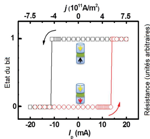
Figure I.9 – État du bit en fonction de l'intensité du courant d'écriture pour une piste de tantale de largeur 1,3 \mu\text{m} surmontée d'un plot magnétique de diamètre 1 \mu\text{m} . Le courant est injecté sous forme d'impulsions de 50 ns dans la piste de tantale de la cellule SOT-MRAM [25]. Les flèches rouge et noire représentent l'aimantation du matériau ferromagnétique adjacent au tantale et les flèches jaunes le CoFeB le plus éloigné de la piste de tantale.
