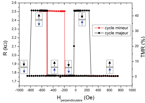
Figure II.10 – Courbes d’hystérésis mineure et majeure d’un empilement de 10 Ta/1 Co_{60}Fe_{20}B_{20}/MgO/1,5 Co_{20}Fe_{60}B_{20}/5 Ta/5 Ru correspondant respectivement au retournement de l’aimantation de la couche ferromagnétique douce (les carrés rouges) et aux retournements des aimantations des couches douces et dures (les points noirs). La flèche bleue du bas représente l’aimantation de la couche de CoFeB douce, la flèche noire du haut l’aimantation du CoFeB de référence.
