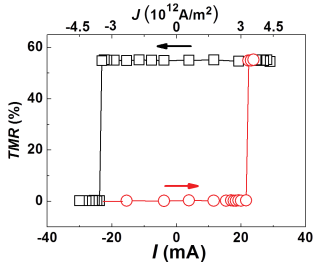
Figure III.5 – Magnétorésistance tunnel (TMR) en fonction du courant injecté dans la piste de tantale sous forme d'impulsions de durée 550 ps. Un champ magnétique extérieur de 1 kOe est appliqué pendant tout le cycle. Les carrés noirs correspondent à la diminution des amplitudes de courant et les ronds rouges à leur augmentation. Les flèches permettent de repérer dans quel sens est parcouru le cycle.
