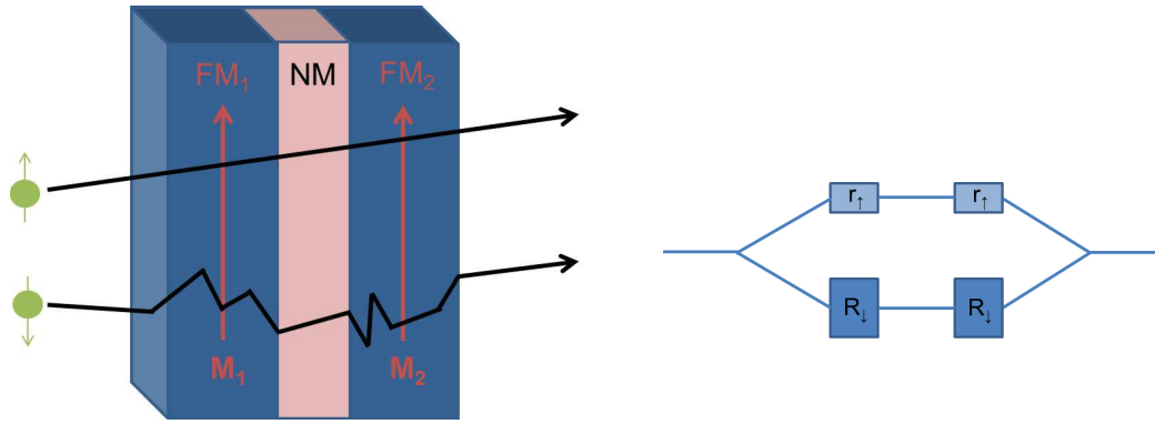
(a) Schéma du parcours des électrons dans la tricoche FM1/NM/FM2. Les cercles verts surmontés d'une flèche correspondent aux électrons avec leur spin et les courbes noires au chemin schématique des électrons. (b) Schéma électrique équivalent à la configuration magnétique parallèle.
