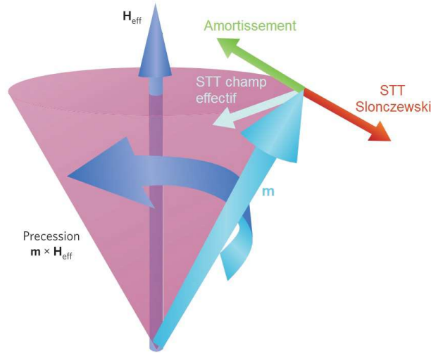
Figure I.19 – Schéma des couples s'exerçant sur l'aimantation normalisée \mathbf{m} décrits dans l'équation (I.18). On suppose que le courant de spin est positif : \mathbf{I}_s > 0 . Si le courant est de sens opposé les couples auront un sens opposé à celui présenté. \mathbf{H}_{eff} est le champ magnétique effectif [44].
