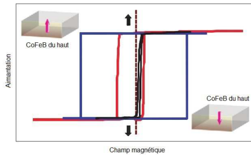
Figure I.40 – Courbes d’hystérésis schématisques expliquant le principe du dispositif logique étudié par Wang et al. Les cycles sont effectués avec un champ magnétique extérieur H_{\text{ext}} = 55 \text{ Oe} représenté schématiquement par la ligne en pointillés. La courbe bleue de champ coercitif le plus large correspond à U_{\text{MTJ}} \approx 0 \text{ V} , la rouge (champ coercitif intermédiaire) à U_{\text{MTJ}} = -0,9 \text{ V} et la noire (champ coercitif proche de 0) à U_{\text{MTJ}} = -1,5 \text{ V} [112].
