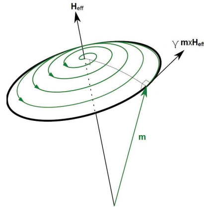
Figure I.18 – Illustration de la précession d'un moment magnétique normalisé \mathbf{m} autour d'un champ magnétique effectif \mathbf{H}_{eff} . La trajectoire en noir correspond au terme de précession seul alors que la trajectoire en vert qui s'enroule autour de \mathbf{H}_{eff} comprend le terme d'amortissement [28].
