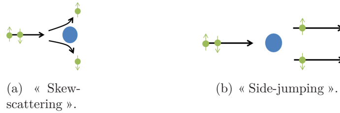
Figure I.24 – Représentation schématique des mécanismes extrinsèques d'effet Hall de spin avec les électrons de conduction en vert surmontés d'une flèche verte (leur spin) arrivant sur une impureté (disque bleu).
