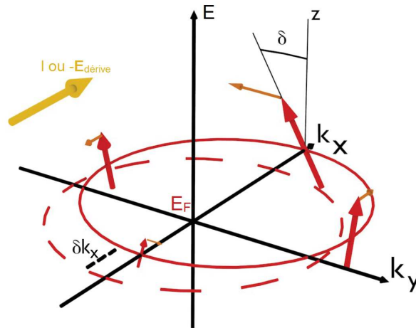
Figure I.22 – Schéma de l'effet du couple Rashba de champ effectif \Gamma_{\mathbf{R},\mathbf{t}} sur les spins des électrons majoritaires (flèches rouges) du niveau de Fermi E_F (cercle rouge). Les flèches de couleur orange (contenues dans un plan parallèle à (0, \mathbf{k}_x, \mathbf{k}_y) ) indiquent le champ magnétique Rashba ressenti par les spins des électrons. L'intégration de tous ces champs sur la surface de Fermi donne maintenant un résultat non nul [76].
