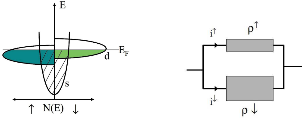
(a) Densités d'états n(E) schématiques des bandes énergétiques des électrons d de spins \uparrow (en bleu, majoritaires) et \downarrow (en vert, minoritaires) et des bandes s .
