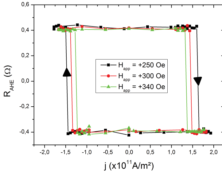
Figure III.2 – Mesures de la résistance d'effet Hall anomal R_{\text{AHE}} en fonction de la densité de courant j injectée dans la piste de tantale. Les impulsions de courant durent 20 ns. Les couleurs codent pour les différentes valeurs de champ magnétique extérieur H_{\text{app}} , les flèches indiquent le sens de parcours du cycle en partant de j = 0 .
