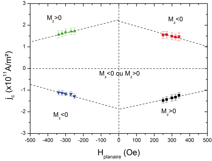
Figure III.3 – Diagramme d'état de l'aimantation d'un plot circulaire de CoFeB/MgO sur une piste de tantale lithographiée sous forme de croix de Hall. Les symboles pleins sont les points de mesures correspondant au retournement de l'aimantation. Les pointillés sont des extrapolations qui délimitent les zones de stabilité de l'aimantation et les barres d'incertitudes correspondent à l'écart-type sur les 25 mesures.
