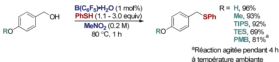
Schéma 1. Catalyse par B(C 6 F 5 ) 3 ·H 2 O dans le nitrométhane permettant la substitution chimiosélective d'une large gamme d'alcools \pi -activés.
