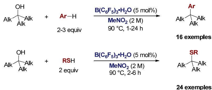
Schéma 2. Catalyse par \text{B(C}_6\text{F}_5)_3 \cdot \text{H}_2\text{O} dans le nitrométhane permettant l'utilisation substœchiométrique dans la substitution d'alcools tertiaires aliphatiques.
