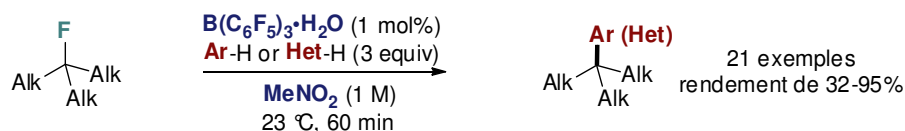
Schéma 4. Arylation de composés aliphatiques fluorés par la réaction de Friedel-Crafts permise par B(C_6F_5)_3 \cdot H_2O dans le nitrométhane.
