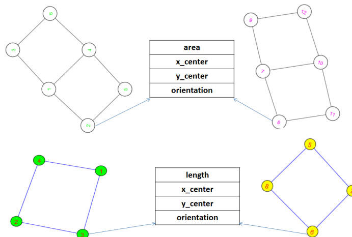
Figure 4.17 – Graphes attribués pour les deux ensembles de primitives de la figure 4.14. Première ligne : graphe correspondant à l'ensemble d'ellipses extraites de l'image de référence (gauche) ; graphe correspondant à l'ensemble d'ellipses extraites de l'image de l'objet à évaluer (droite). Deuxième ligne : graphe correspondant à l'ensemble des segments de droite extraits de l'image de référence (gauche) ; graphe correspondant à l'ensemble des segments de droite de l'image test (droite).
