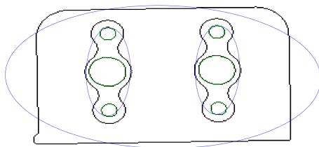
Figure 4.11 – Extraction d'ellipses par la méthode de Prasad : les ellipses considérées correctes sont dessinées en vert et les candidates non retenues sont dessinées en bleu. Le contour est affiché en noir sur fond blanc pour plus de clarté
