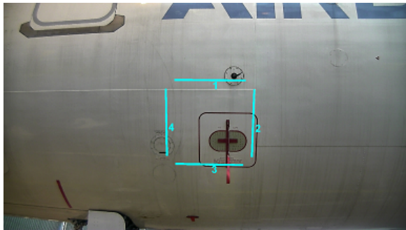
(a) Projection des primitives CAO (segments de droite) sur l'image acquise avec la caméra PTZ.
